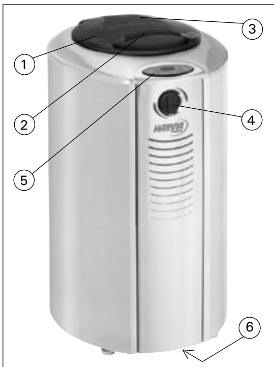
Figure 1. Heater parts Abbildung 1. Teile des Saunaofens
