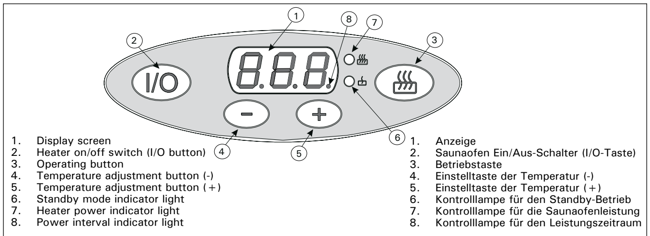
Figure 2. Heater control units Abbildung 2. Steuerelemente des Saunaofens
