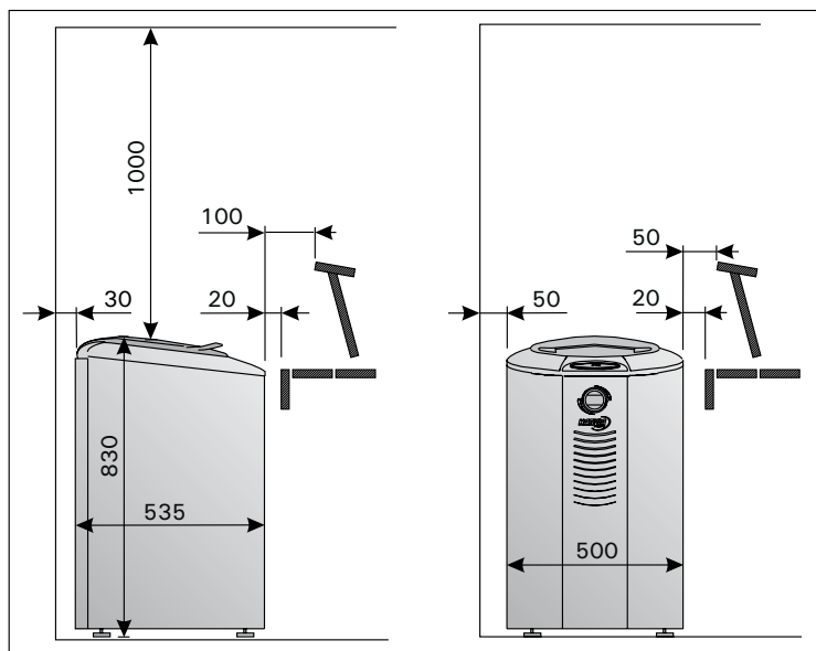
Figure 7. Minimum safety distances from the heater (mm) Abbildung 7. Minimum Sicherheitsmindestabstände des Saunaofens (mm)
