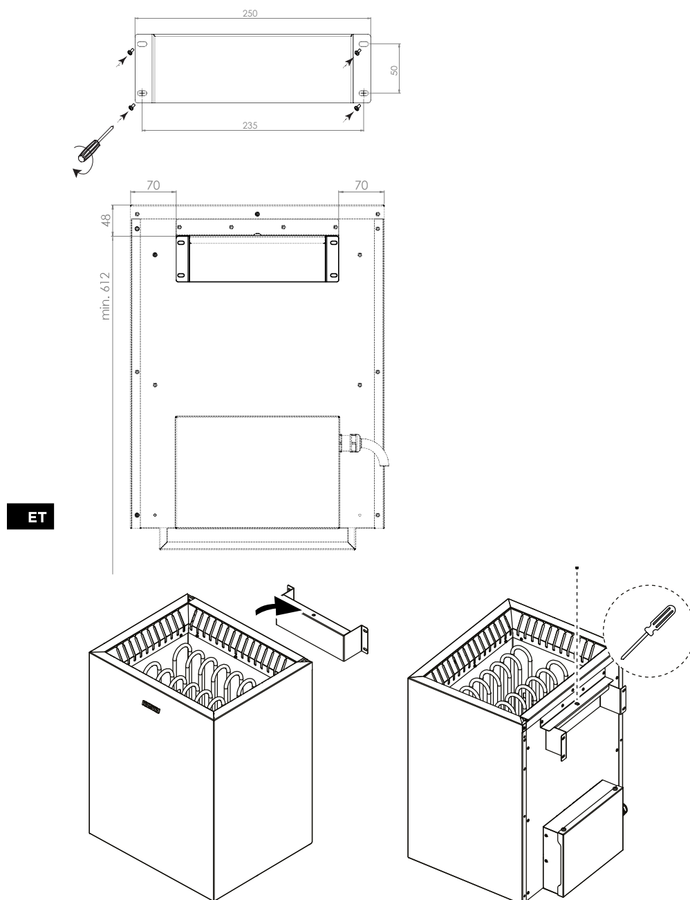
Joonis 2. Kerise paigaldamine
