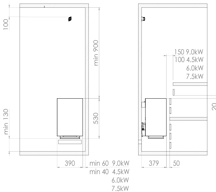
Figura 1. Distancias de seguridad
