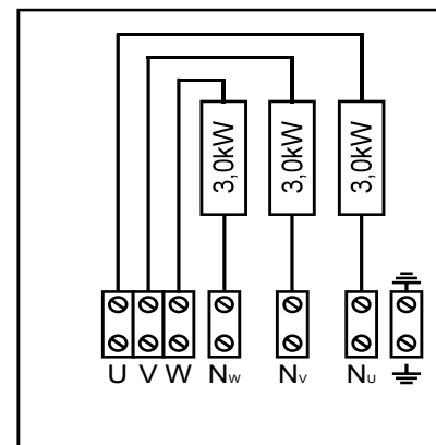
Abbildung 8. Verdrahtungsschema HLW90E
