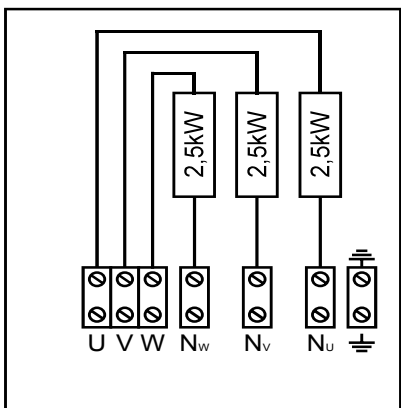
Abbildung 7. Verdrahtungsschema HLW75E
