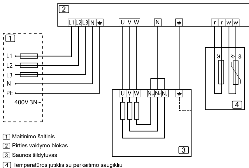
9 pav. Laidų prijungimo schema 400V 3N~
