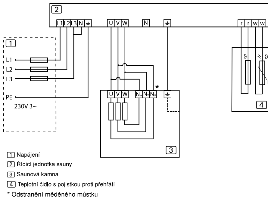
Obrázek 11. Schéma zapojení 230V 3~
