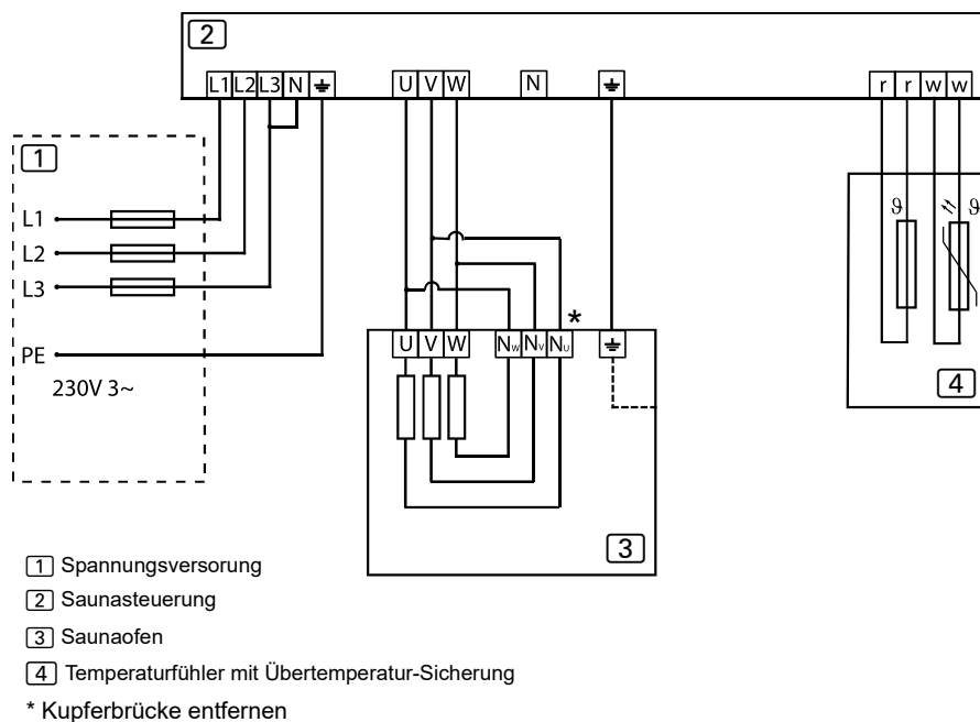
Abbildung 11. Anschlussplan 230V 3~
