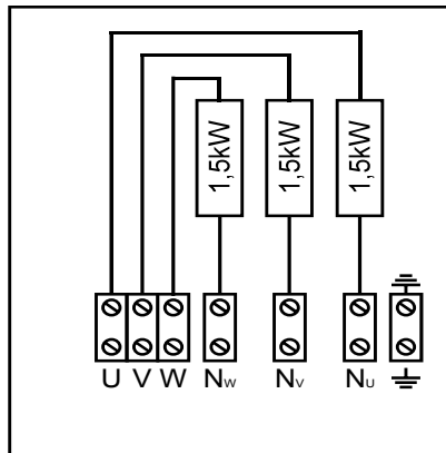
Abbildung 5. Verdrahtungsschema HLW45E
