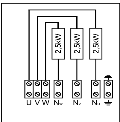
Figure 7. Schéma de câblage HLW75E
