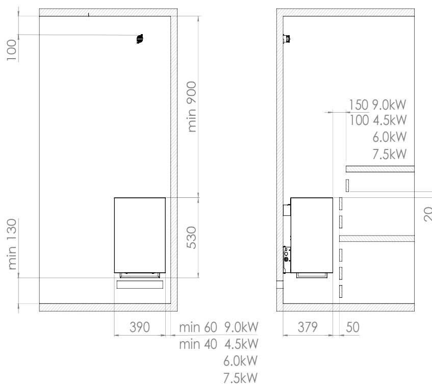
Bild 1. Säkerhetsavstånd
