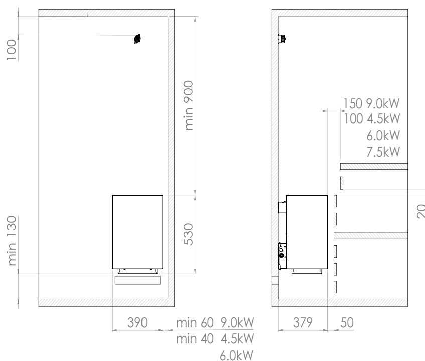
Joonis 1. Ohutuskaugused
