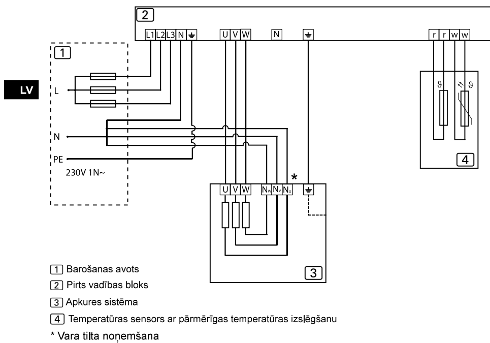
10. attēls. Savienojuma shēma 230V 1N~
