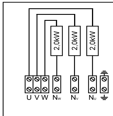
Figuur 6. Aansluitschema HLW60E
