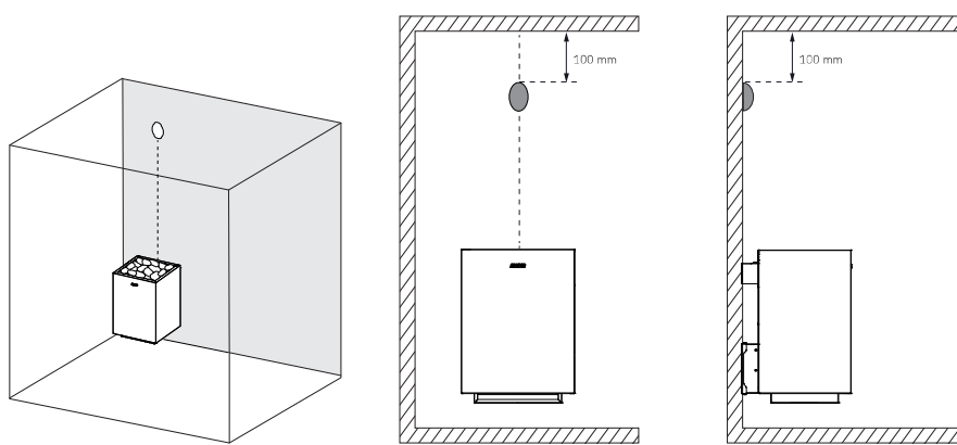
Figure 3. Installation du capteur de chaleur au mur
