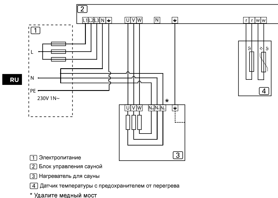
Рисунок 10. Электрическая схема 230V 1N~
