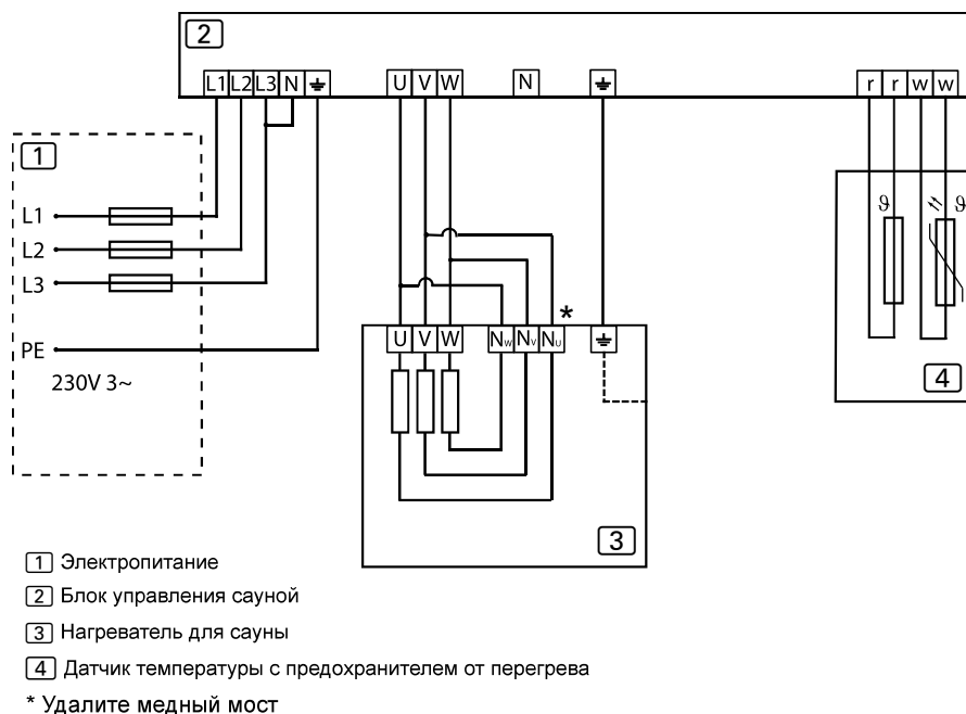
Рисунок 11. Электрическая схема 230V 3~
