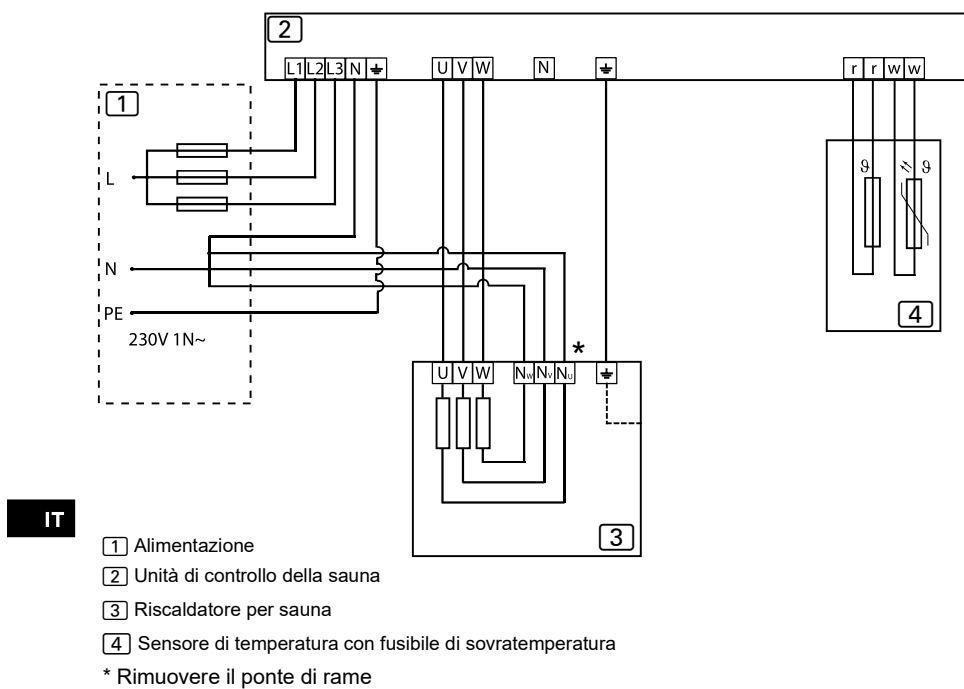
Figura 10. Schema elettrico 230V 1N~
