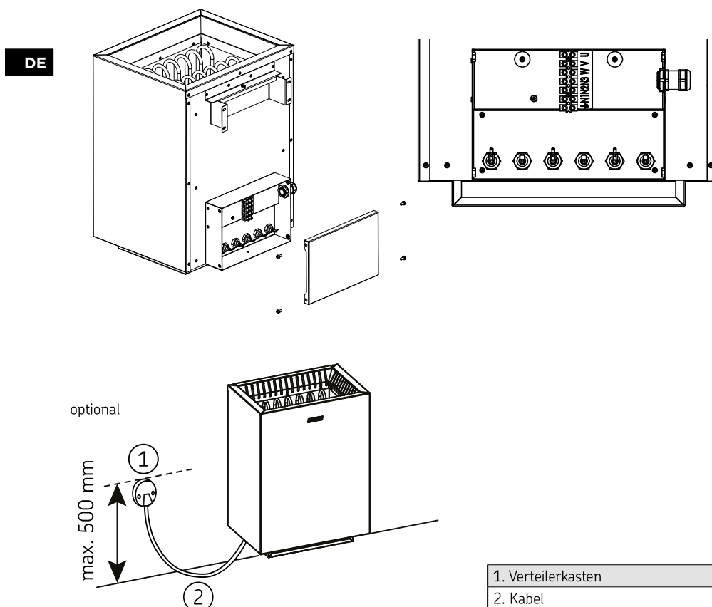
Abbildung 4. Elektroanschlüsse
