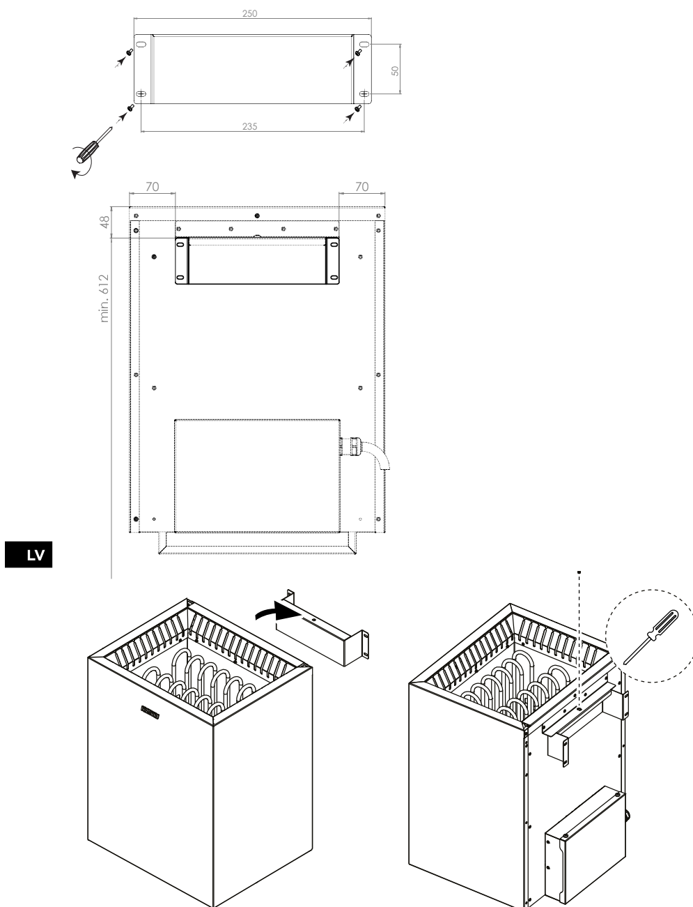
2. attēls. Pirts sildītāja uzstādīšana
