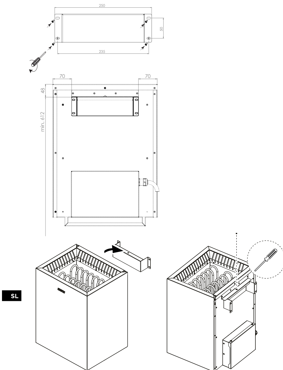
Slika 2. Namestitev grelca za savno
