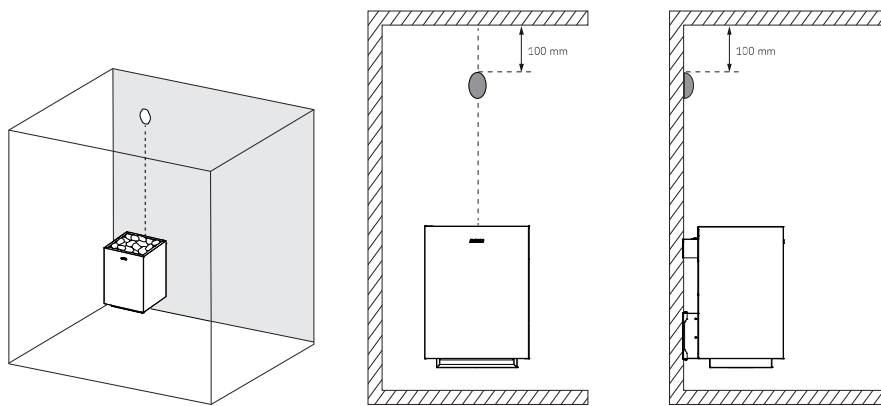
Abbildung 3. Montage des Ofenfühlers an der Wand
