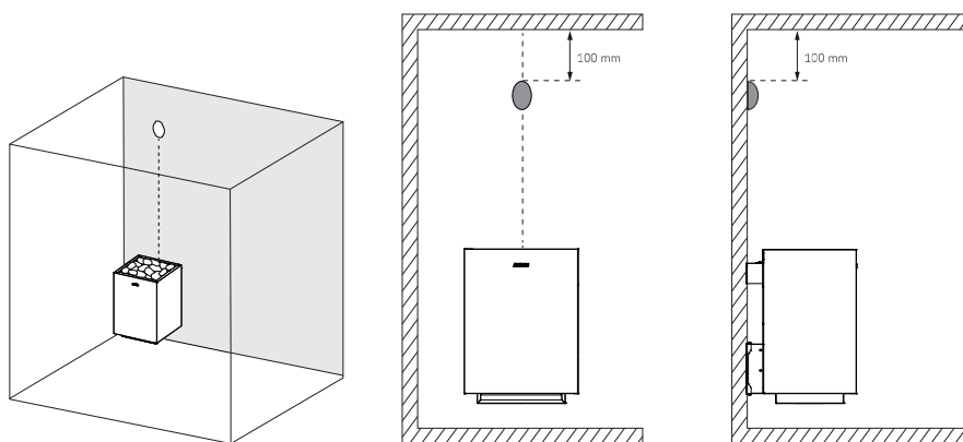
Bild 3. Installera värmegivaren på väggen
