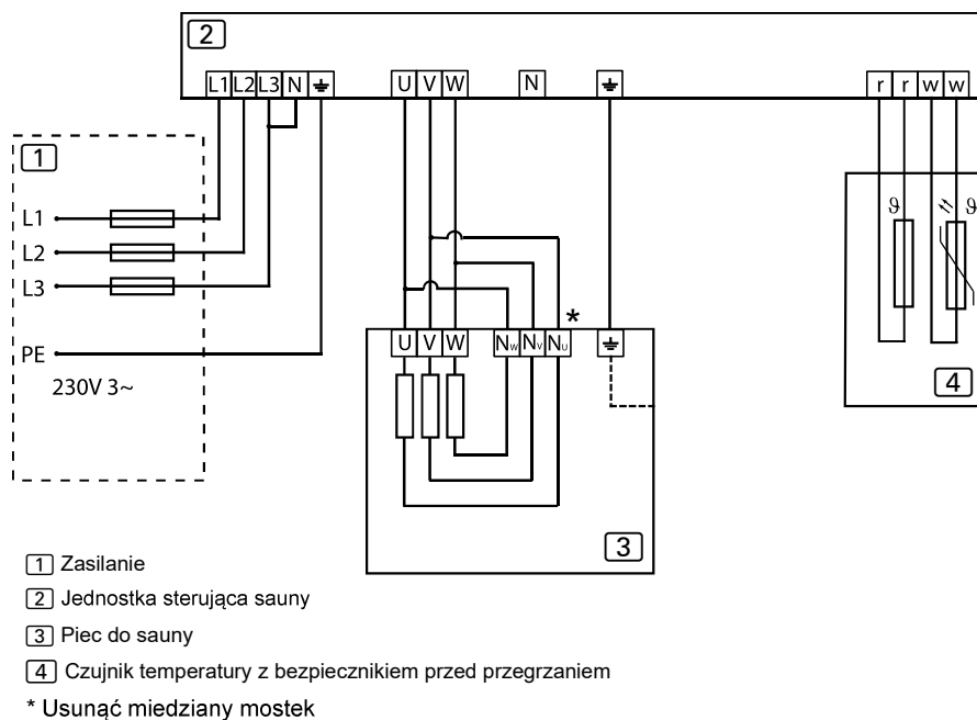
Rysunek 11. Schemat połączeń 230V 3~
