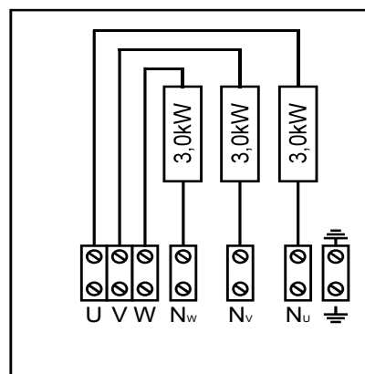
Kuva 8. Kytentäkaavio HLW90E
