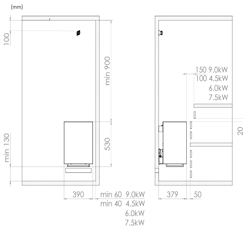
Figuur 1. Veiligheidsafstanden
