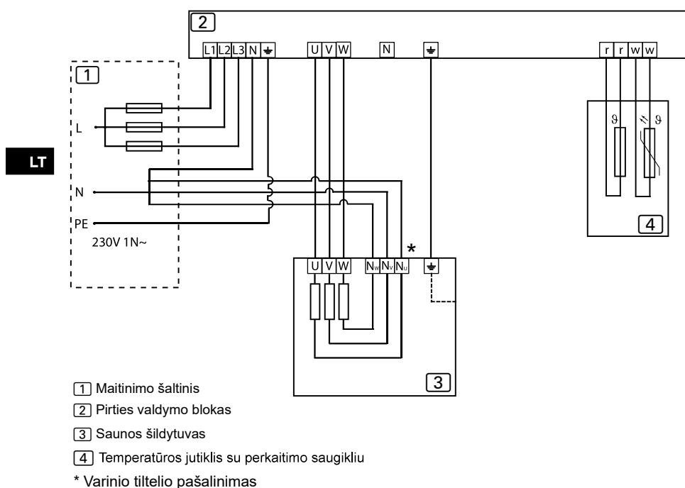
10 pav. Laidų prijungimo schema 230V 1N~
