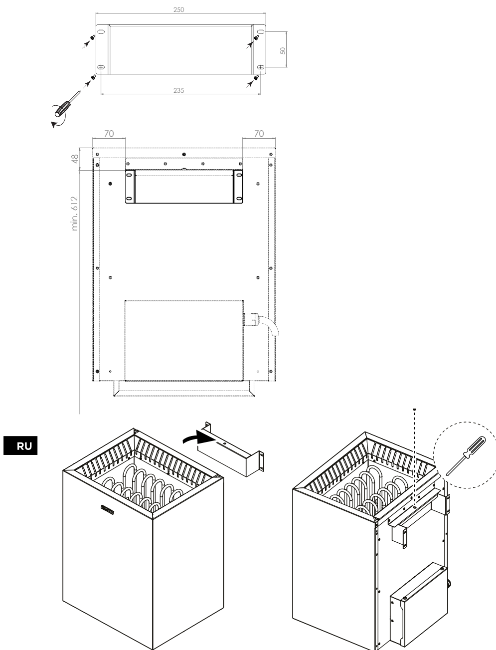
Рисунок 2. Установка каменки
