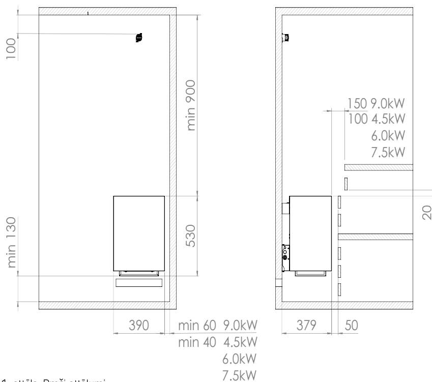
1. attēls. Droši attālumi
