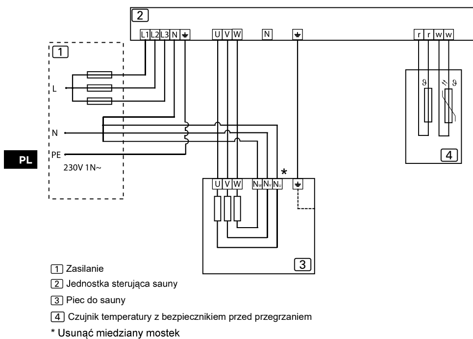
Rysunek 10. Schemat połączeń 230V 1N~
