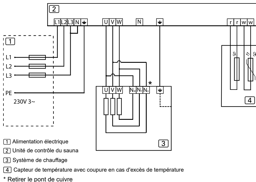
Figure 11. Schéma de câblage 230V 3~
