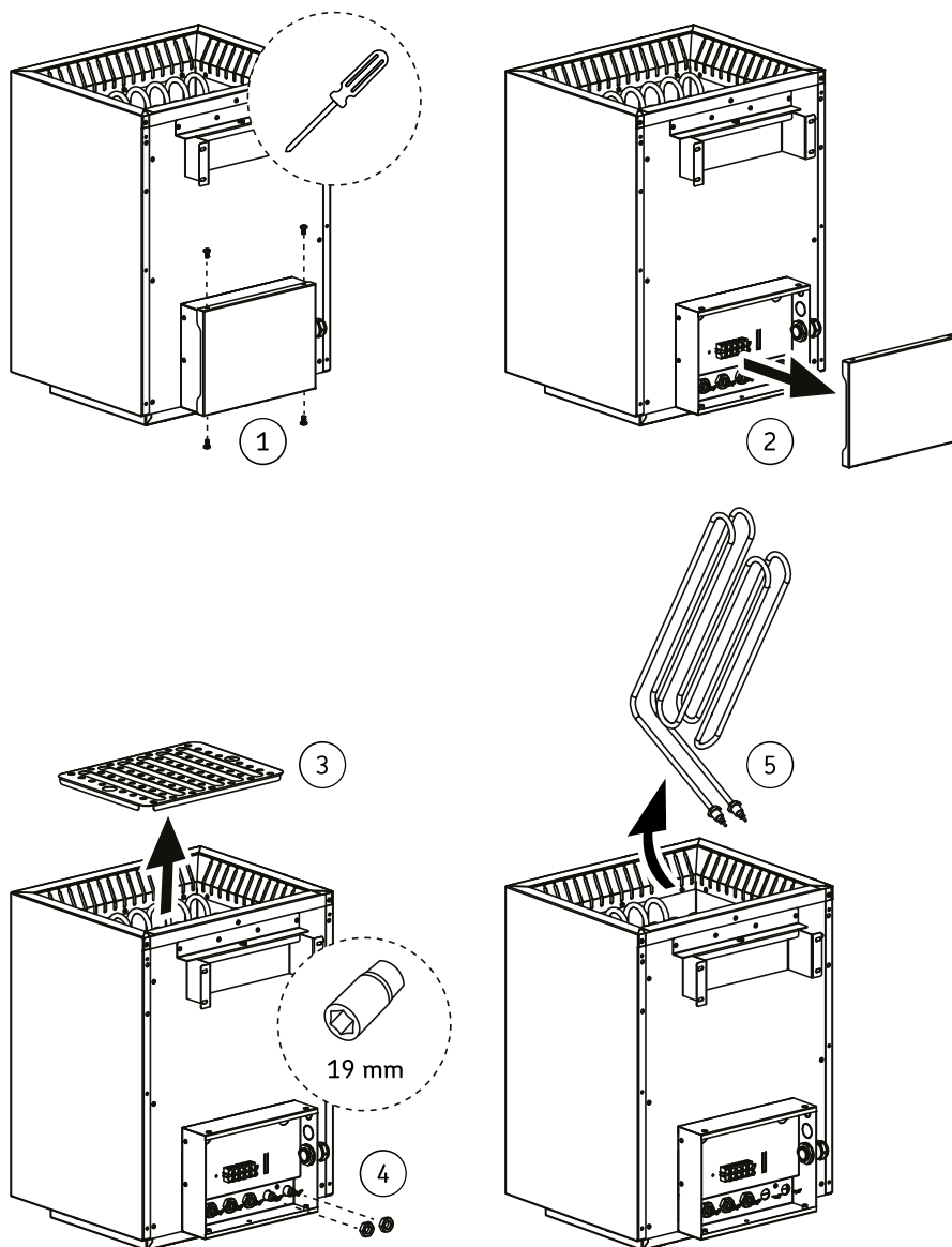
Kuva 14. Vastusten vaihtaminen
