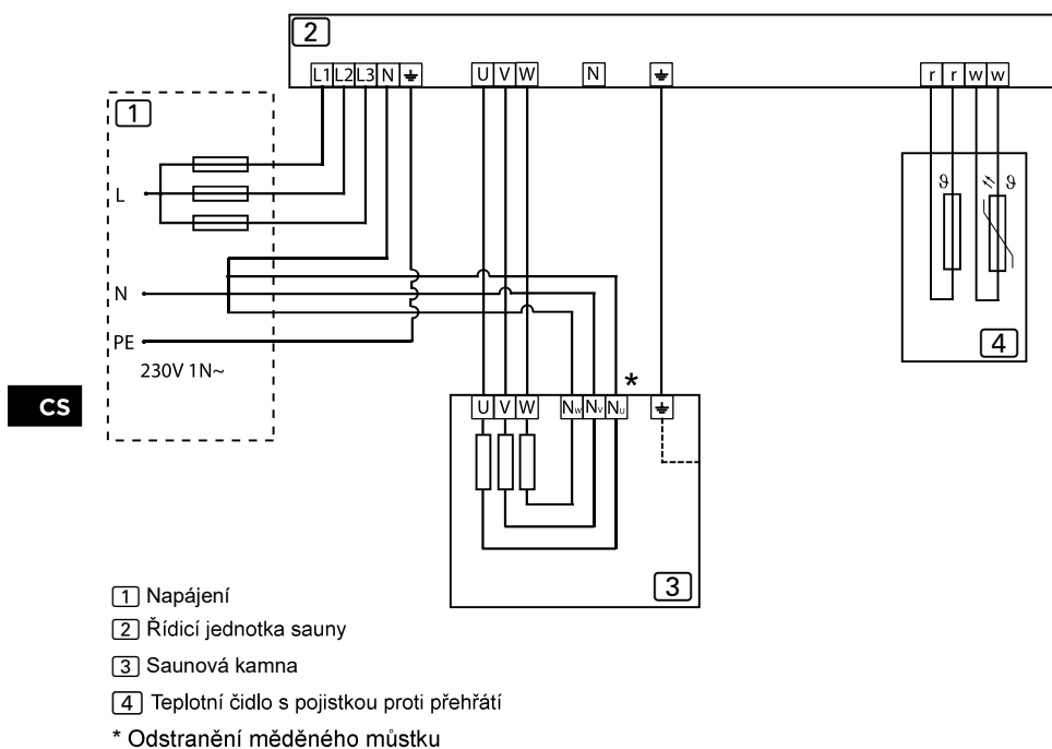
Obrázek 10. Schéma zapojení 230V 1N~
