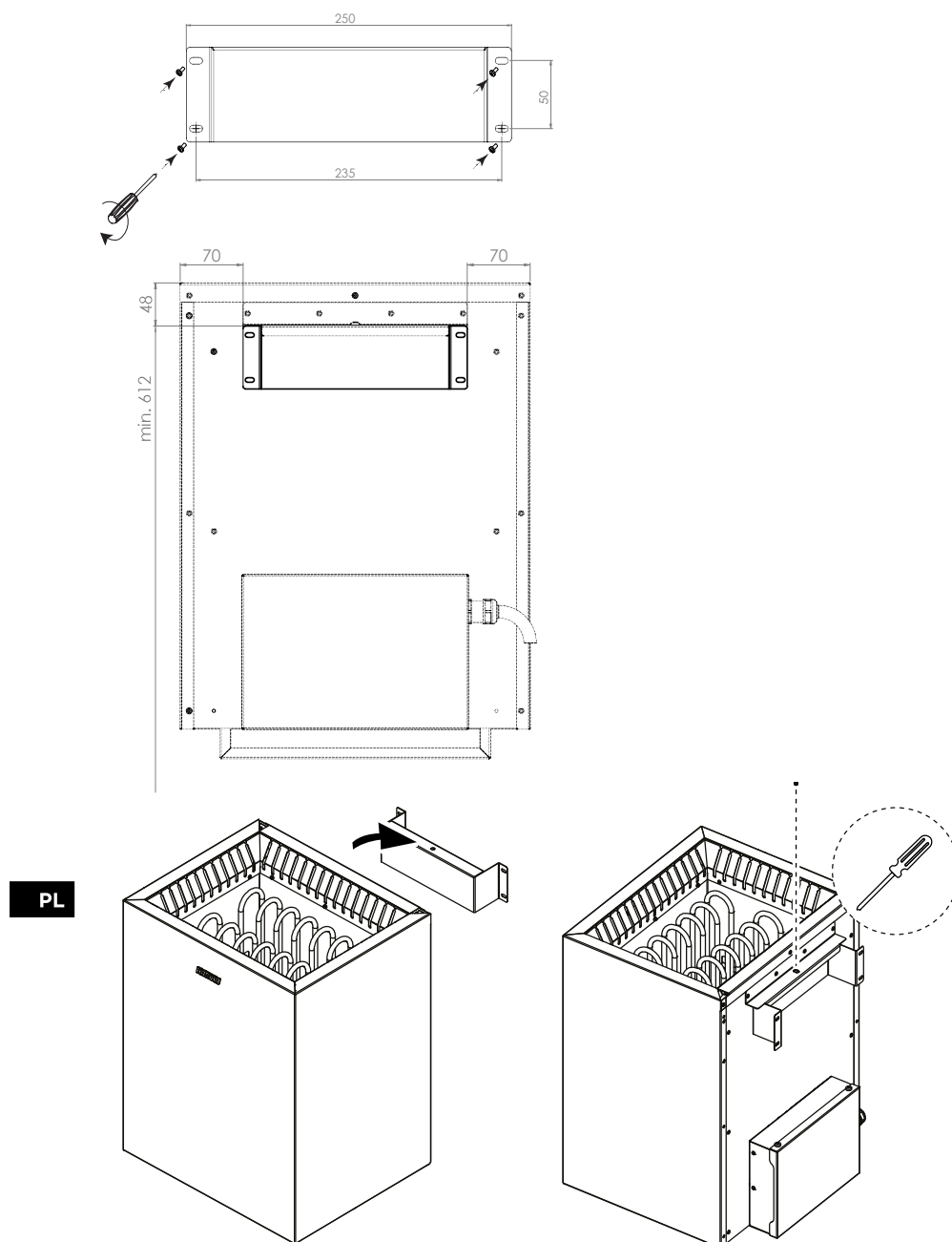
Rysunek 2. Montaż pieca do sauny
