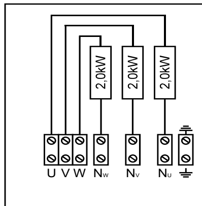
Kuva 6. Kytentäkaavio HLW60E
