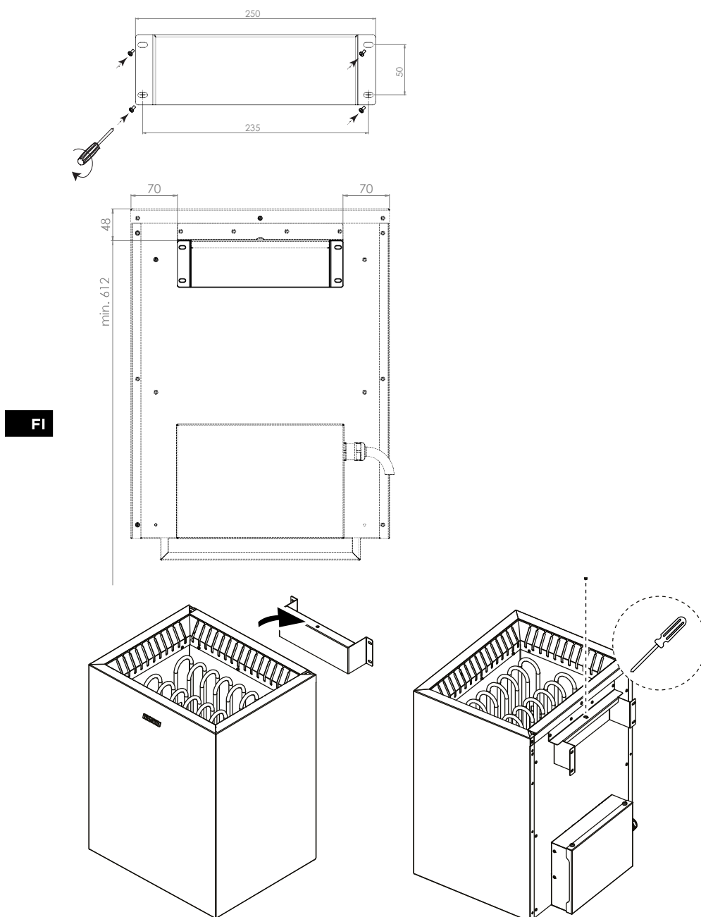
Kuva 2. Kiukaan asennus
