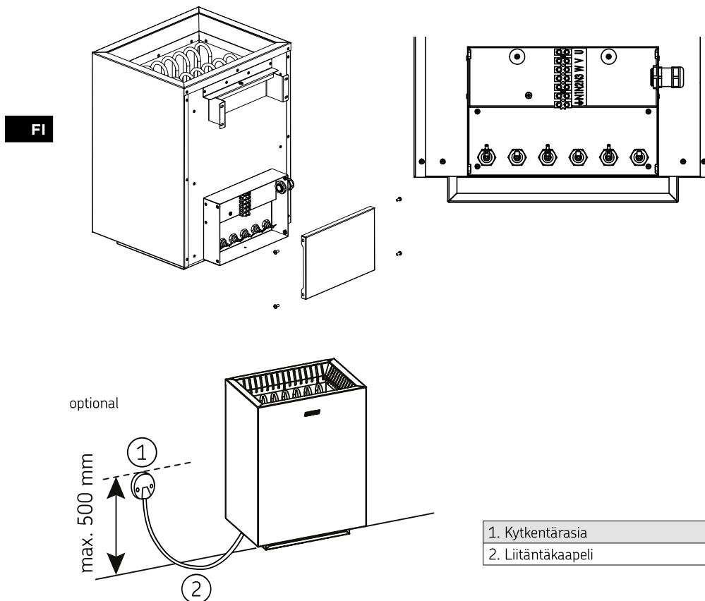
Kuva 4. Sähkökytkennät
