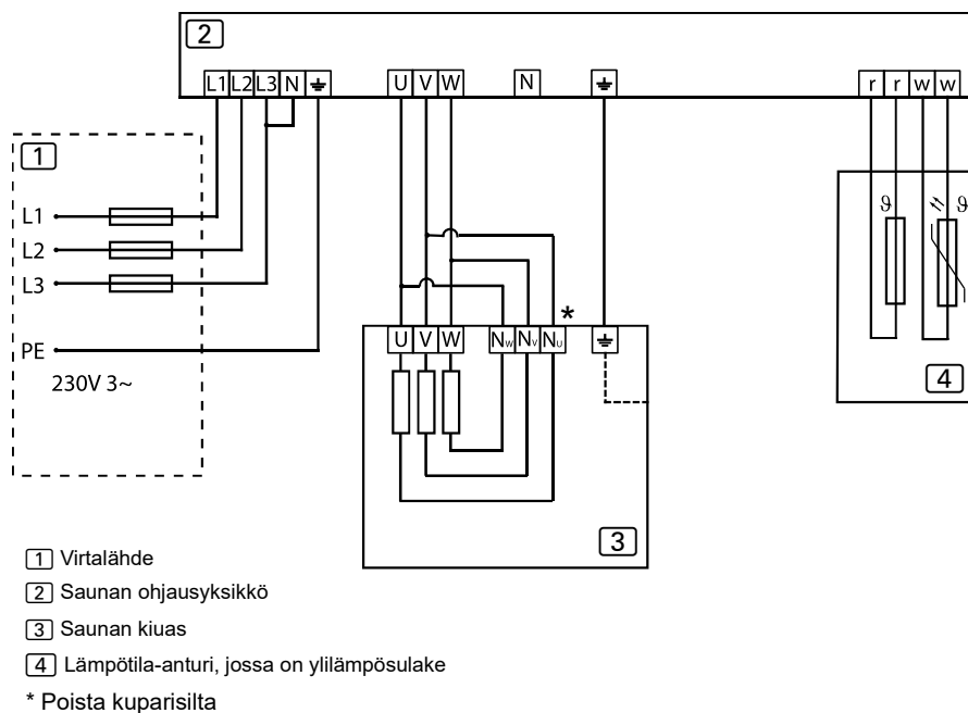
Kuva 11. Kytentäkaavio 230V 3~
