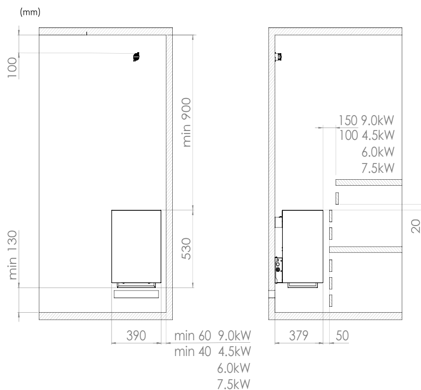
Рисунок 1. Безопасное расстояние
