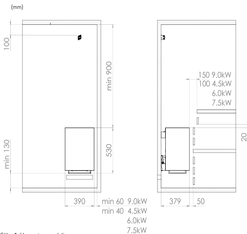
Slika 1. Varnostne razdalje
