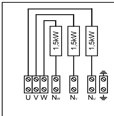
Kuva 5. Kytentäkaavio HLW45E
