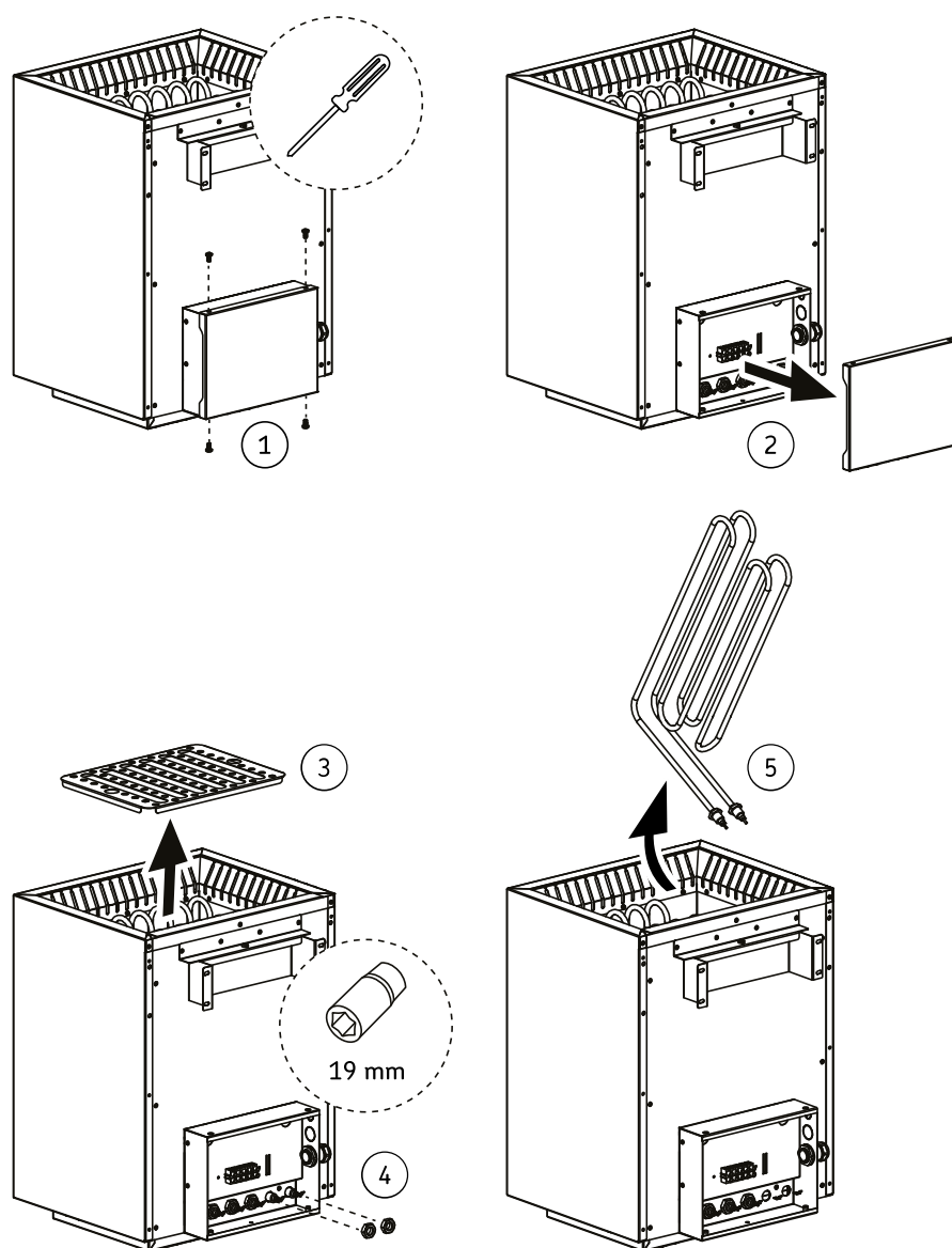
Figuur 14. Verwarmingselementen vervangen
