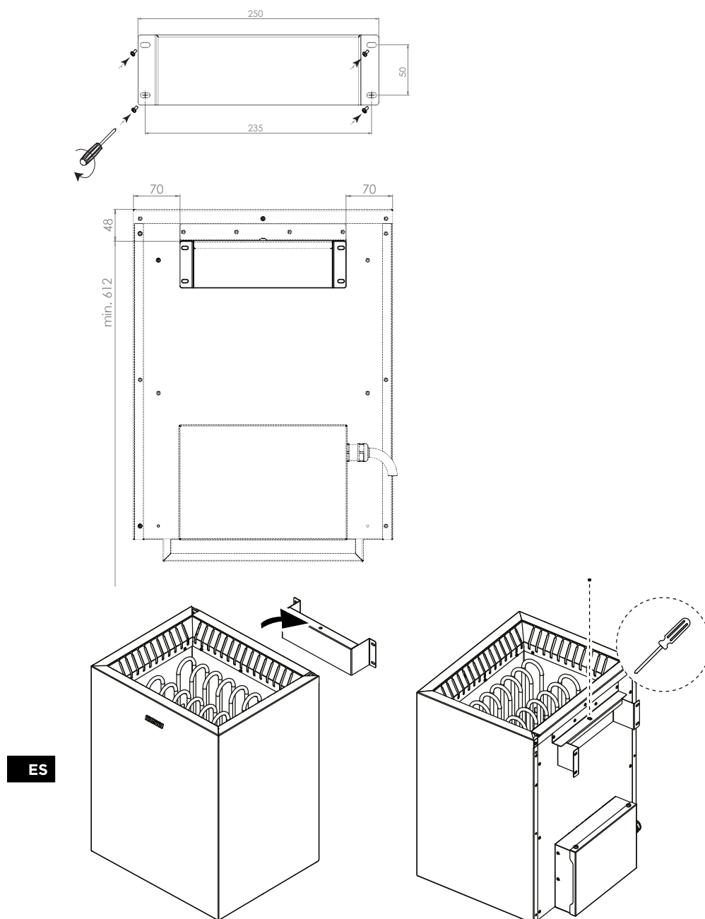
Figura 2. Instalación del calentador para sauna
