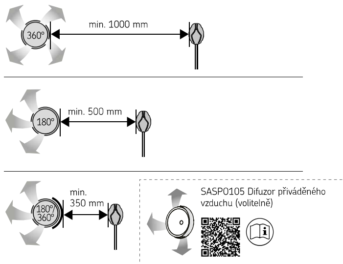
Obrázek 13. Minimální vzdálenost od větracího otvoru přívodu vzduchu k teplotnímu senzoru
