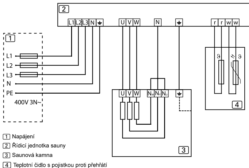
Obrázek 9. Schéma zapojení 400V 3N~
