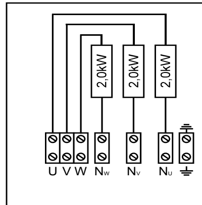
Abbildung 6. Verdrahtungsschema HLW60E
