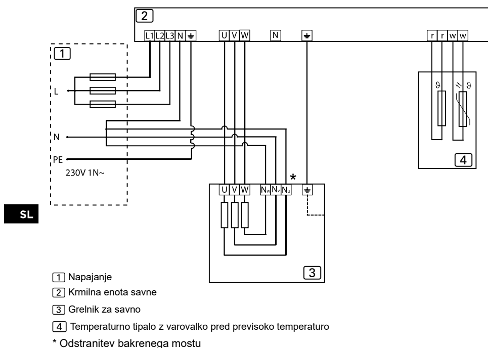
Slika 10. Shema ožičenja 230V 1N~
