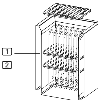
Figure 12. Placement des pierres de poêle
