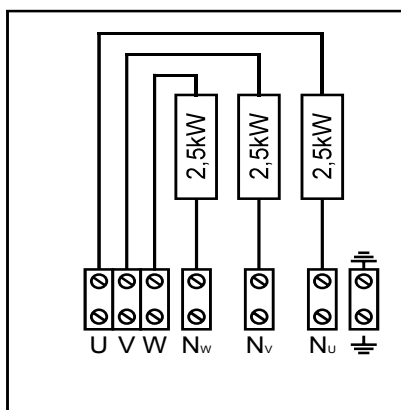
Рисунок 7. Электрическая схема HLW75E
