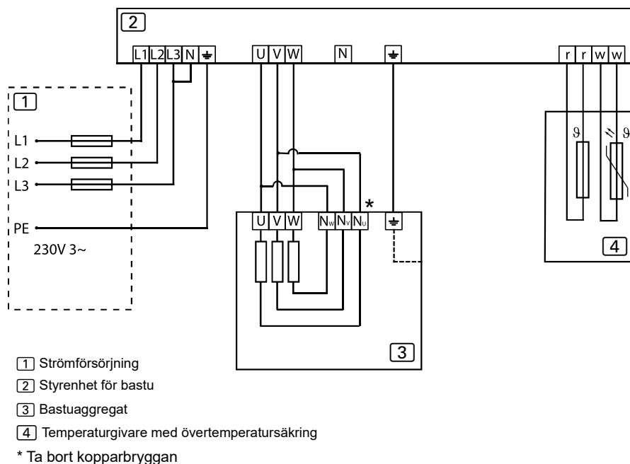
Bild 11. Kopplingsschema 230V 3~
