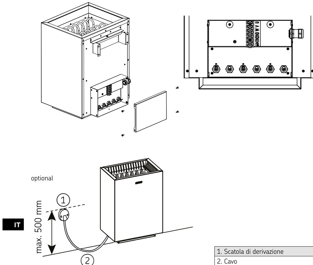
Figura 4. Collegamenti elettrici
