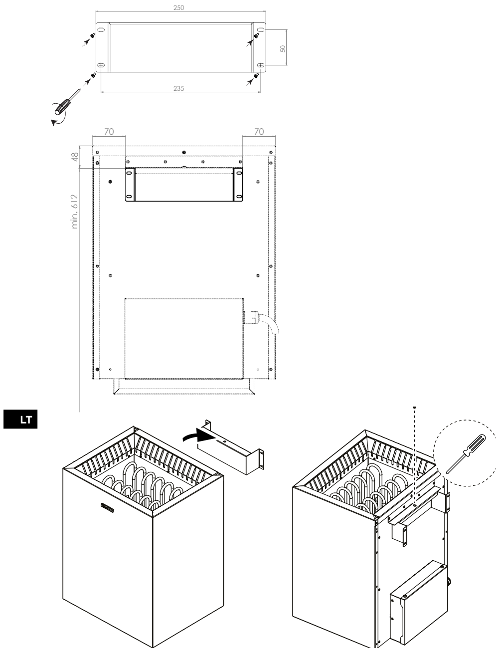
2 pav. Saunos krosnelės įrengimas
