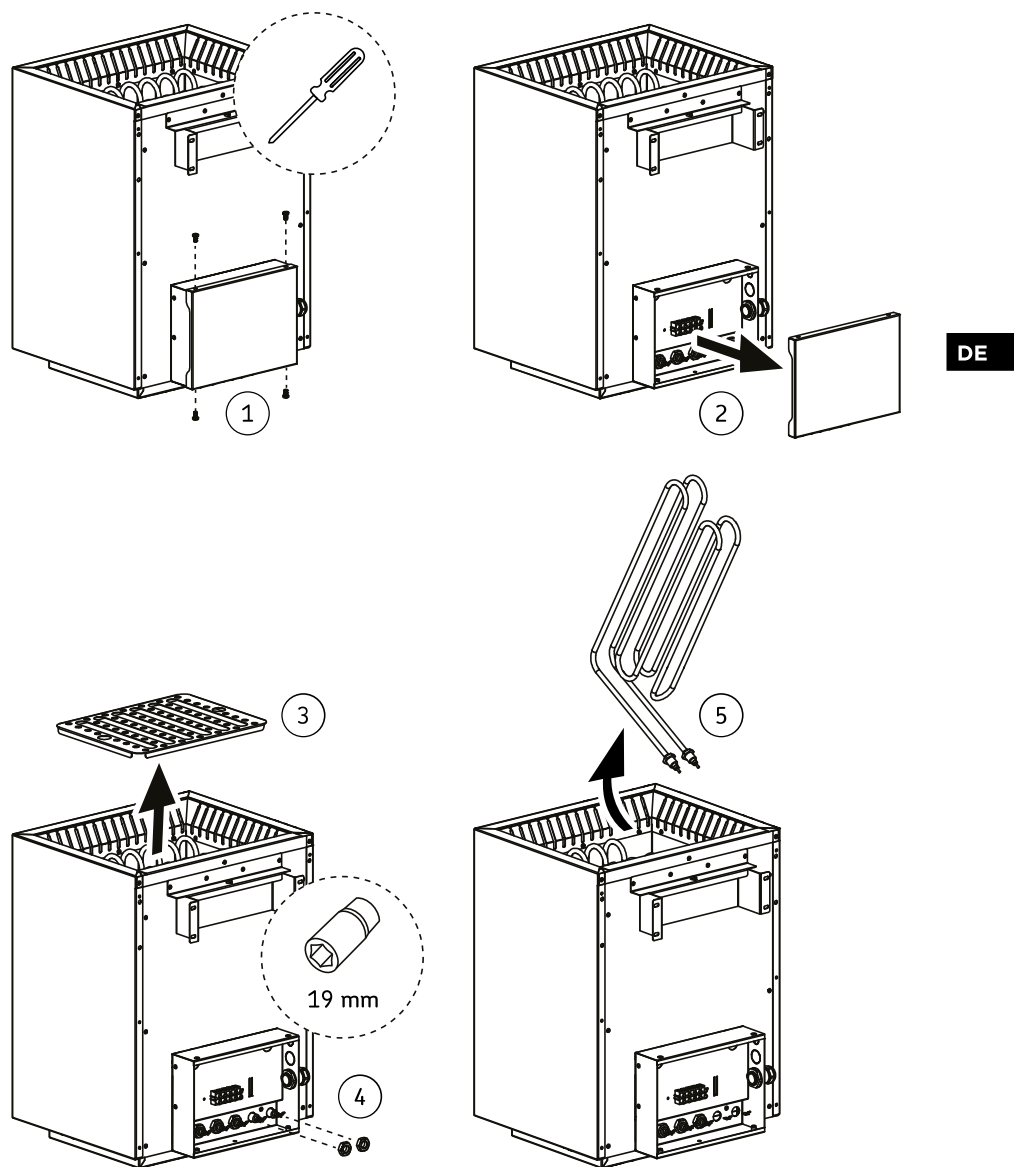
Abbildung 14. Auswechseln der Heizelemente
