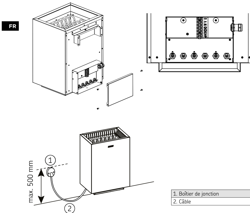
Figure 4. Raccordements électriques
