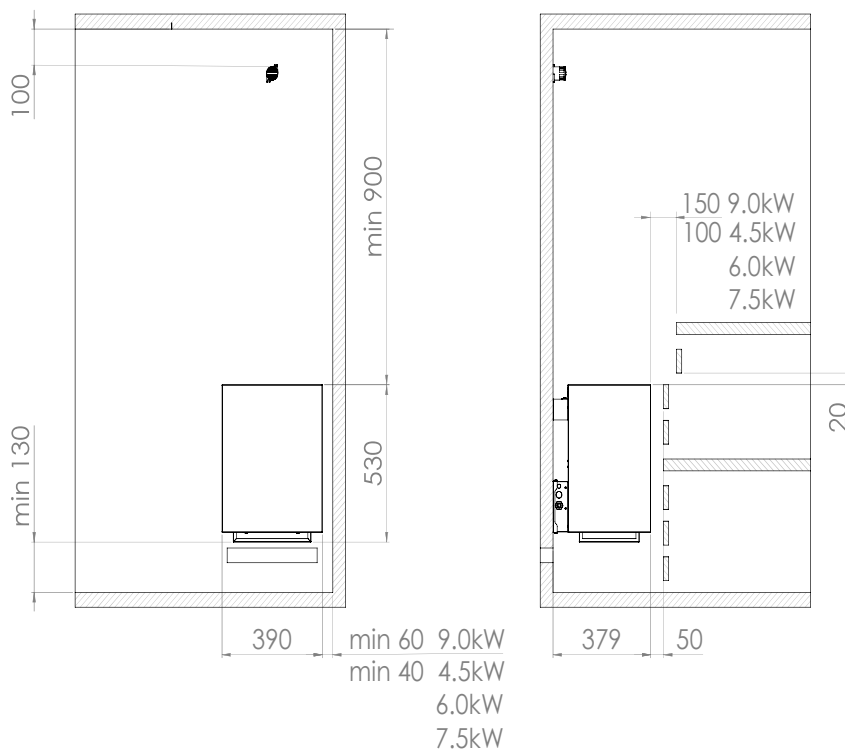
1 pav. Apsauginis atstumas
