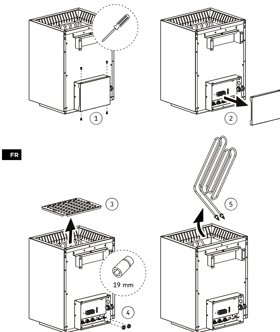
Figure 14. Remplacement des résistances
