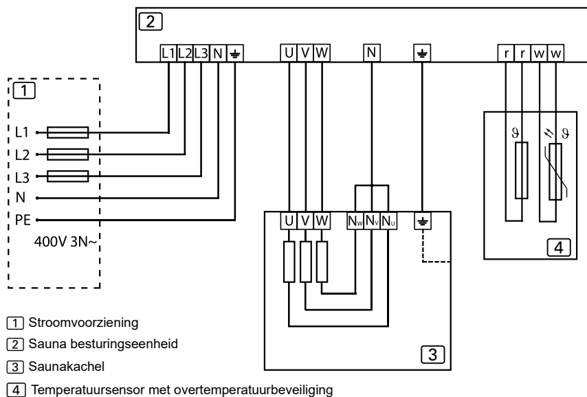
NL Figuur 9. Aansluitschema 400V 3N~
