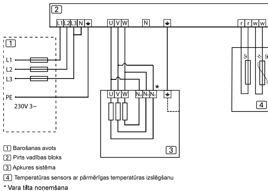
11. attēls. Savienojuma shēma 230V 3~
