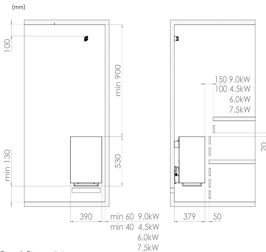
Figura 1. Distanza di sicurezza
