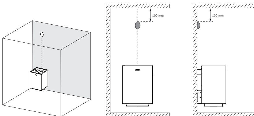
Obrázek 3. Instalace tepelného senzoru na stěnu
