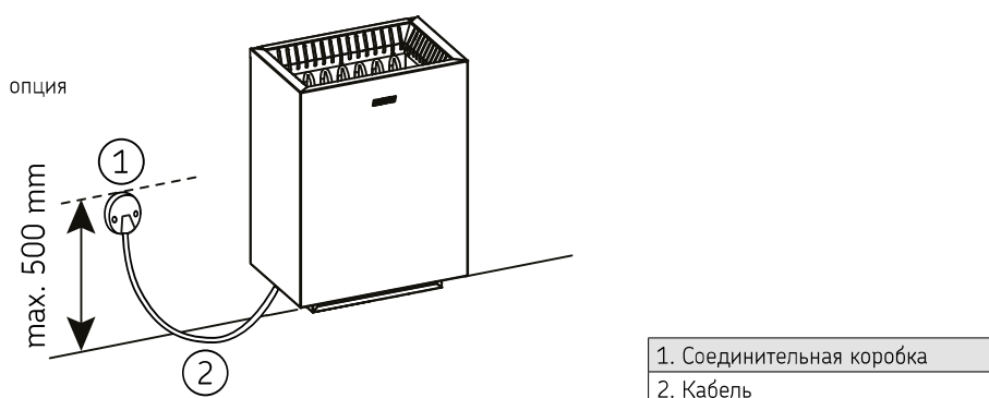
Рисунок 4. Электрические соединения
