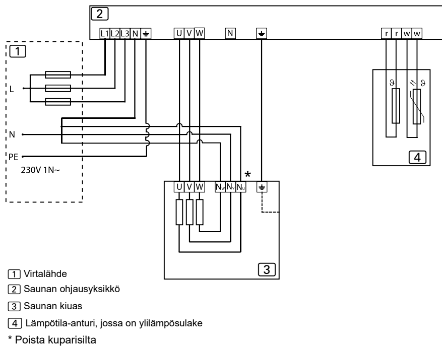
Kuva 10. KytKentäkaavio 230V 1N~
