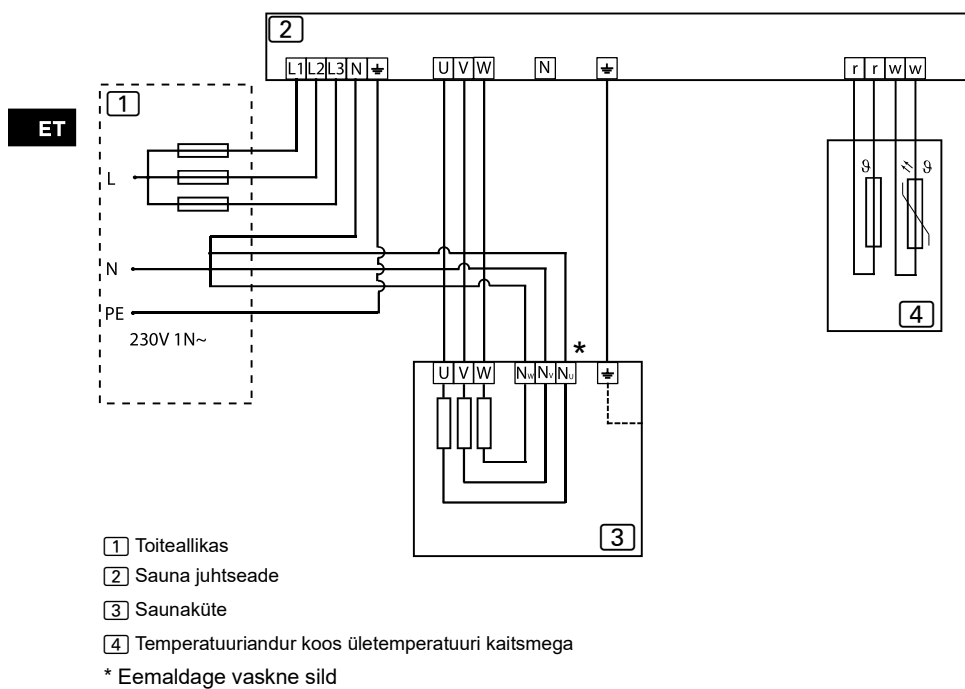
Joonis 10. Elektriskeem 230V 1N~
