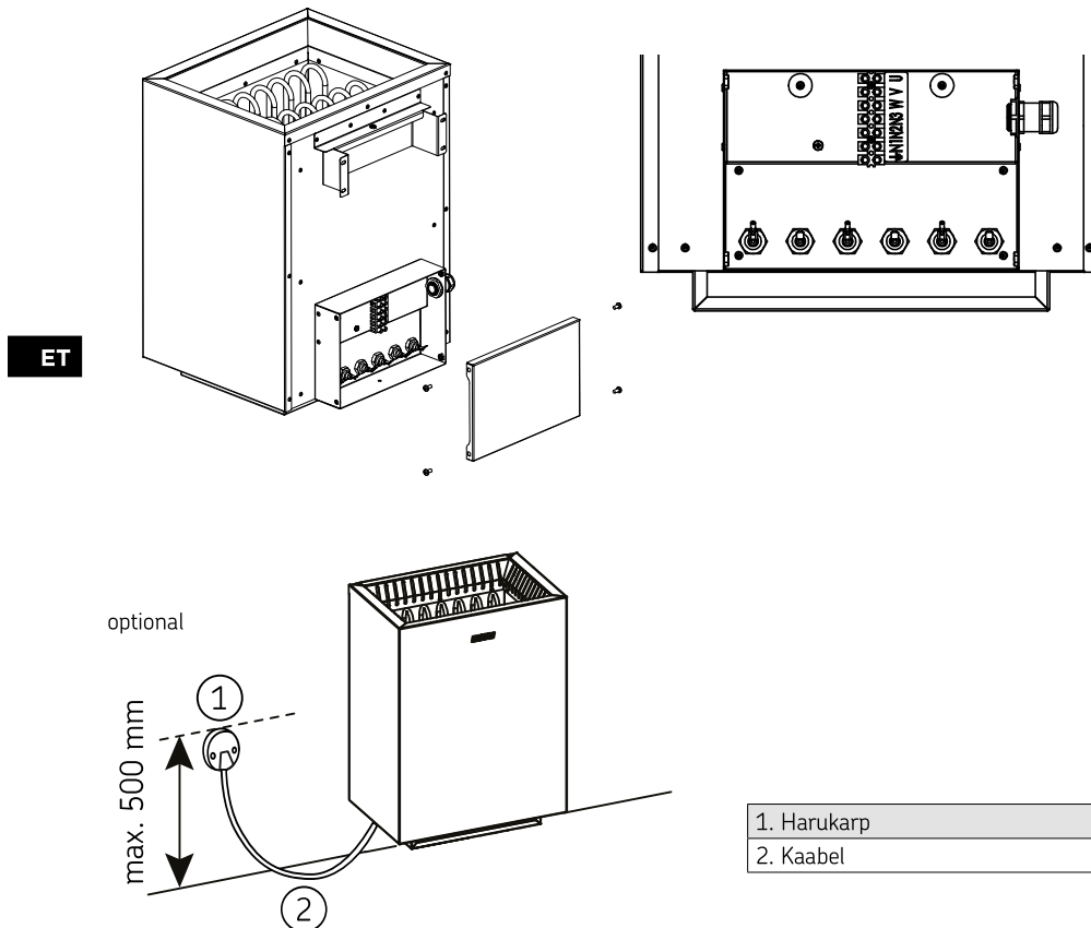
Joonis 4. Elektriühendused
