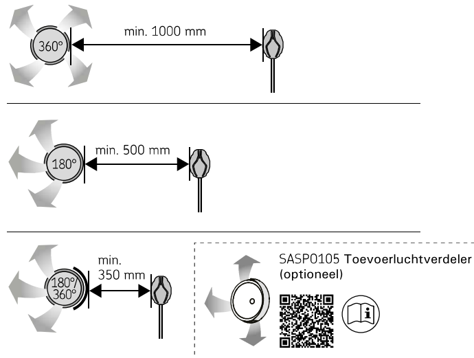
Figuur 13. Minimale afstand van de luchttoevoerlepel tot de temperatuursensor.
