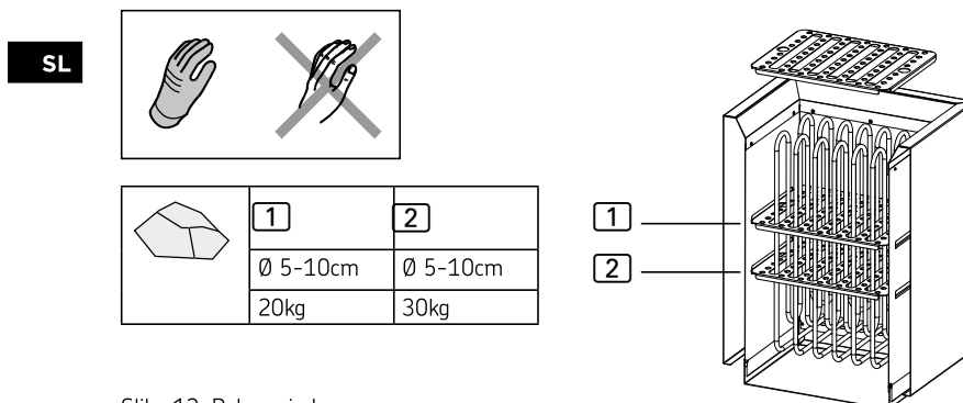
Slika 12. Polaganje kamnov za savno
