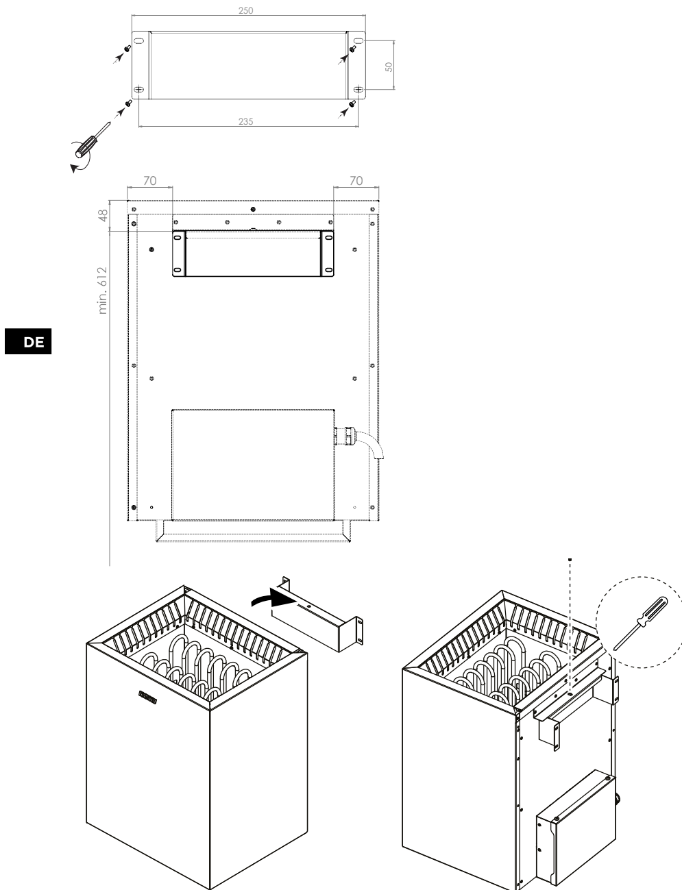
Abbildung 2. Installation eines Saunaofens
