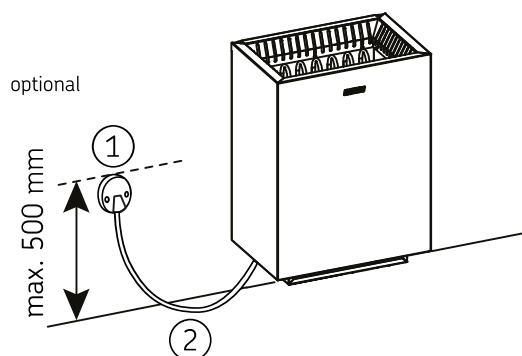
4. attēls. Elektroapgādes pieslēgumi
