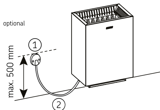
4 pav. Elektros jungtys
