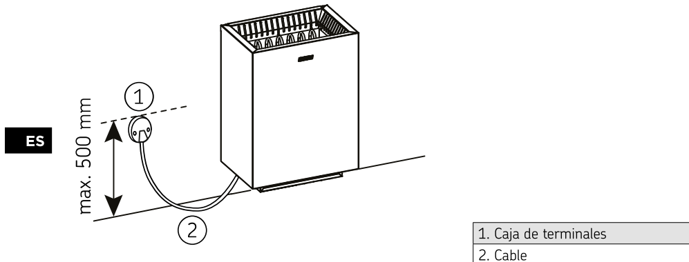
Figura 4. Conexiones eléctricas
