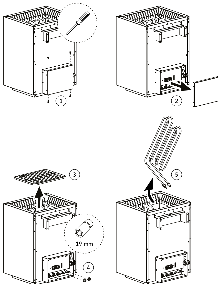
Figura 14. Sustitución de los elementos calefactores
