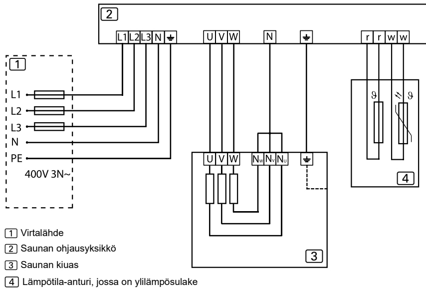
FI Kuva 9. KytKentäkaavio 400V 3N~
