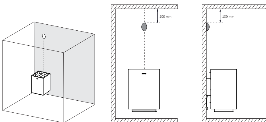
Figura 3. Instalación del sensor térmico en la pared
