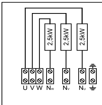
Joonis 7. Elektriskeem HLW75E
