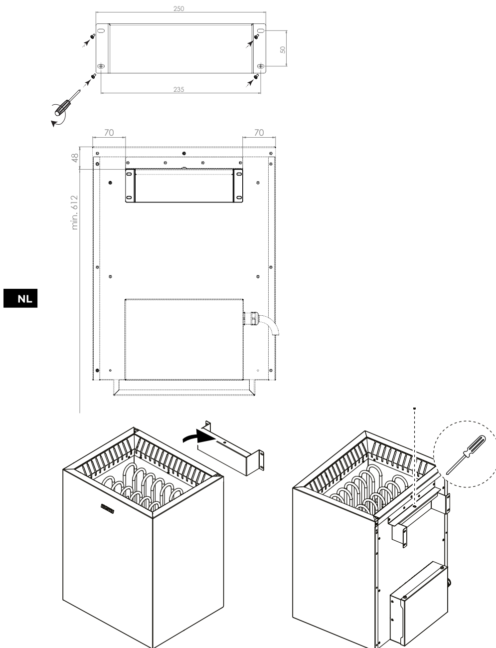
Figuur 2. Installatie saunakachel
