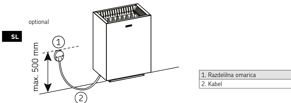
Slika 4. Električni priključki
