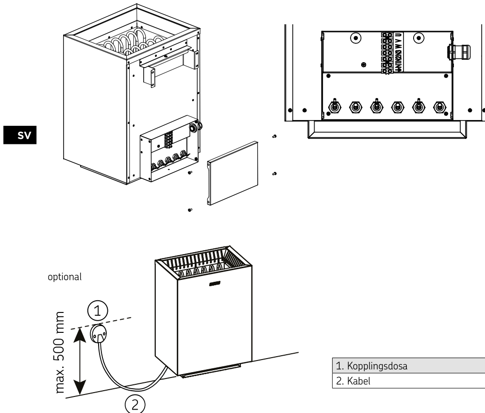
Bild 4. Elinstallation
