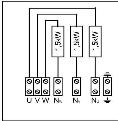
Bild 5. Kopplingsschema HLW45E
