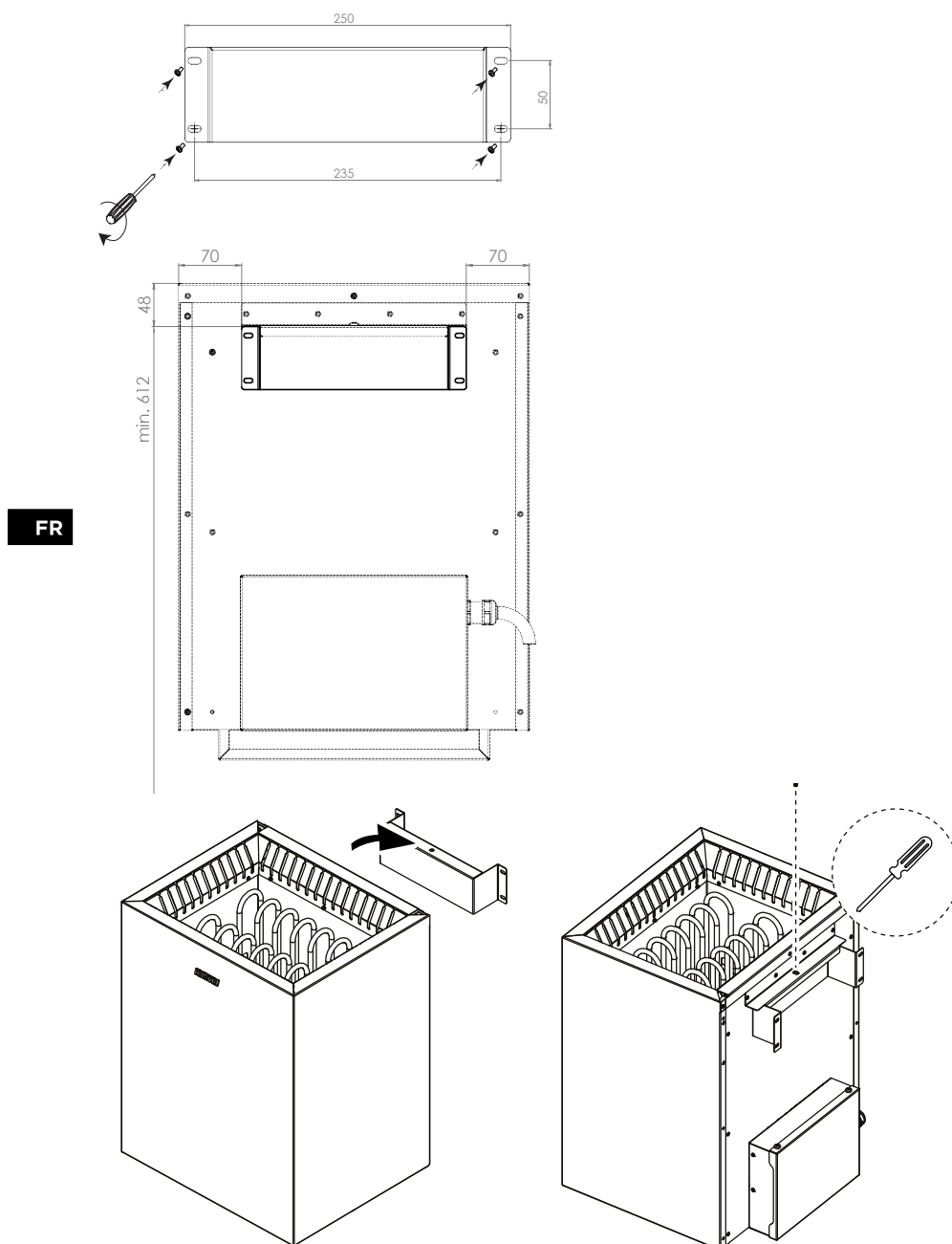
Figure 2. Installation du poêle pour sauna
