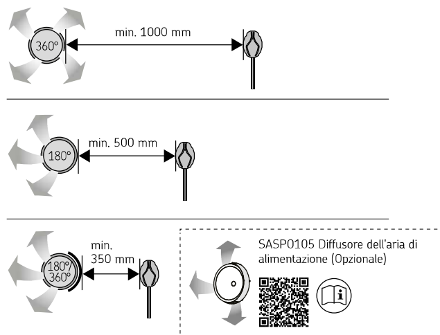
Figura 13. Distanza minima tra lo sfiato dell'aria di alimentazione e il sensore di temperatura.
