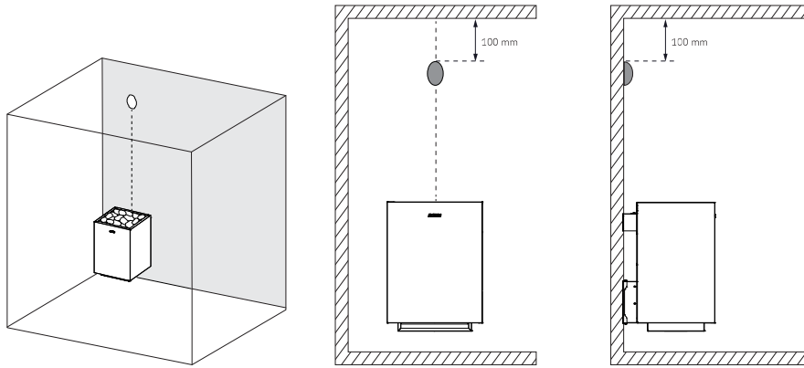
Kuva 3. Lämpöanturin asentaminen seinälle
