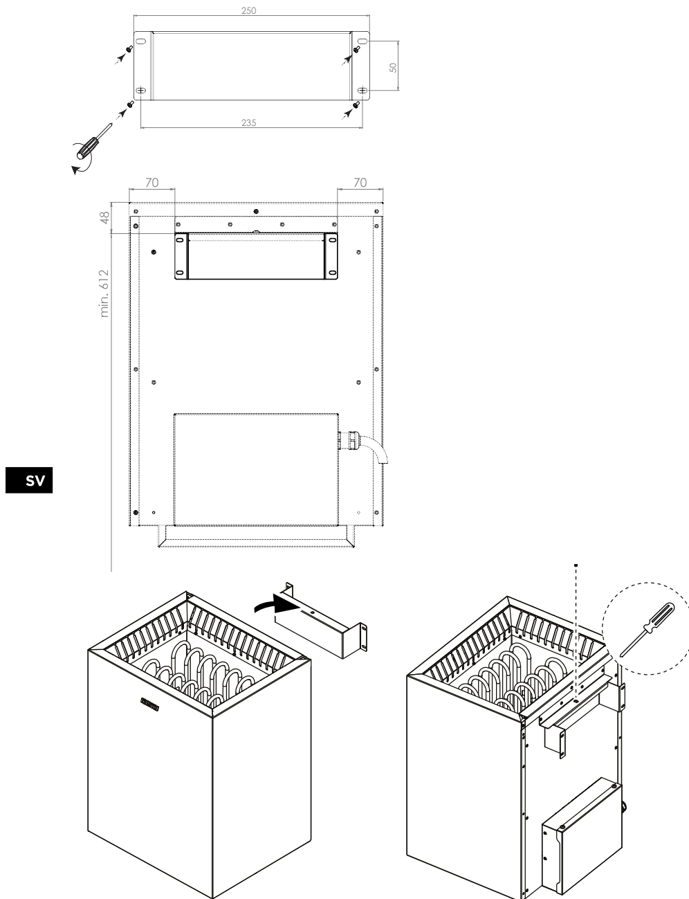
Bild 2. Installation av bastuaggregat
