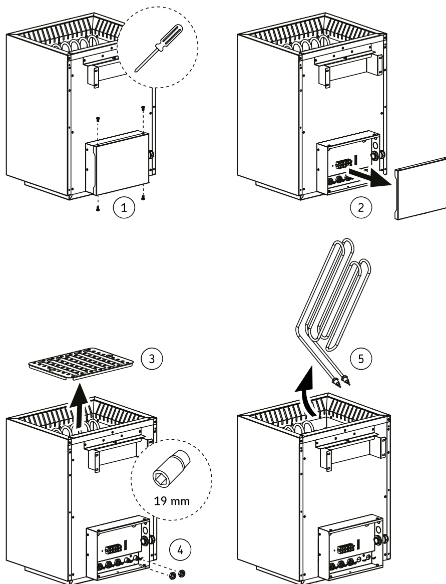
Bild 14. Byta värmeelement
