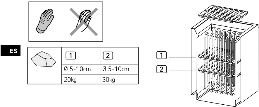
Figura 12. Colocación de las piedras de la sauna
