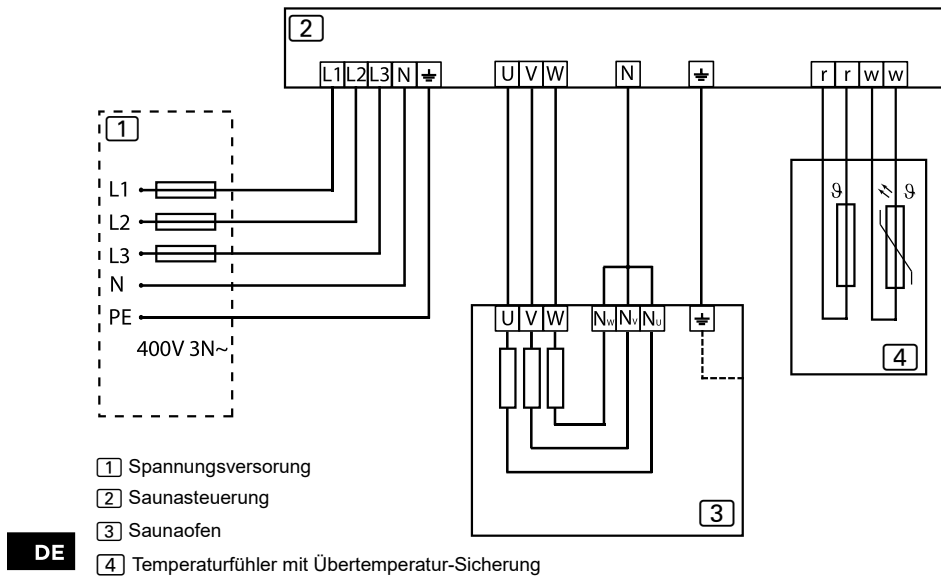
Abbildung 9. Anschlussplan 400V 3N~
