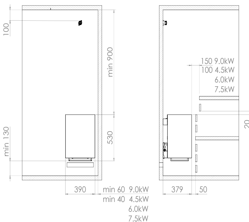
Obrázek 1 Bezpečnostní vzdálenosti
