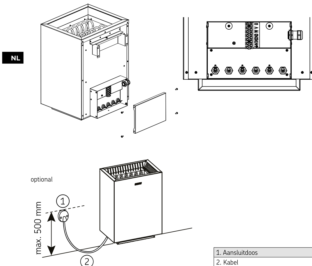
Figuur 4. Elektrische aansluitingen
