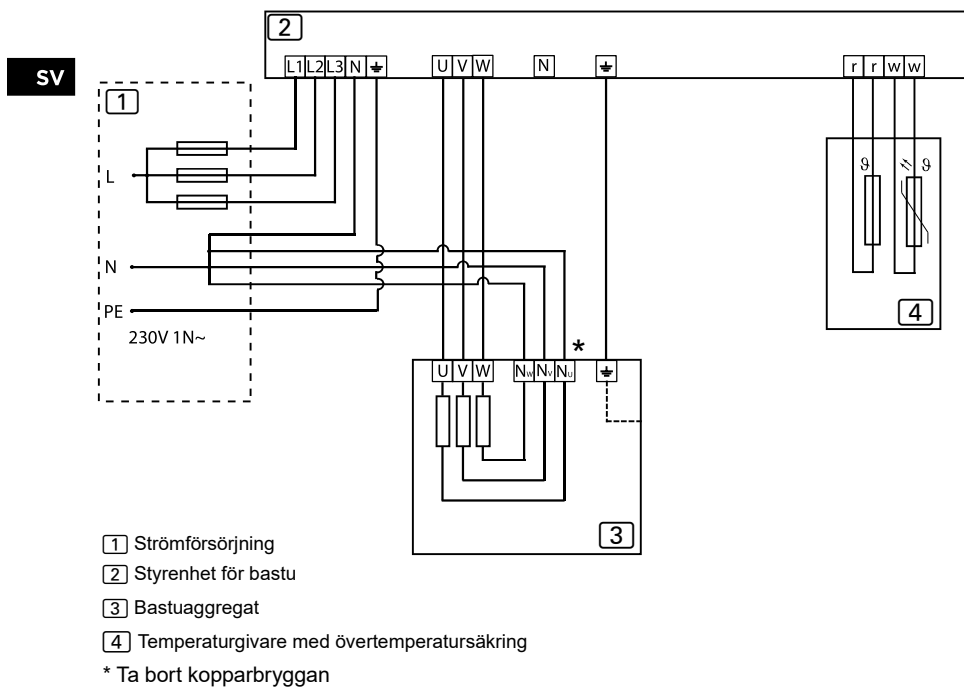
Bild 10. Kopplingsschema 230V 1N~
