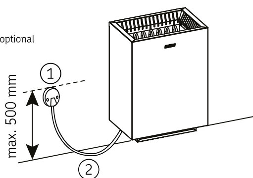
Obrázek 4 Elektrické připojení
