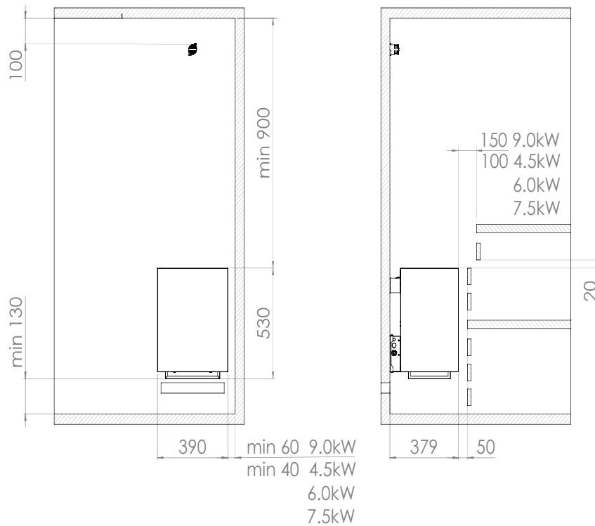
Kuva 1. Suojaetäisyydet
