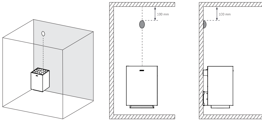
Kuva 3. Lämpöanturin asentaminen seinälle
