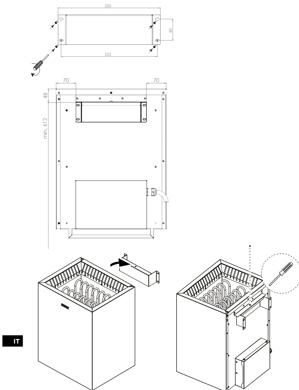
Figura 2. Installazione della stufa per sauna
