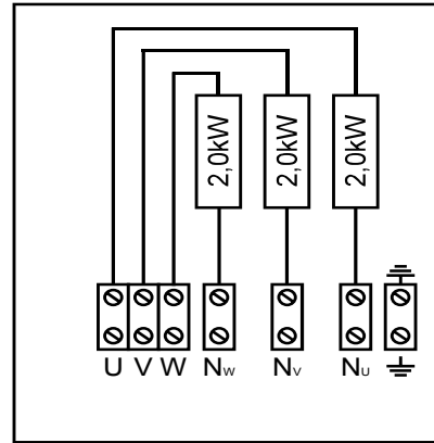
Bild 6. Kopplungsschema HLW60E
