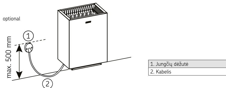
4 pav. Elektros jungtys
