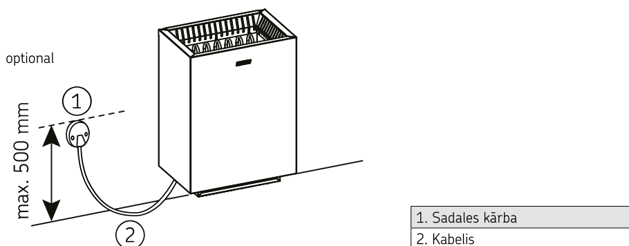
4. attēls. Elektroapgādes pieslēgumi
