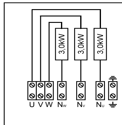
Bild 8. Kopplungsschema HLW90E
