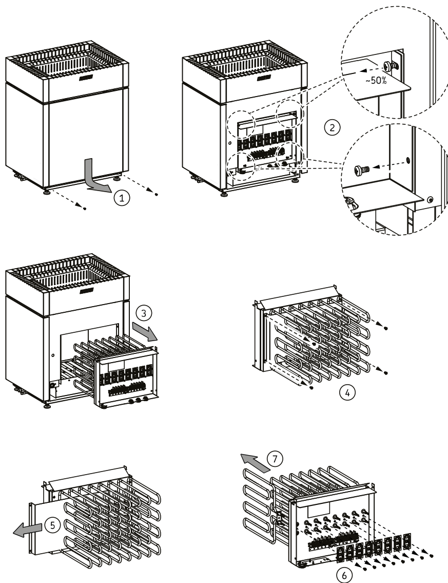
11 pav. Kaitintuvų keitimas
