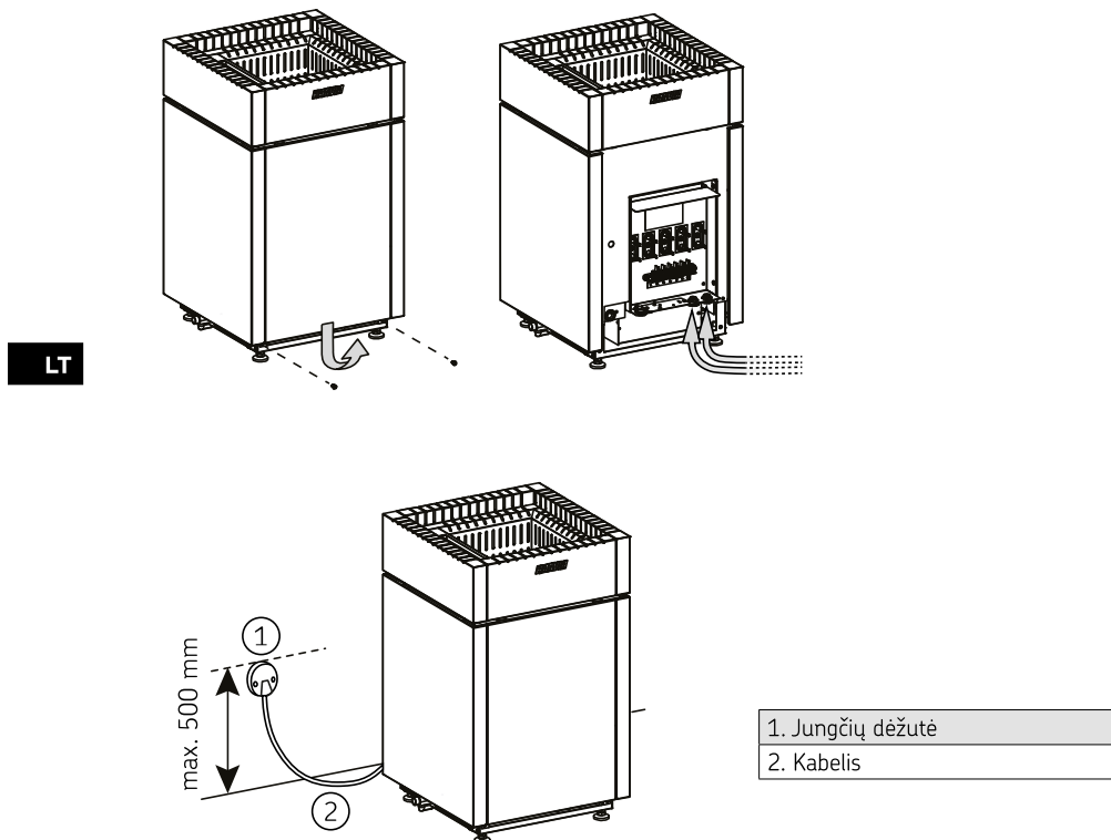
4 pav. Elektros jungtys
