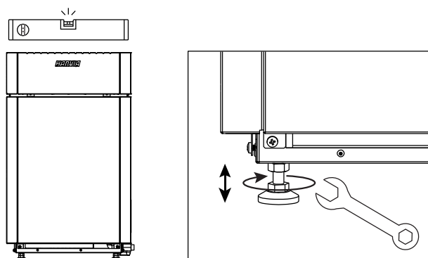
Рисунок 2. Установка каменки
