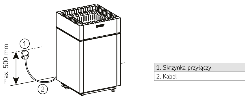
Rysunek 4. Połączenia elektryczne
