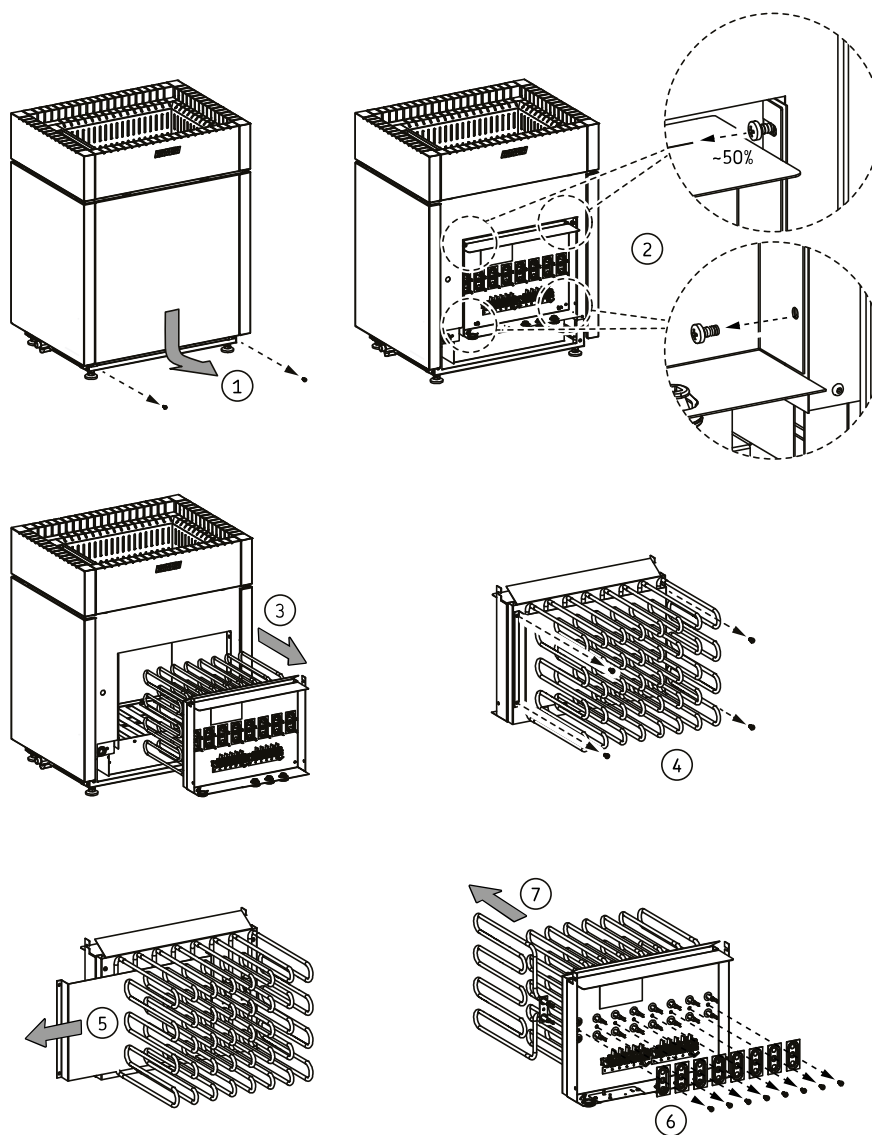
Obrázek 11 Výměna topných těles
