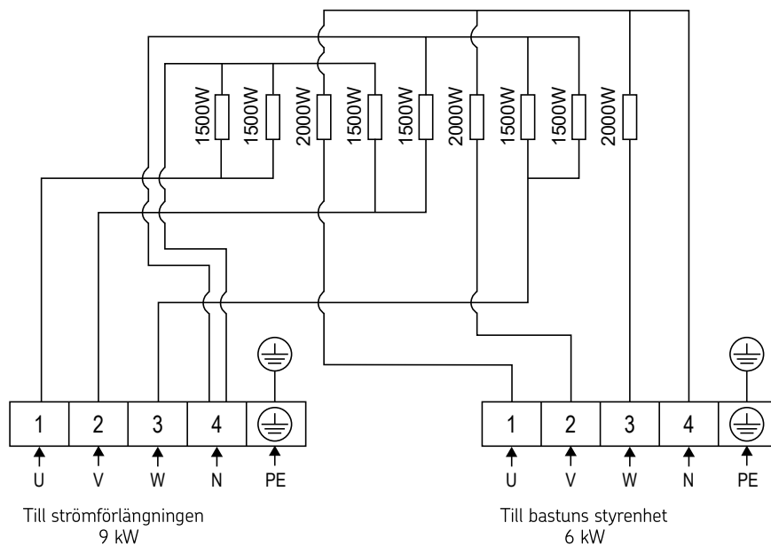
Bild 8. Kopplingsschema QU150E
