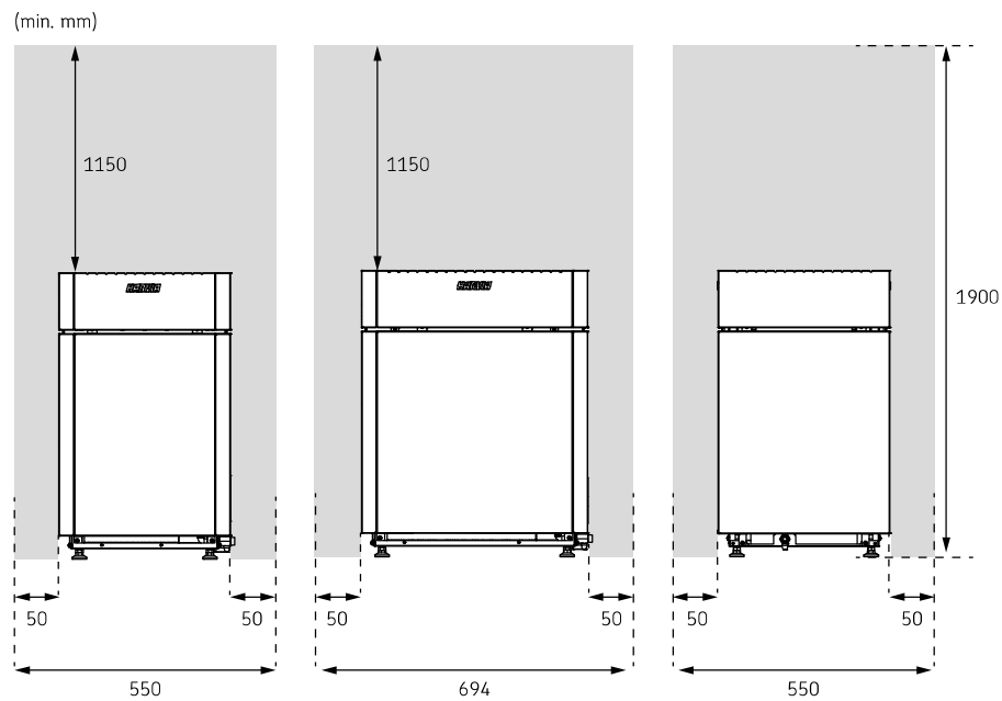
Figura 1. Distanza di sicurezza
