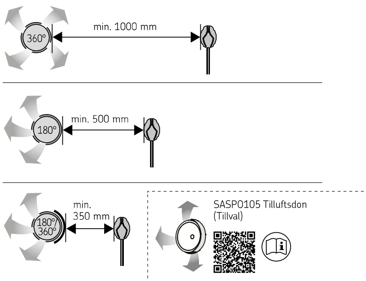
Bild 10. Minimiumstånd mellan tilluftsventil och temperaturgivare.
