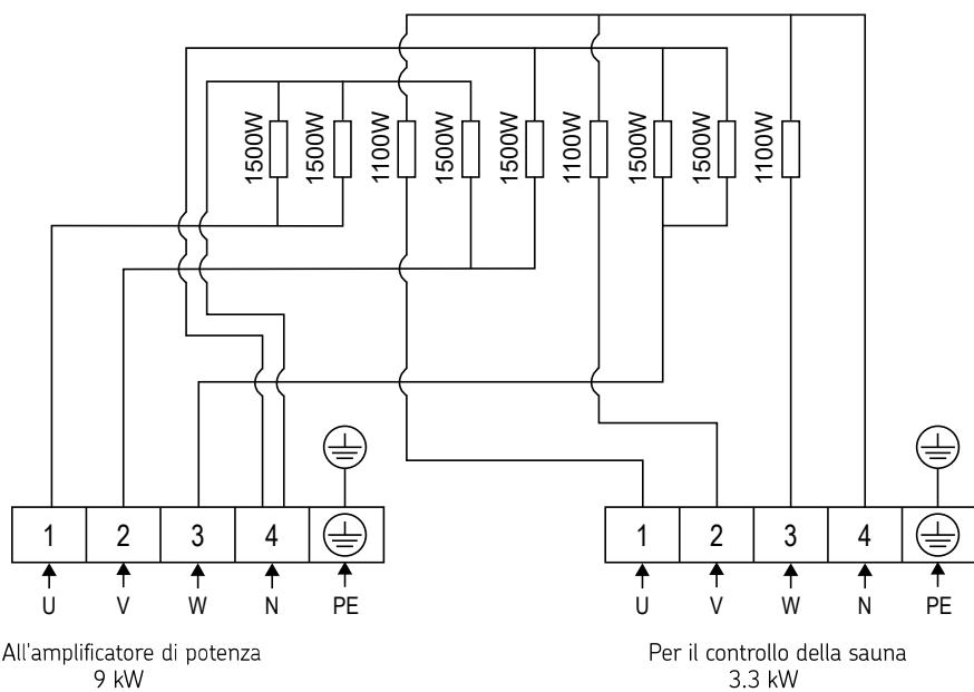
Figura 7. Schema elettrico QU120E
