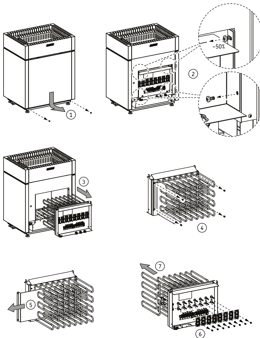
Figura 11. Sostituzione delle resistenze
