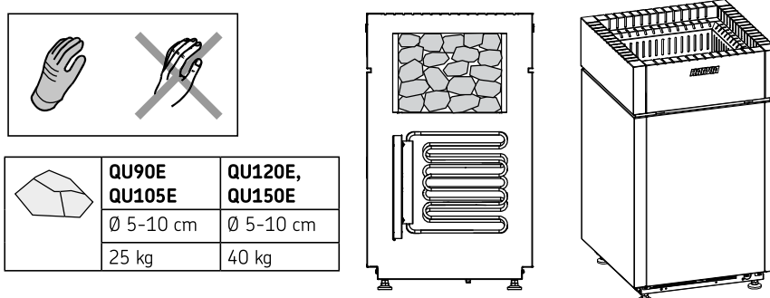
Figuur 8. Saunastenen plaatsen
