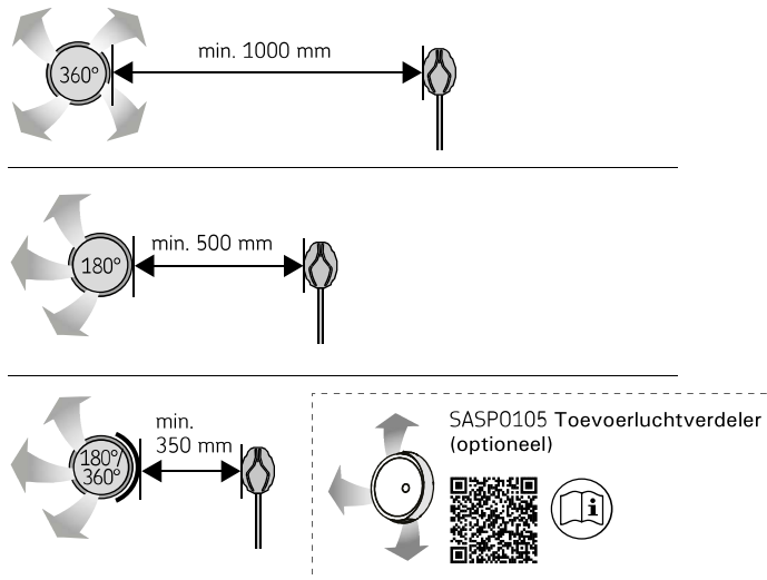
Figuur 10. Minimale afstand van de luchttoevoerklep tot de temperatuursensor.
