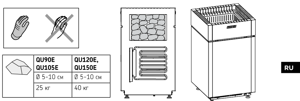
Рисунок 9. Наполнение каменки камнями
