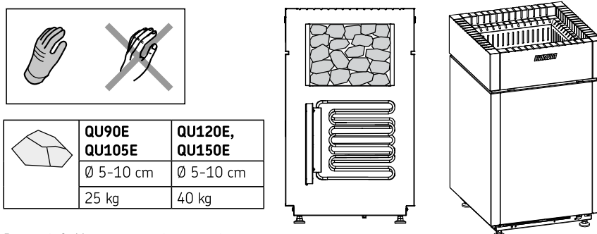
Rysunek 9. Umieszczanie kamieni do sauny
