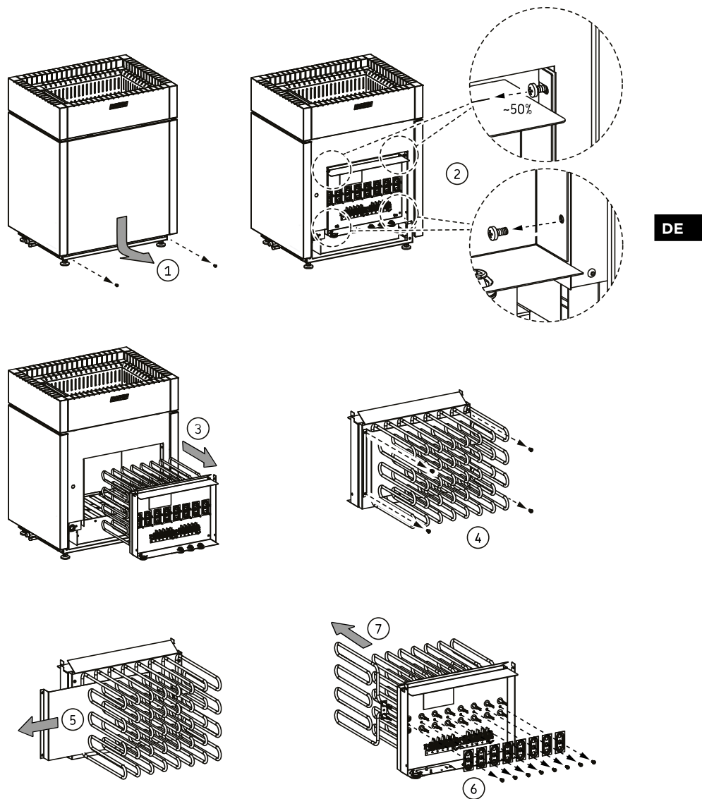
Abbildung 11. Auswechseln der Heizelemente
