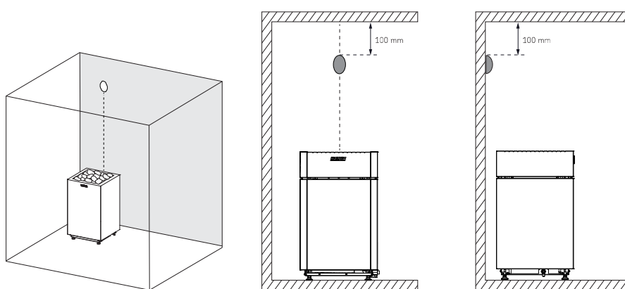
Figure 3a. Installation du capteur de chaleur au mur
