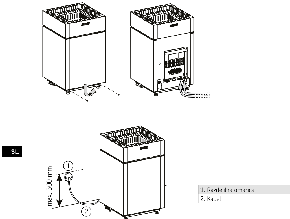
Slika 4. Električni priključki
