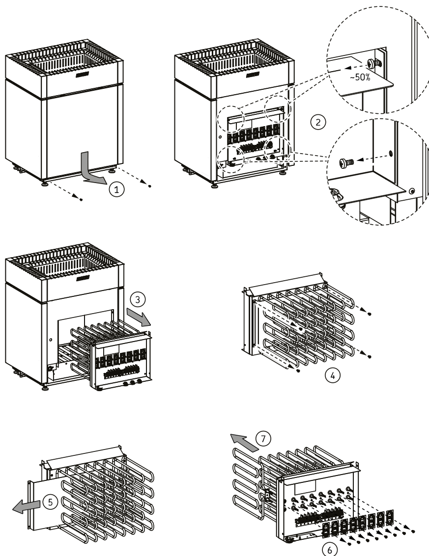
Joonis 11. Kütteelementide vahetamine
