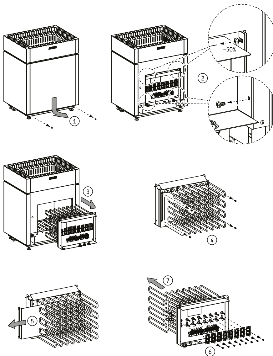
Rysunek 11. Wymiana elementów grzejnych
