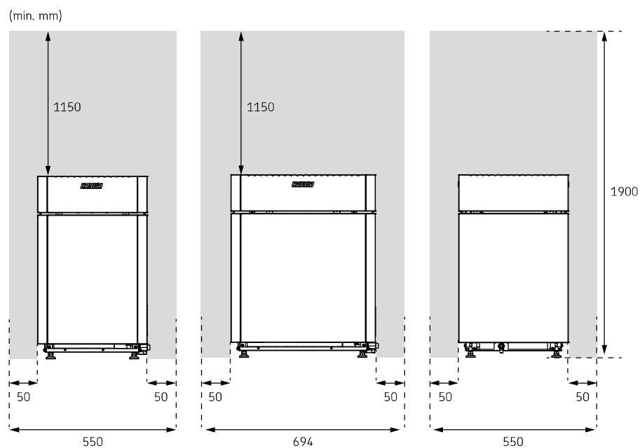
Figure 1. Distances de sécurité
