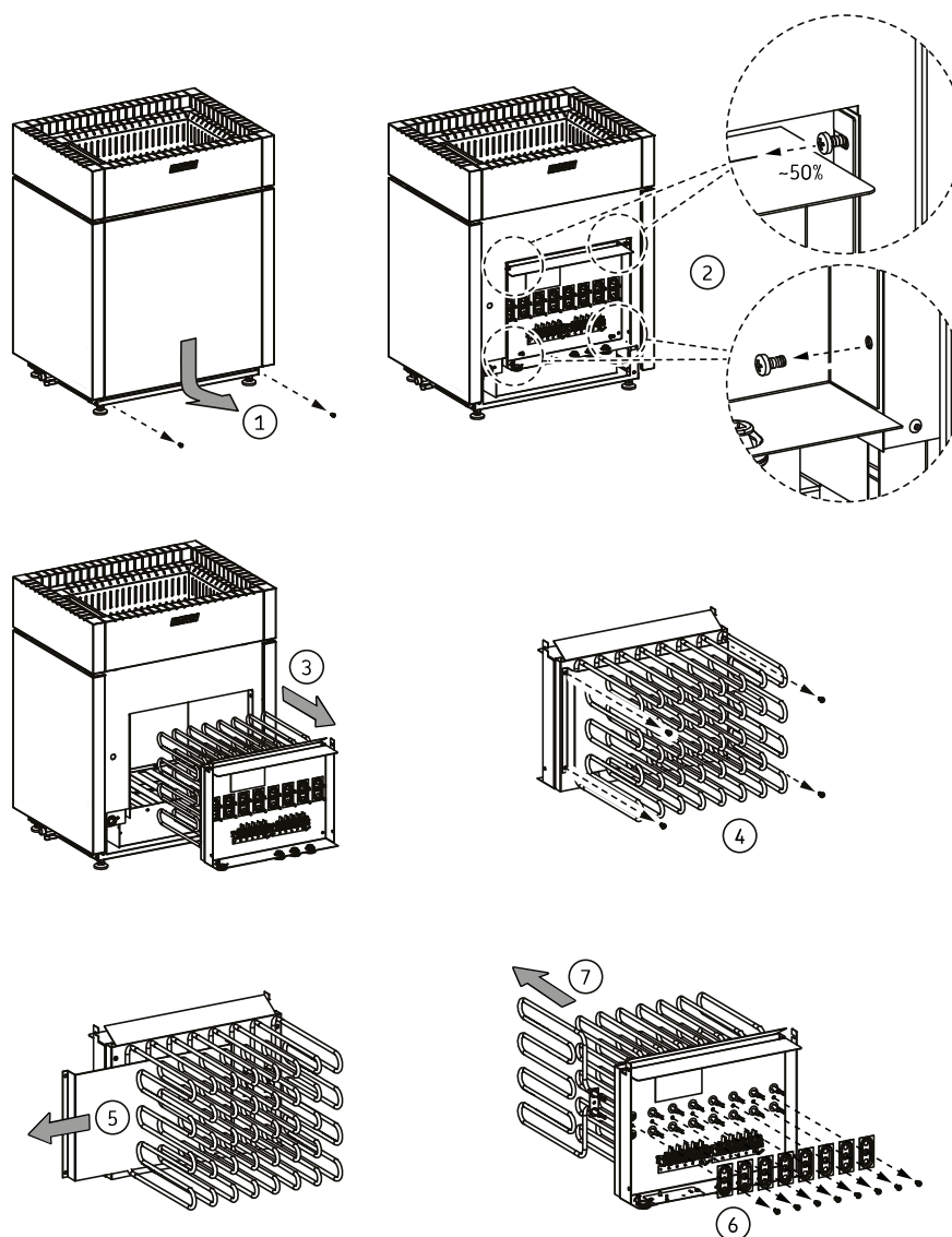
Figura 11. Sustitución de los elementos calefactores
