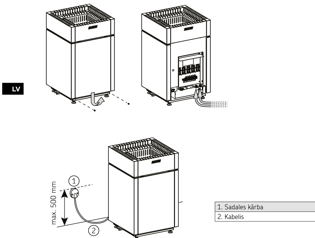
4. attēls. Elektroapgādes pieslēgumi
