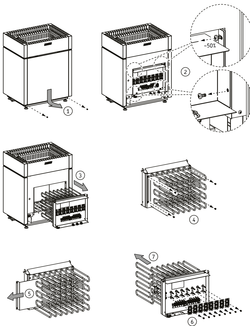
Slika 11. Menjava grelnih elementov
