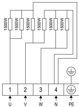
Obrázek 5. Schéma zapojení QU90E
