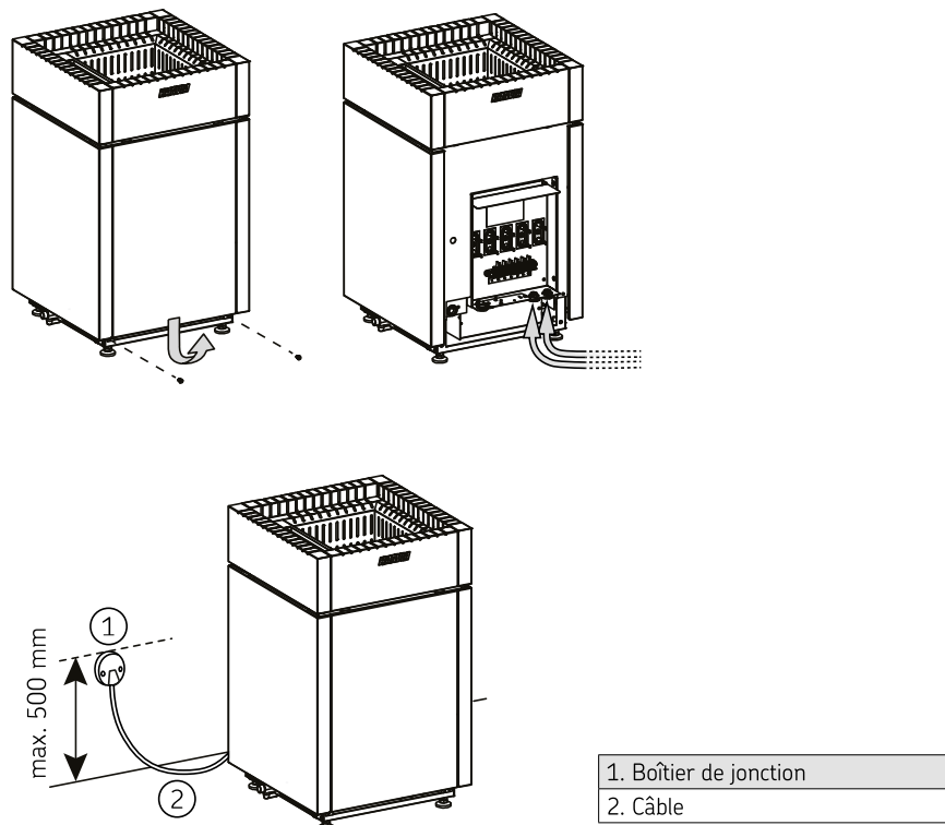
Figure 4. Raccordements électriques
