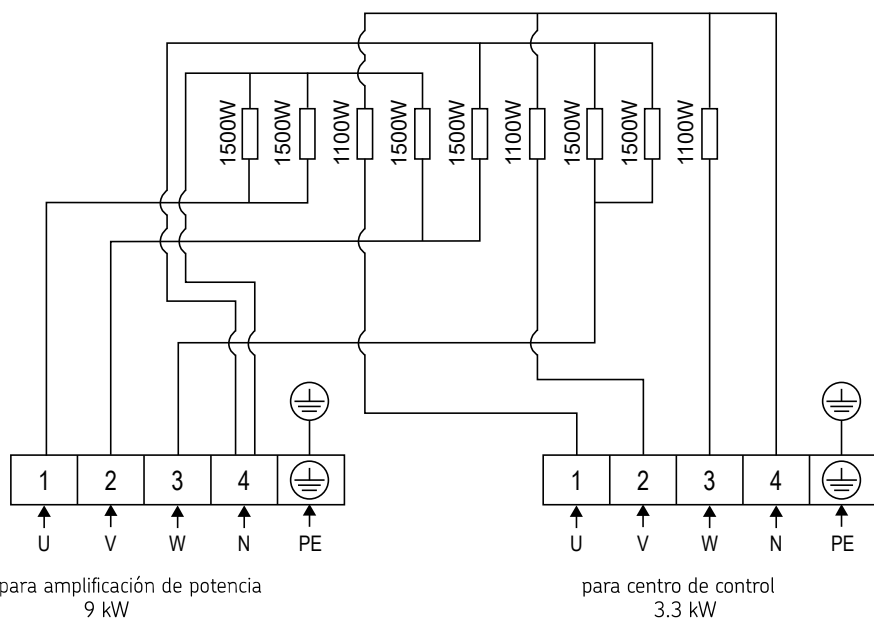
Figura 7. Esquema eléctrico QU120E
