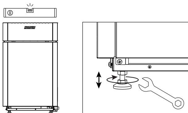
Kuva 2. Kiukaan asennus
