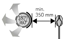
Rysunek 10. Minimalna odległość otworu wentylacyjnego od czujnika.
