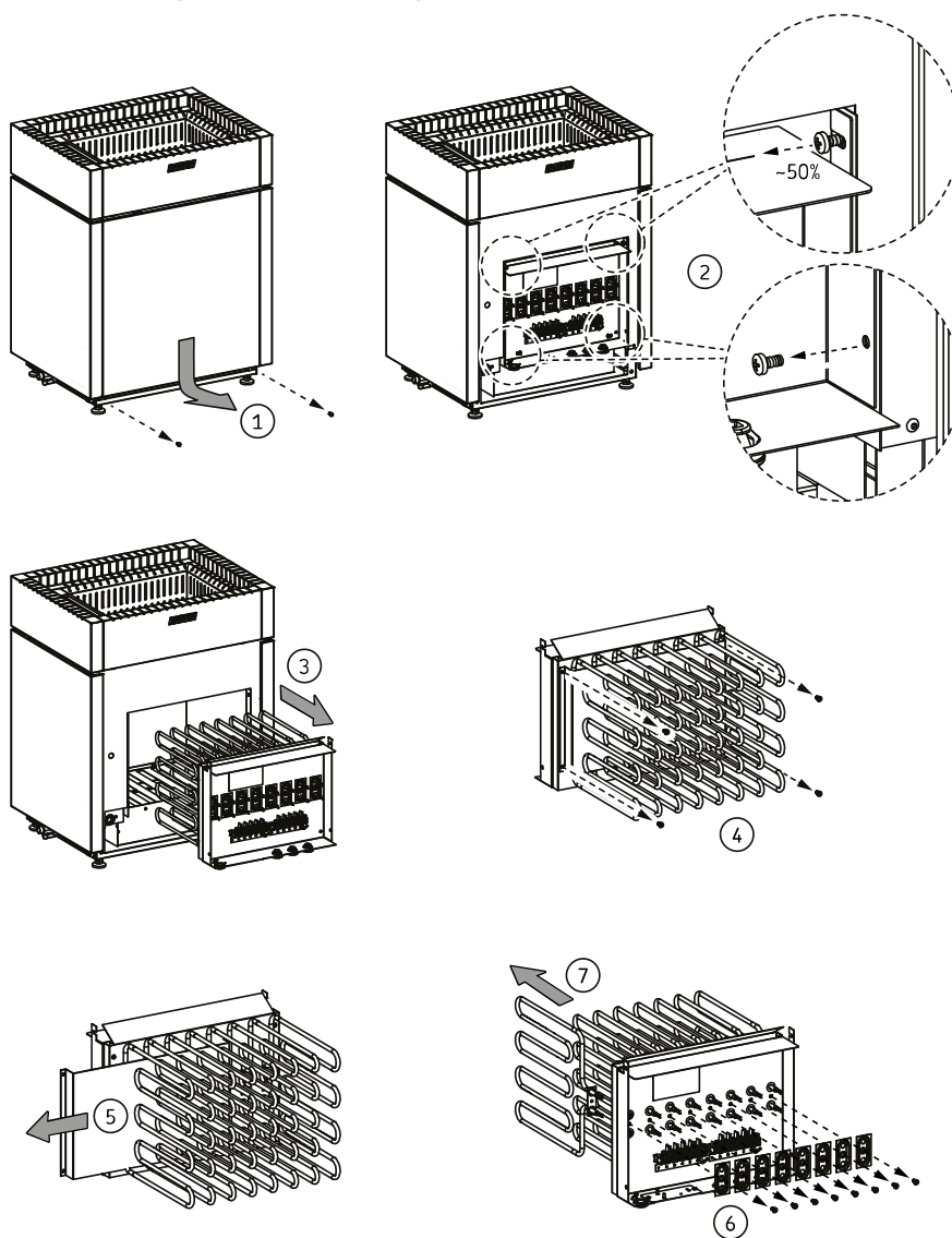
Figuur 11. Verwarmingselementen vervangen
