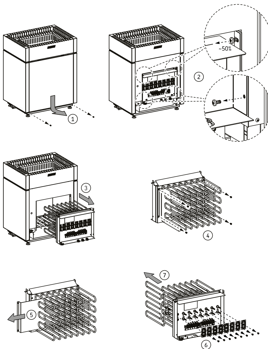
Figure 11. Remplacement des résistances
