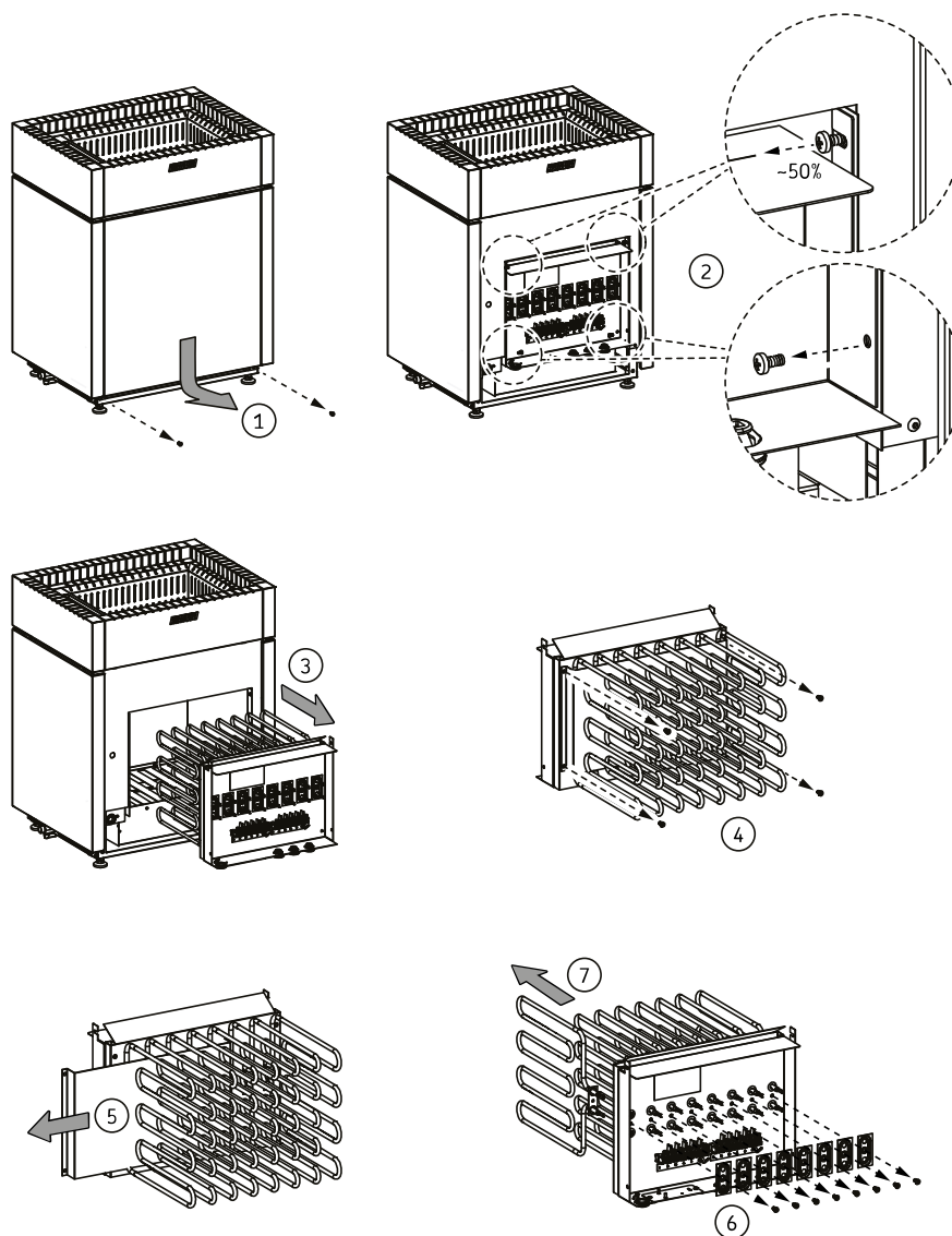
Bild 11. Byta värmeelement
