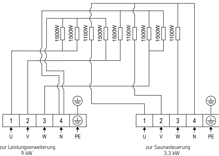
Abbildung 7. Verdrahtungsschema QU120E
