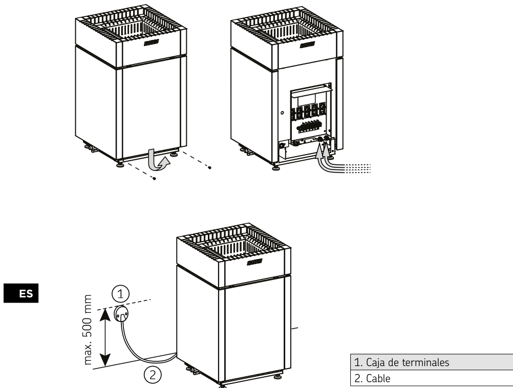
Figura 4. Conexiones eléctricas
