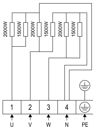
Figure 6. Schéma de câblage QU105E
