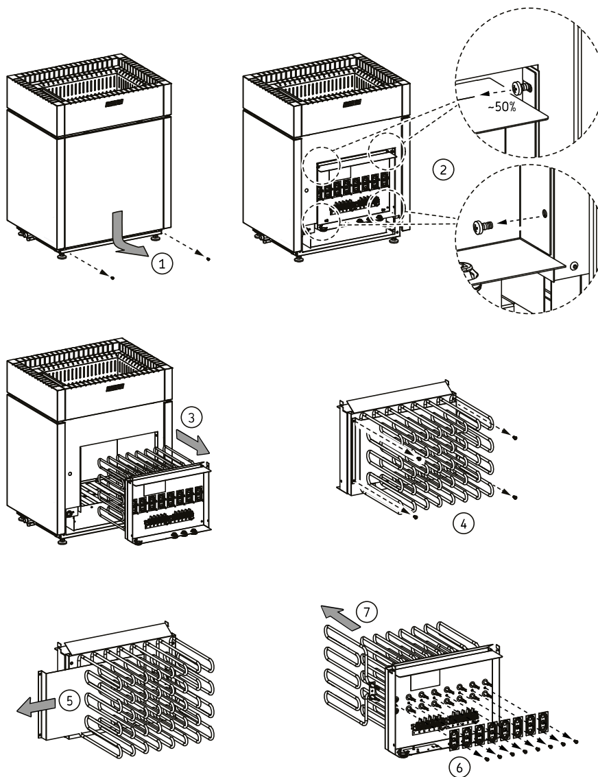
11. attēls. Sildelementu maiņa
