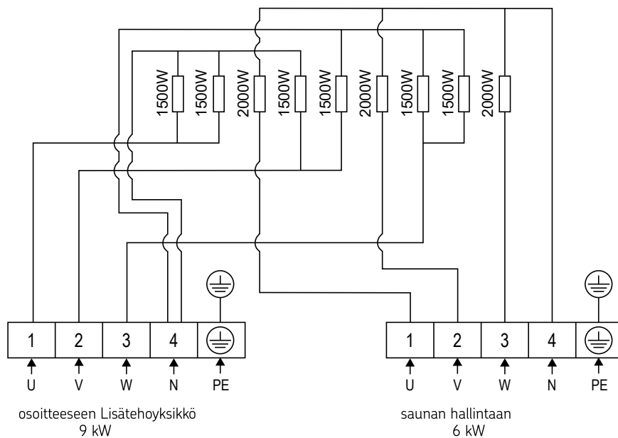
Kuva 8. Kytentäkaavio QU150E
