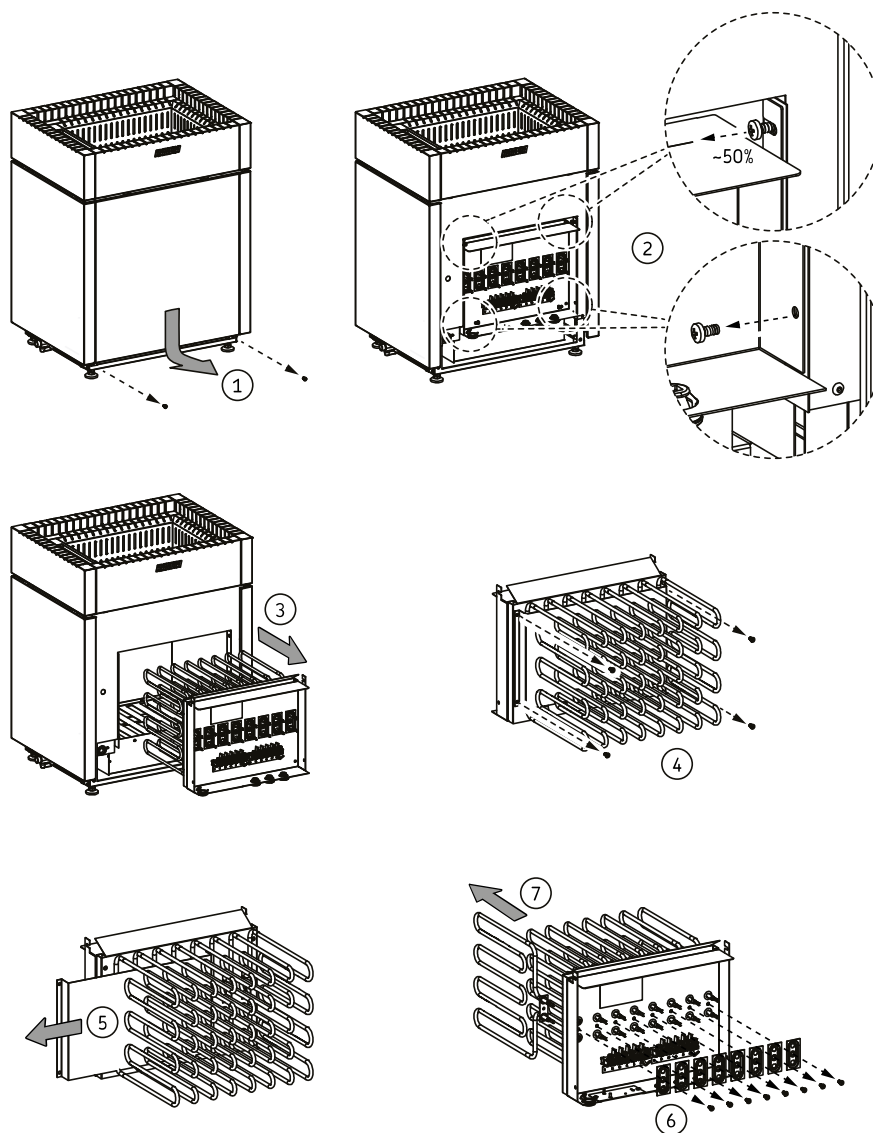
Kuva 11. Vastusten vaihtaminen
