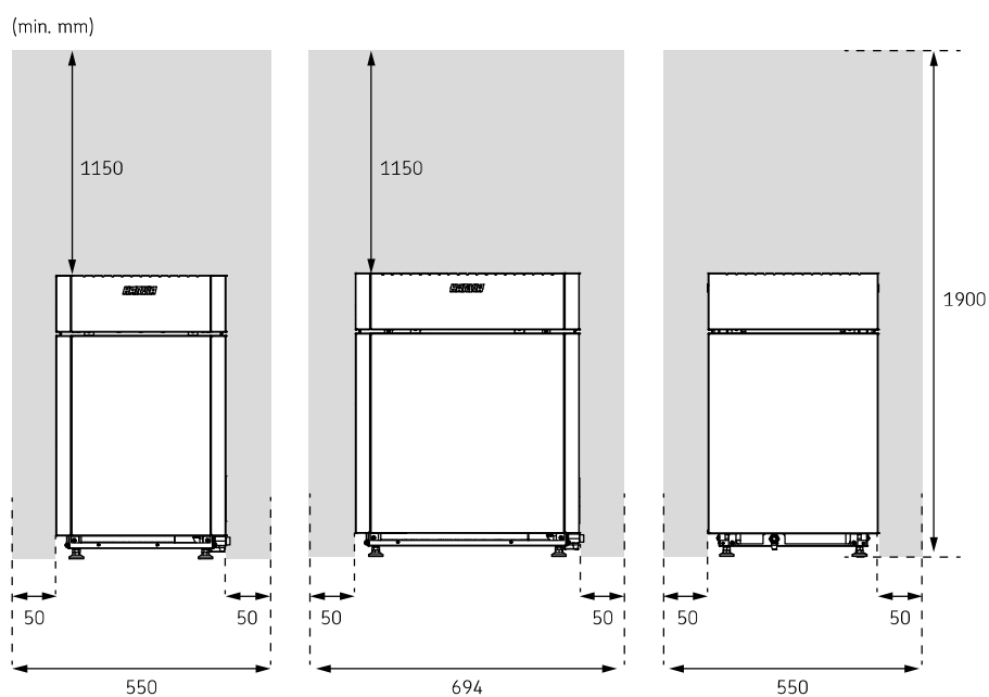
Figuur 1. Veiligheidsafstanden
