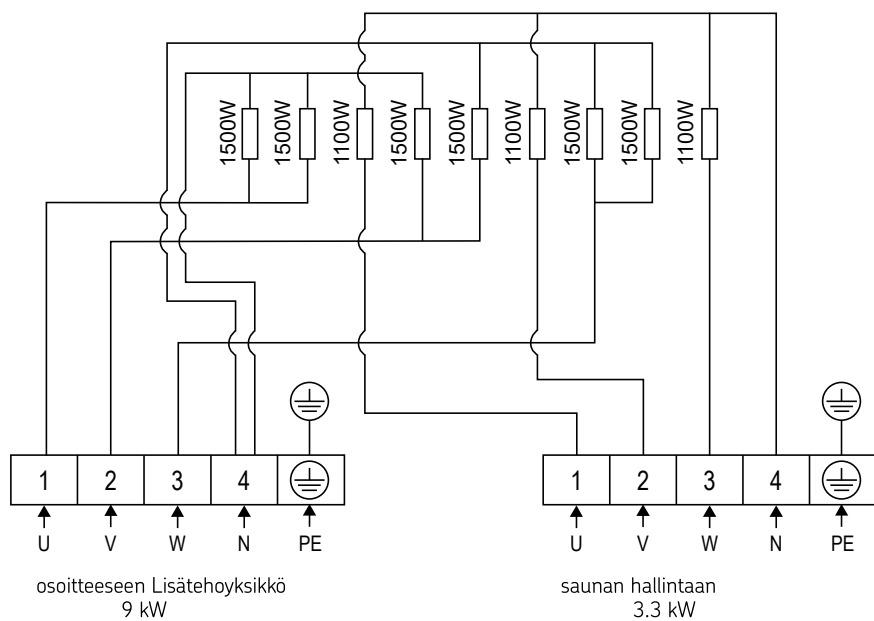
Kuva 7. Kytentäkaavio QU120E
