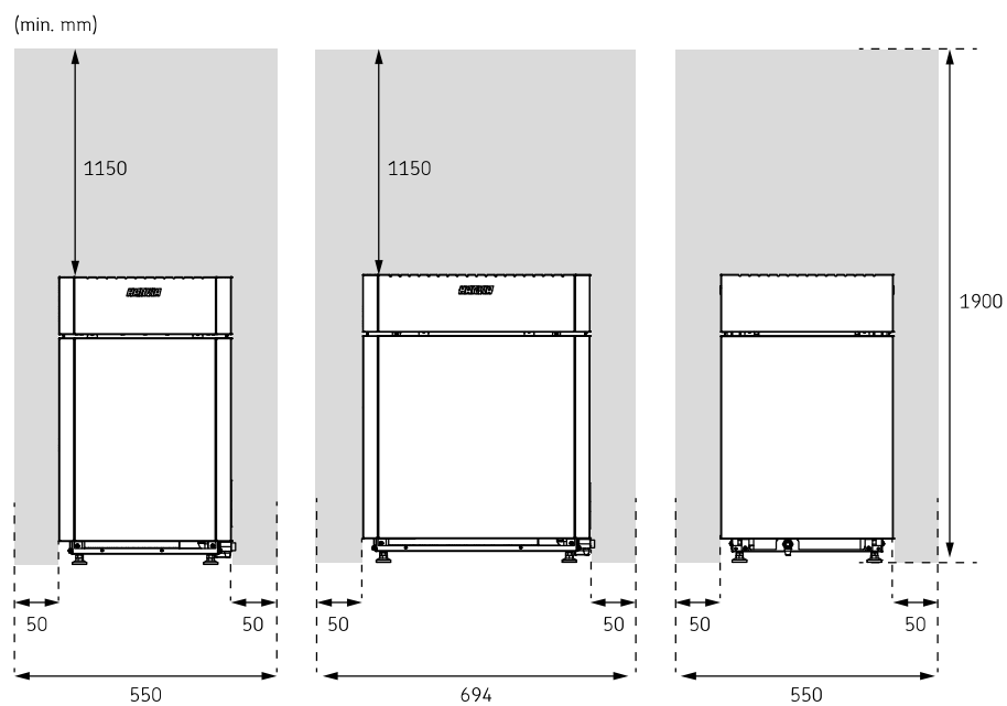
1. attēls. Droši attālumi
