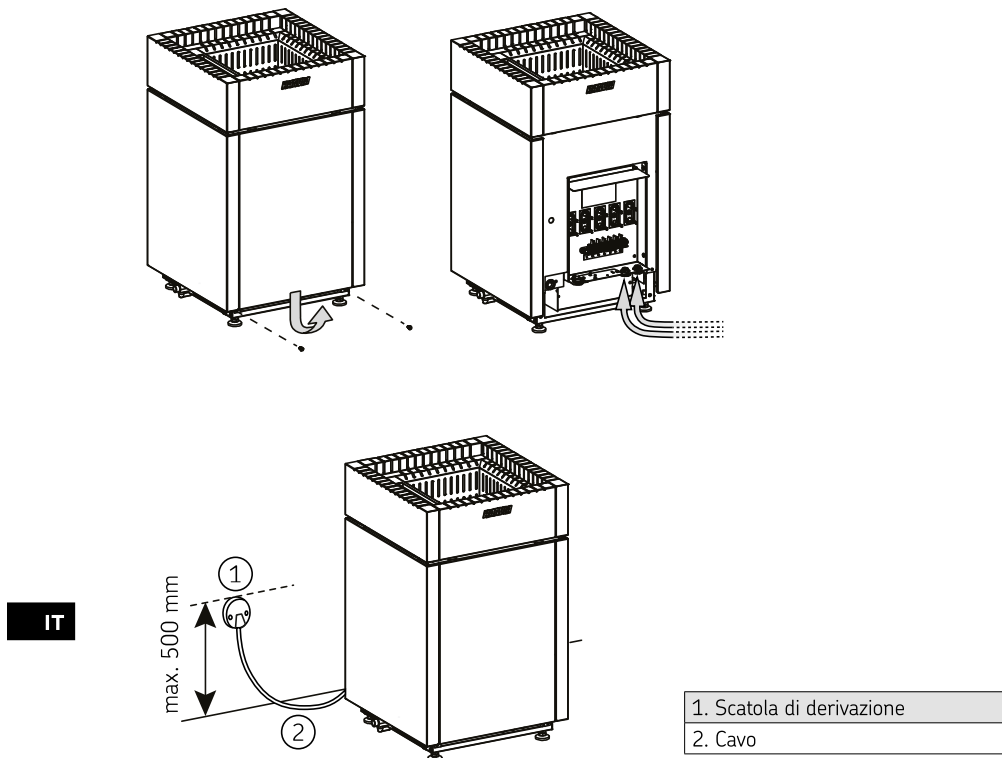
Figura 4. Collegamenti elettrici
