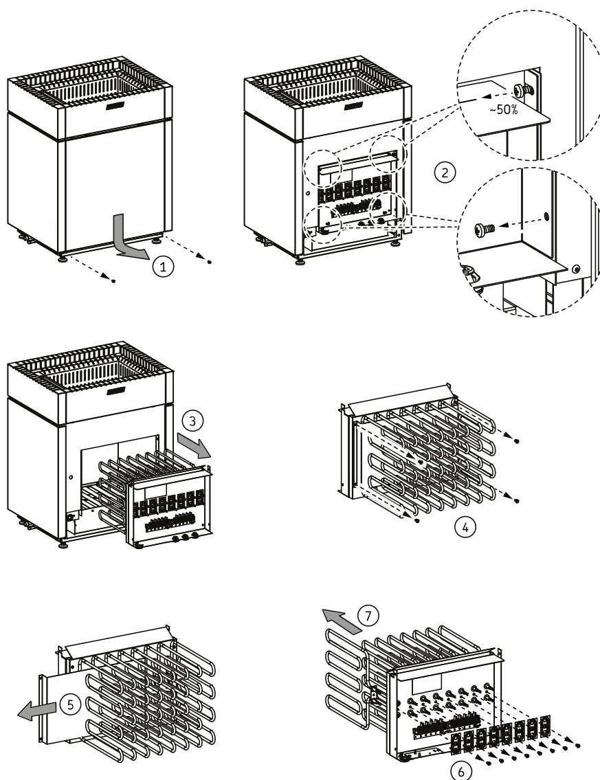
Рисунок 11. Замена нагревательных элементов
