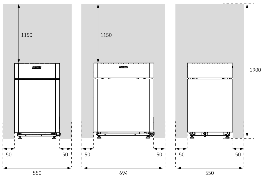
Bild 1. Säkerhetsavstånd
