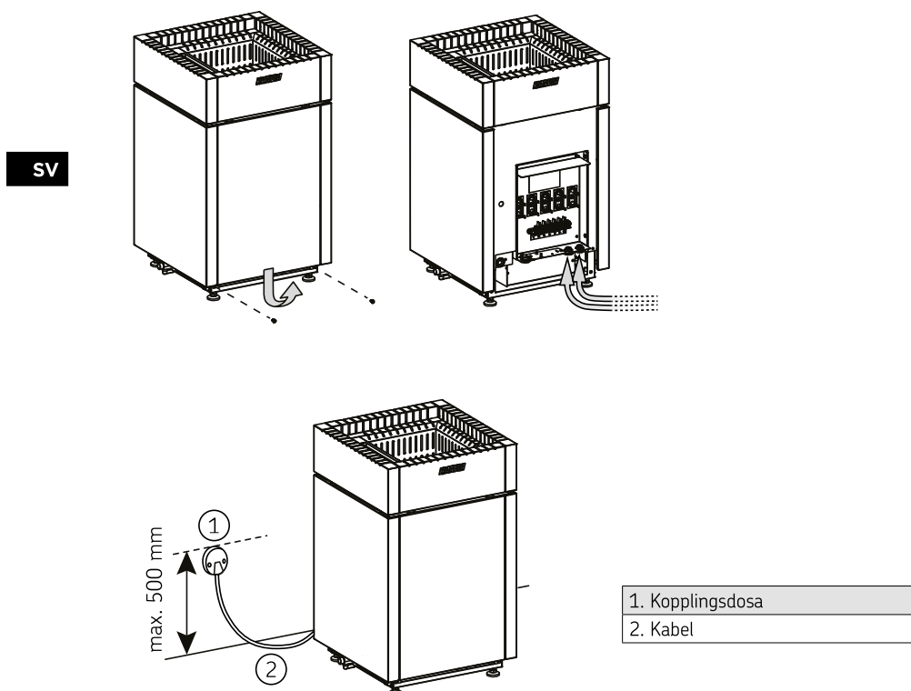
Bild 4. Einstallation
