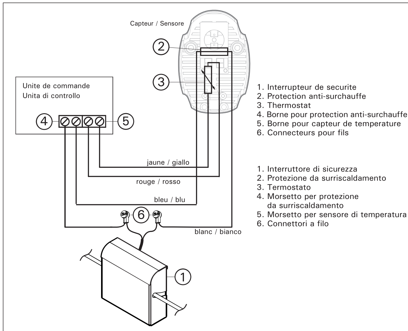
Figure 6. Schema de câblage pour les unités de commande sans bornes pour les fonctions de sécurité. Figura 6. Schema elettrico per centraline senza morsetti dedicati alle funzioni di sicurezza.
