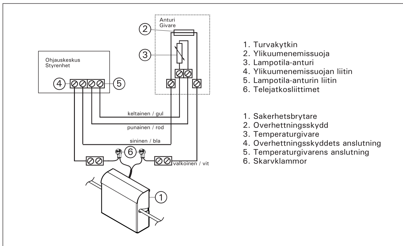
Kuva 5. Kytentakaavio Sentiotec:n ohjauskeskuksille Bild 5. Kopplingsschema for Sentiotechs styrenheter
