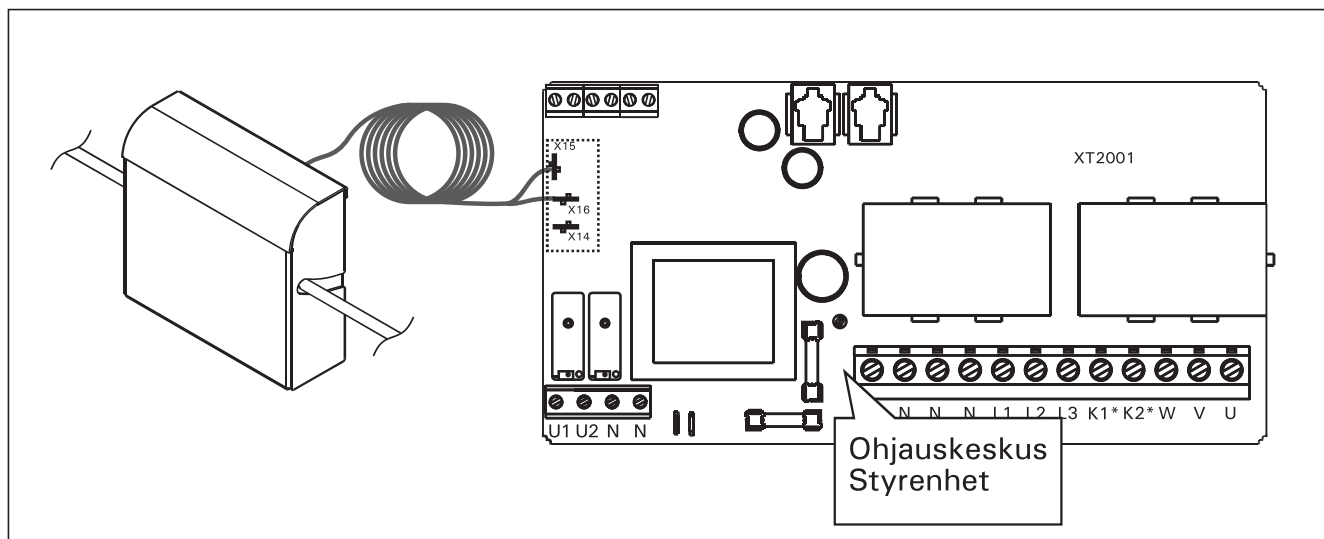
Kuva 4. Kytentakaavio Harvian ohjauskeskuksille Bild 4. Kopplingsschema for Harvias styrenheter
