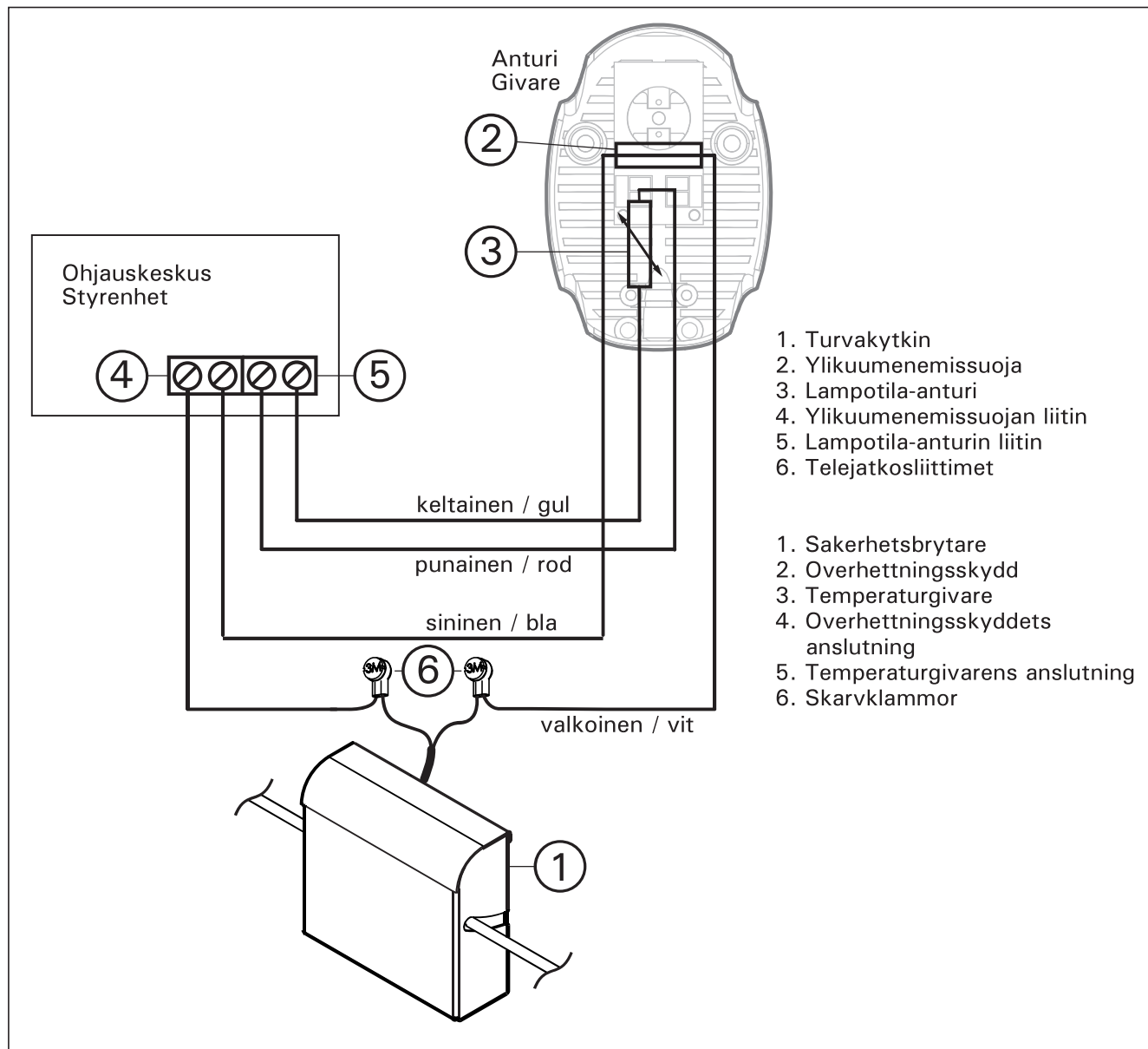
Kuva 6. Kytentakaavio ohjauskeskuksille, joissa ei ole turvalaiteliitäntää Bild 6. Kopplingsschema for styrenheter utan intag för säkerhetsanordningar
