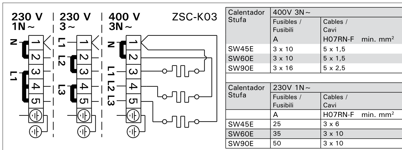
Figura 11b. Conexiones electricas (SW45E, SW60E, SW90E)
