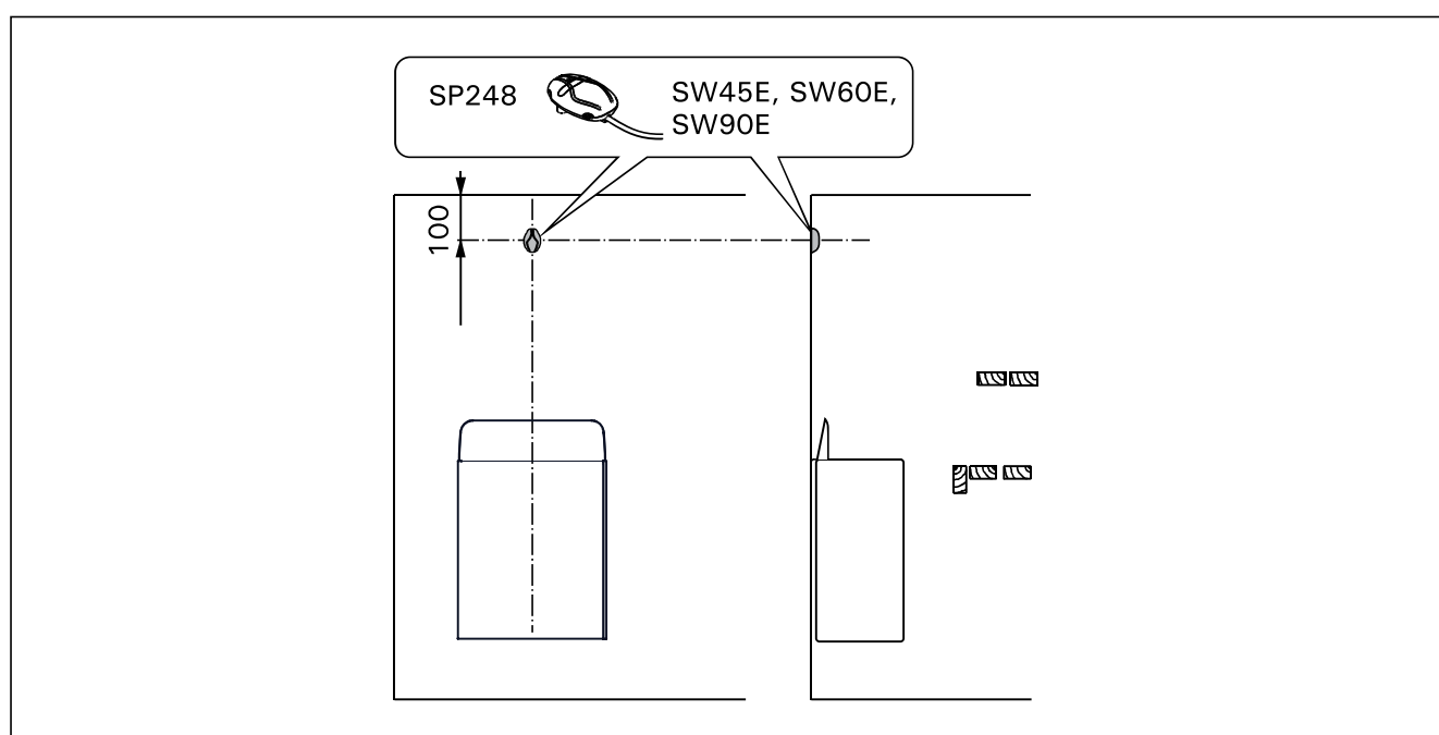
Figure 6. Instalacion del sensor de temperatura (todas las dimensiones en mil metros)
