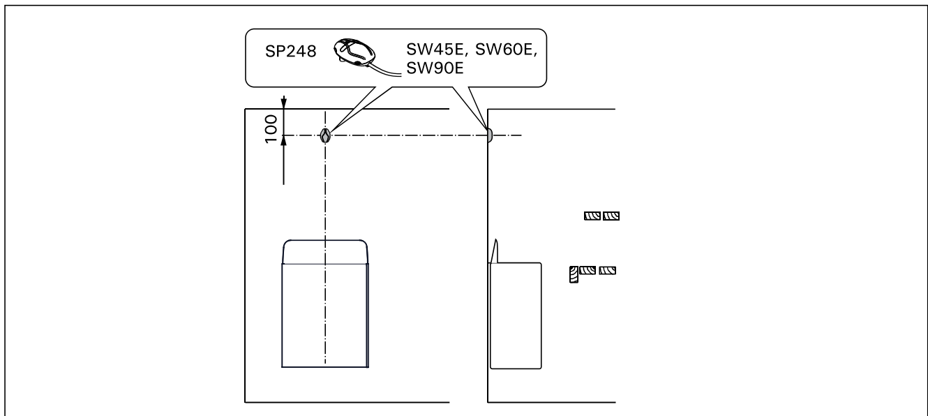
Kuva 6. Anturin asentaminen (mitat millimetreina)
