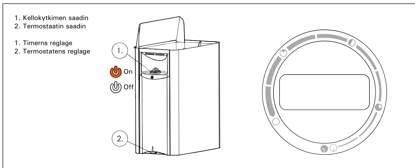
Kuva 2. Saatimet (SW45, SW60, SW80, SW90) Bild 2. Reglagen (SW45, SW60, SW80, SW90)
