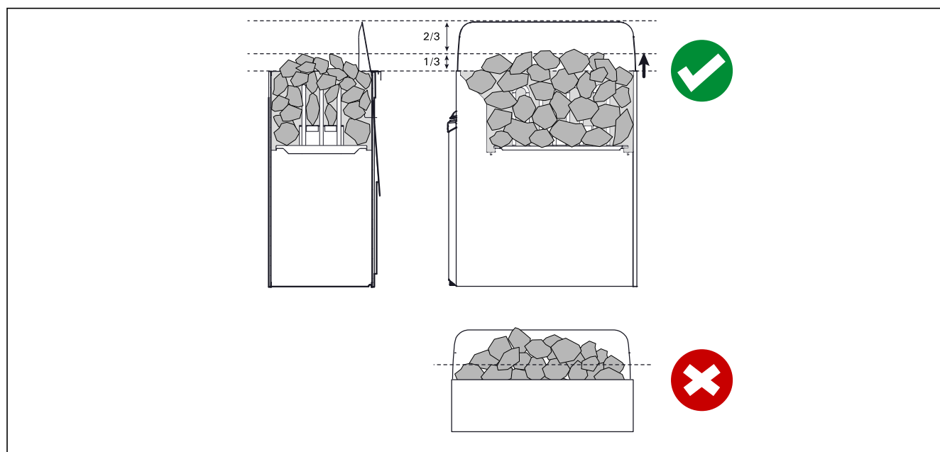
Figure 1. Empilement des pierres du poele
