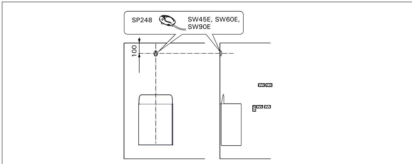
Рисунок 6. Установка датчиков (все размеры приведены в миллиметрах) Joonis 6. Anduri paigaldamine (koik mootmed millimeetrites)
