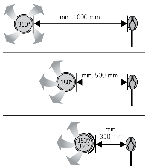
Kuva 4. Tuloilmaventtiilin vähimmäisetäisyys lampotila-anturiin. Bild 4. Minimavstånd mellan tilluftsventil och temperaturgivare.
