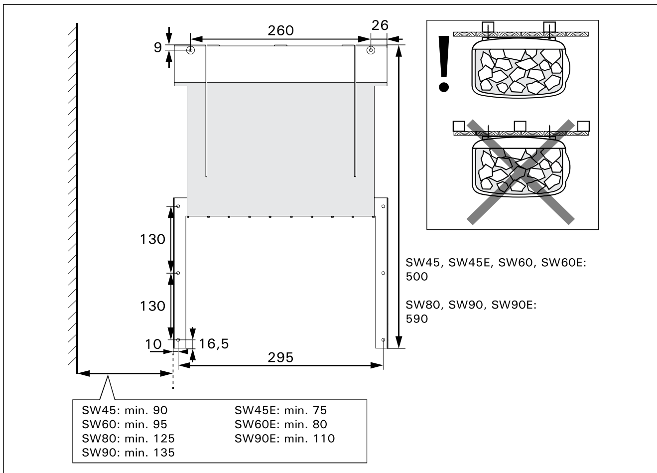
Рисунок 7. Настенный кронштейн, размеры в миллиметрах Joonis 7. Seinakinnitusraam, moodud millimeetrites
