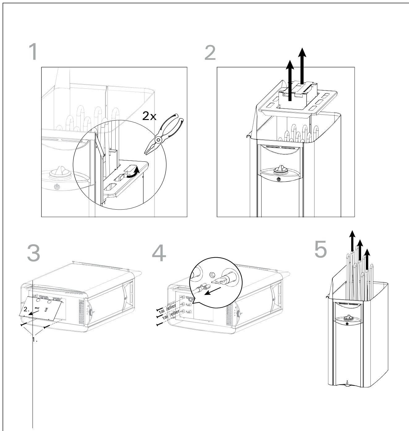
Figura 10. Sustitucion de los elementos calefactores Bild 10. Byte av element
