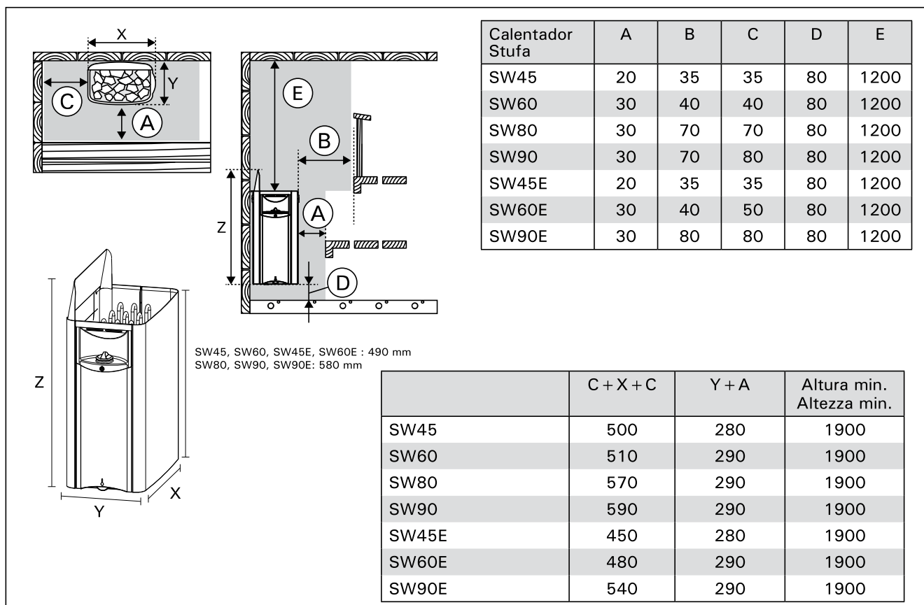
Figura 5. Distancias de seguridad (todas las dimensiones en mil metros)
