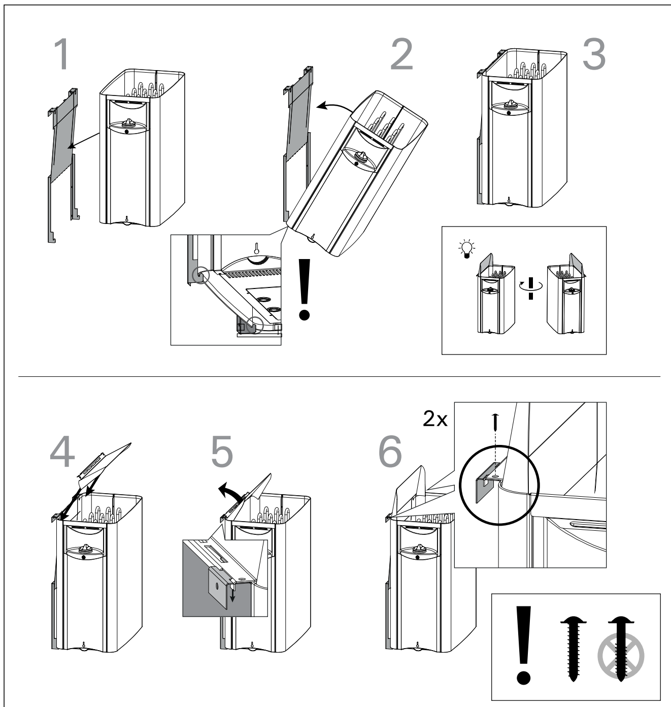
Figura 9. Fijacion del calentador a la pared Figura 9. Come fissare la stufa alla parete
