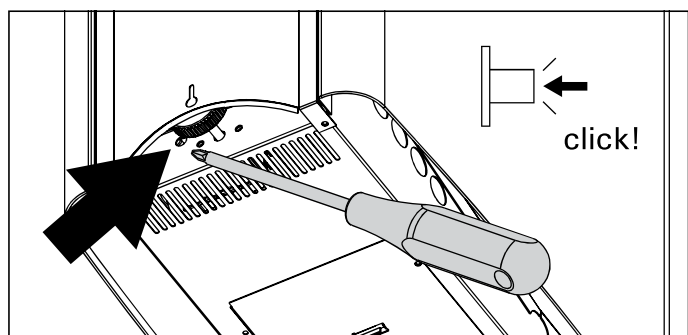
Kuva 12. Ylikuumenemissuojan palautus
