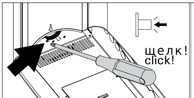
Рисунок 12. Восстановление рабочего состояния после срабатывания режима защиты от перегрева
