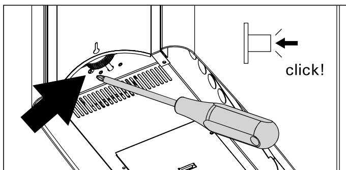
Figure 12. Reinitialisation de la securite-surchauffe Rys. 12. Restartowanie bezpiecznika termicznego
