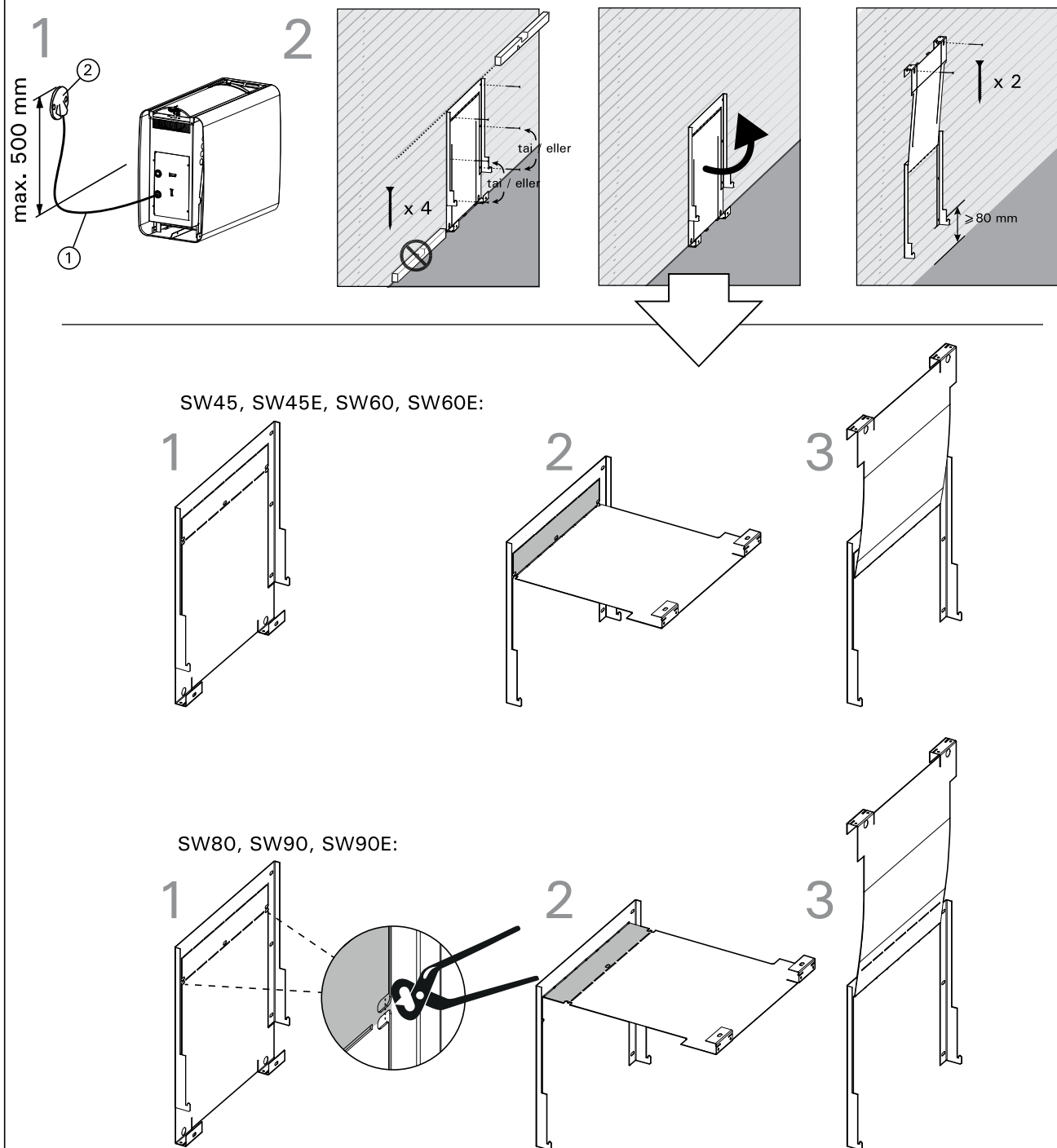
Kuva 8. Seinätelineen kiinnitys Bild 8. Montering av vaggkonsolen
