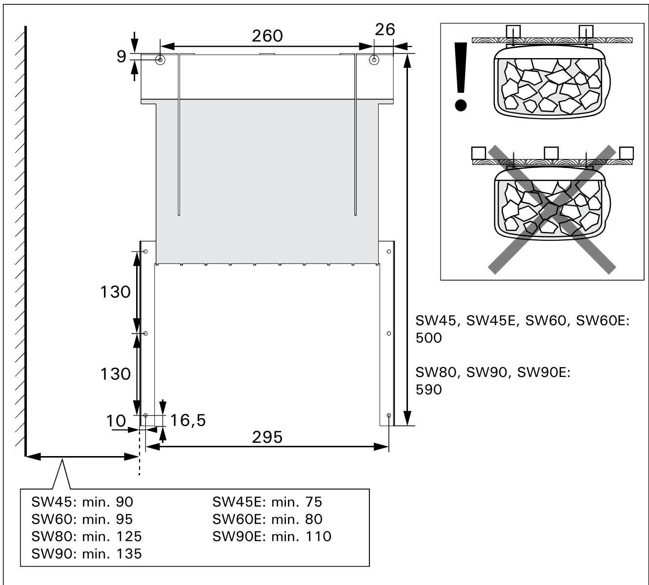
Kuva 7. Seinateline, mitat millimetreina
