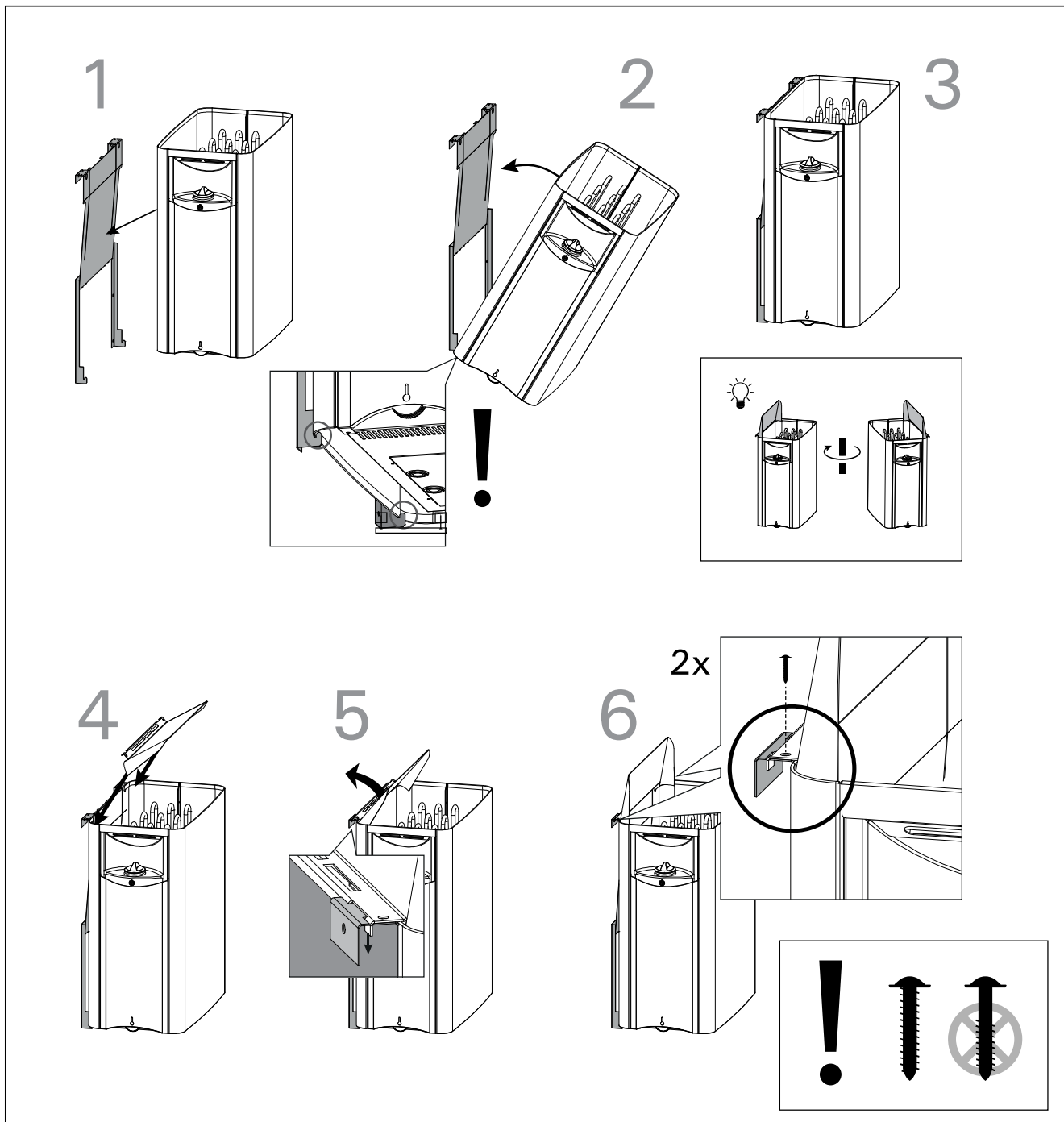
Kuva 9. Kiukaan kiinnitys seinatelineeseen Bild 9. Montering av aggregatet till vaggstallet
