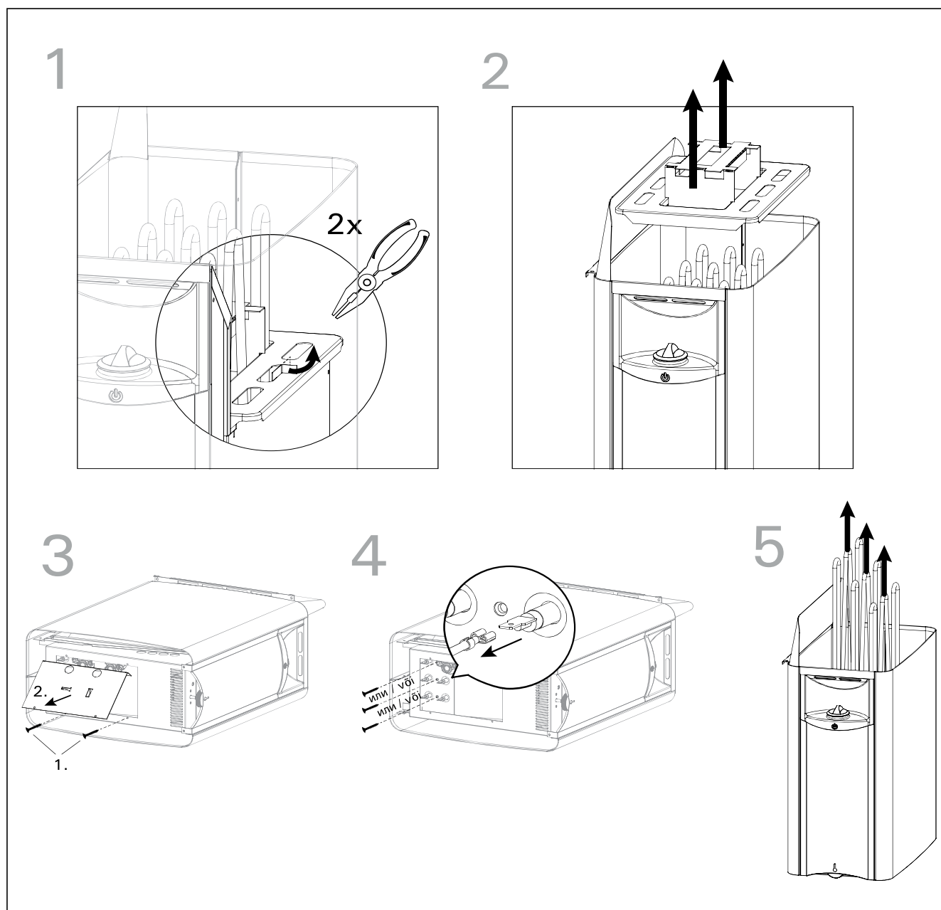
Рисунок 10. Замена нагревательных элементов Joonis 10. Kuttekehade vahetamine
