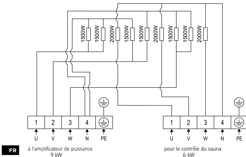
Figure 8. Schéma de câblage CR150E
