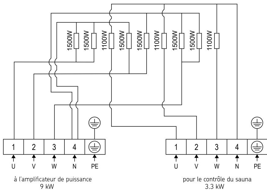
Figure 7. Schéma de câblage CR120E
