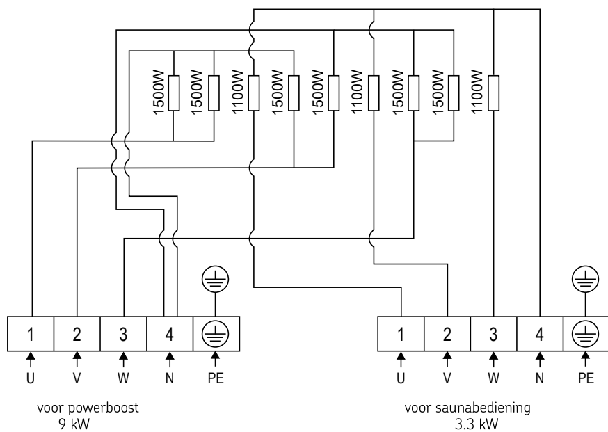
Figuur 7. Aansluitschema CR120E
