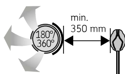
10. attēls. Minimālais attālums no gaisa padeves lūkas līdz temperatūras sensoram
