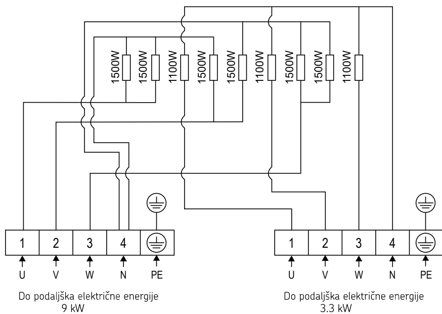
Slika 7. Shema ožičenja CR120E
