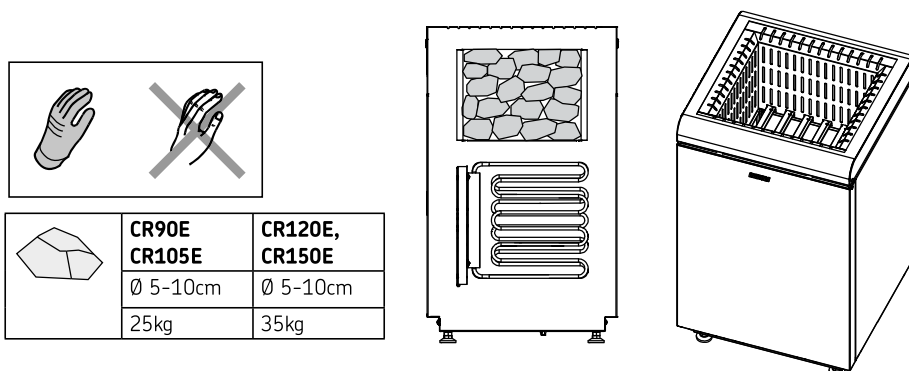
Figuur 8. Saunastenen plaatsen
