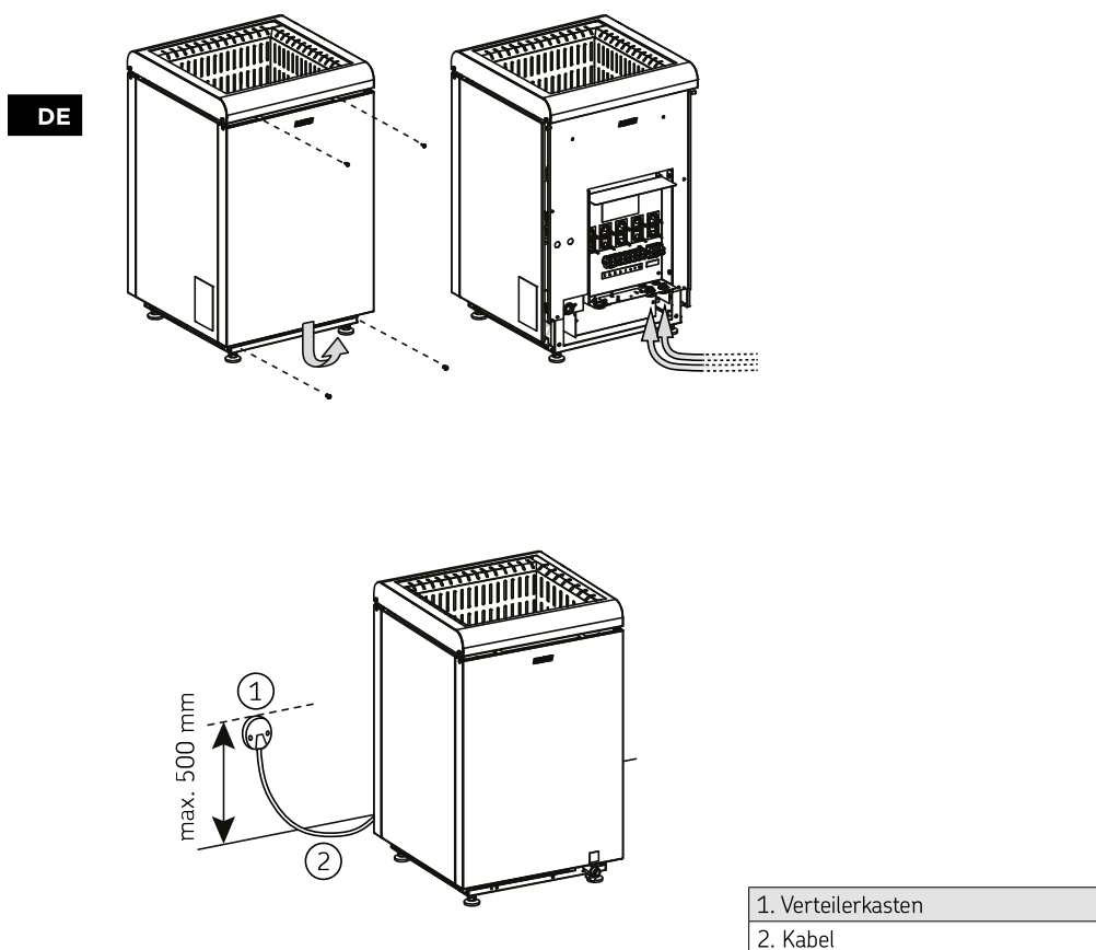
Abbildung 4. Elektroanschlüsse
