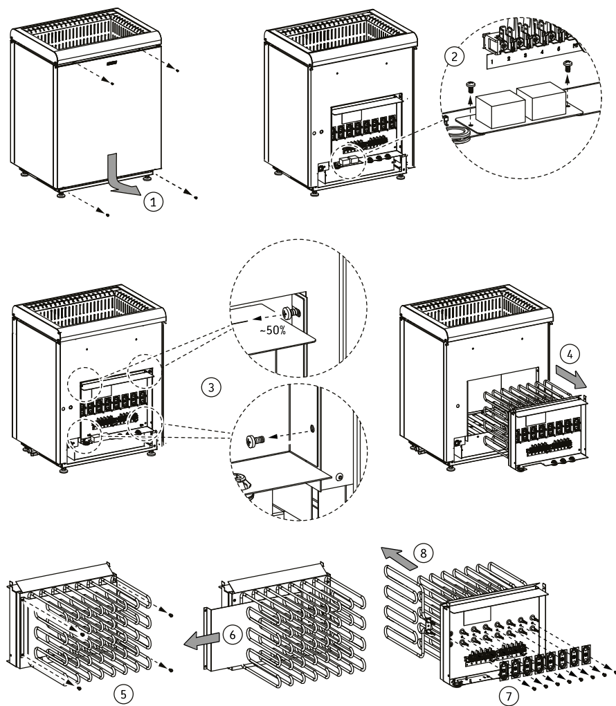
11 pav. Kaitintuvų keitimas
