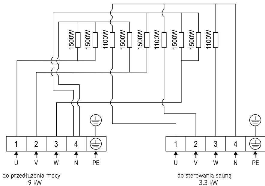
Rysunek 7. Schemat połączeń CR120E
