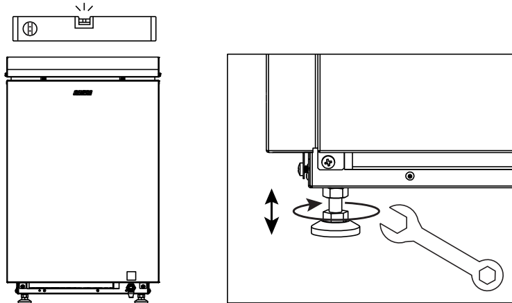
Bild 2. Installation av bastuaggregat
