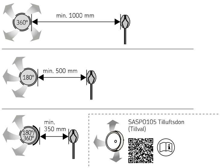
Bild 10. Minimiavstånd mellan tilluftsventil och temperaturgivare.
