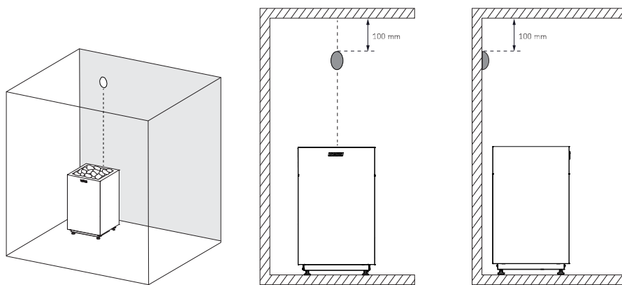
3a pav. Šilumos jutiklio montavimas ant sienos
