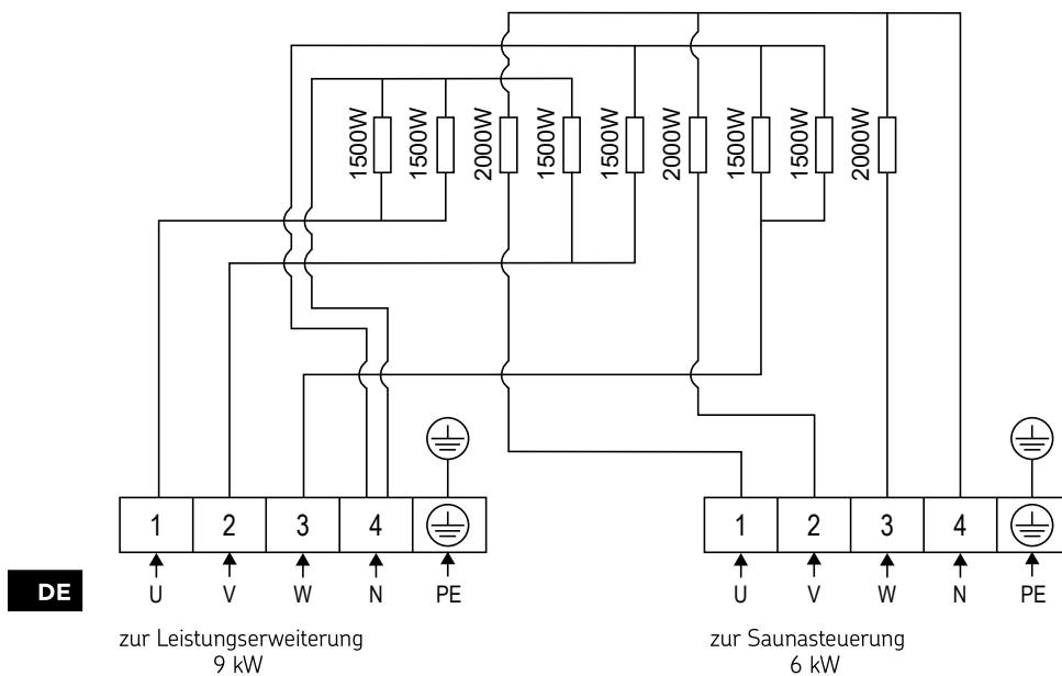
Abbildung 8. Verdrahtungsschema CR150E
