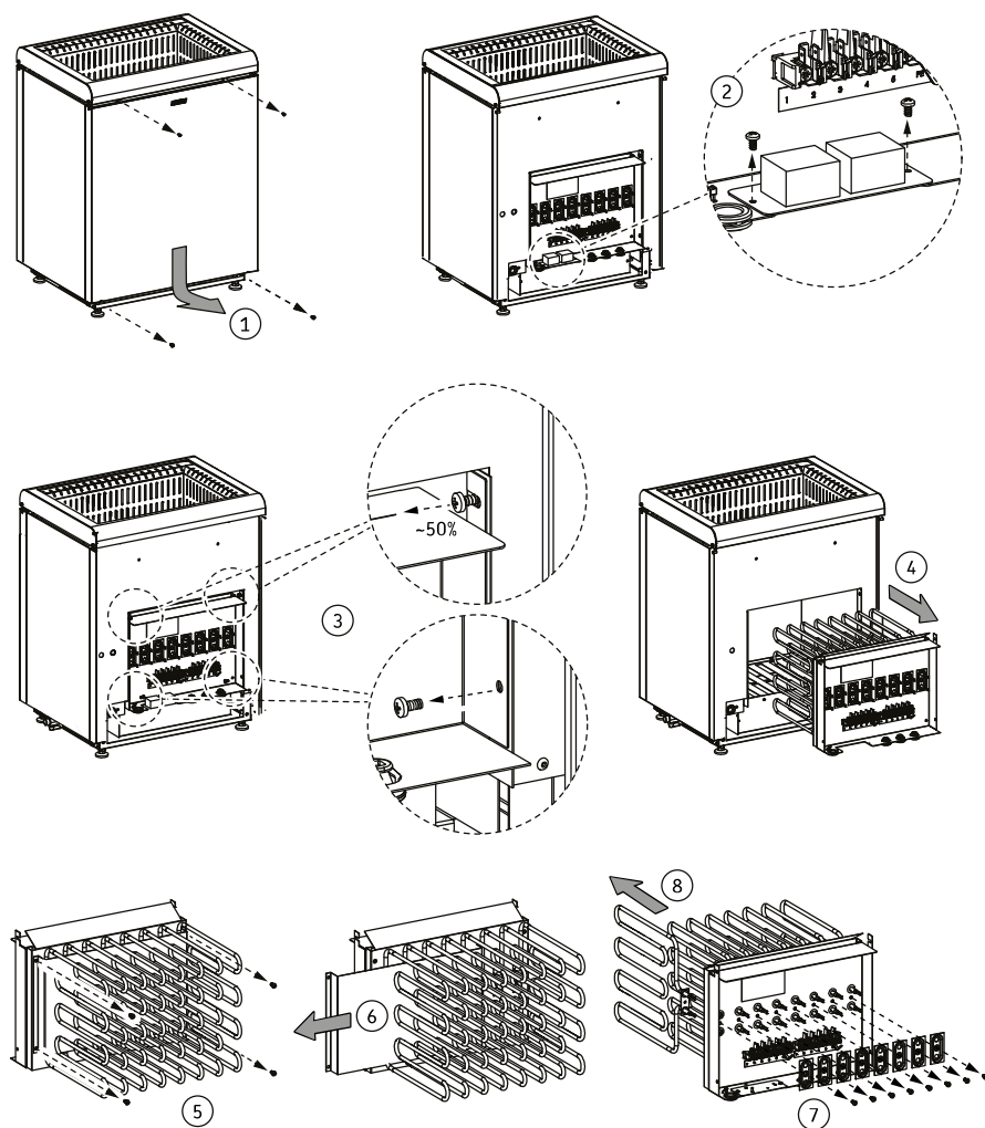
Kuva 11. Vastusten vaihtaminen
