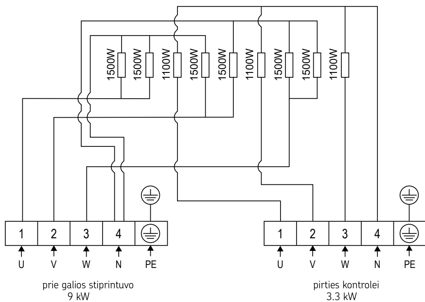
7 pav. Laidų prijungimo schema CR120E
