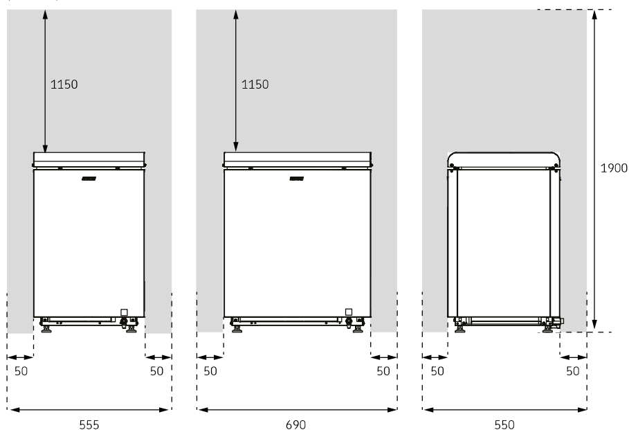
Рисунок 1. Безопасное расстояние
