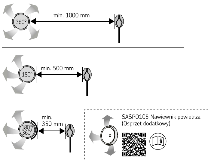
Rysunek 10. Minimalna odległość otworu wentylacyjnego od czujnika.
