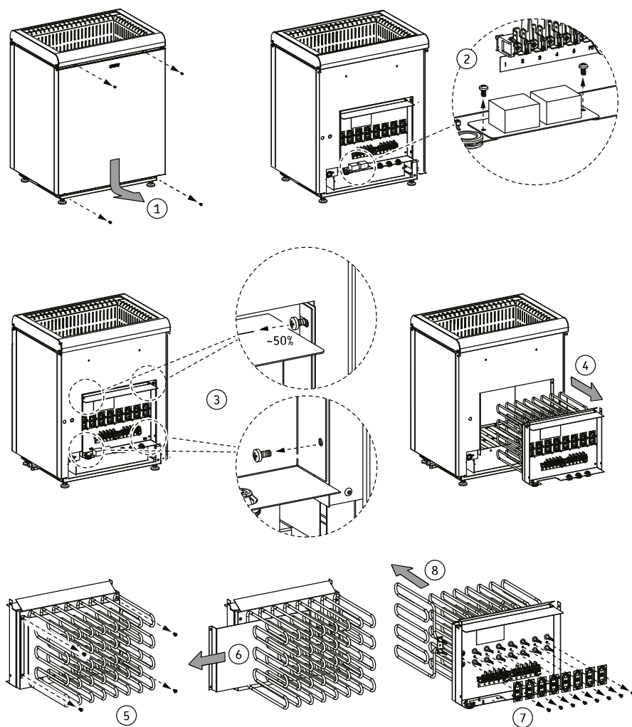
Bild 11. Byta värmeelement
