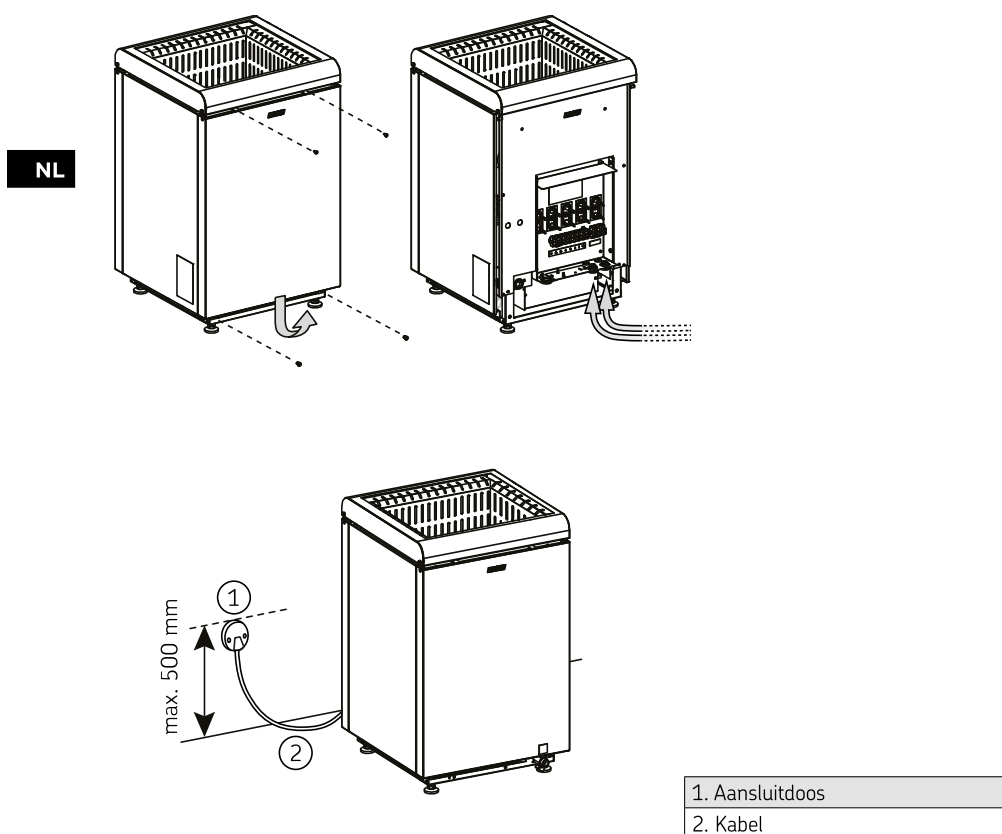
Figuur 4. Elektrische aansluitingen
