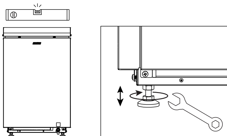
Slika 2. Namestitev grelca za savno
