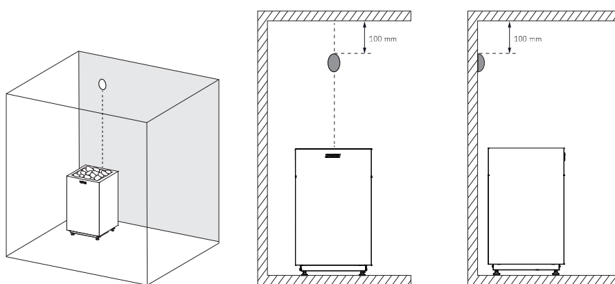
Figura 3a. Installazione del sensore di calore sulla parete
