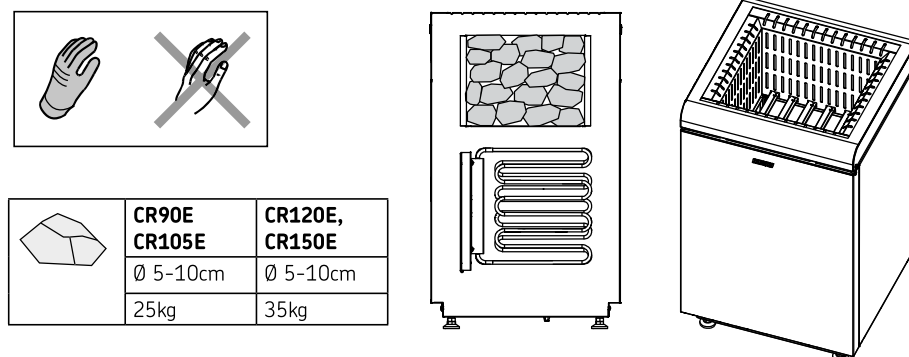
Figure 9. Placement des pierres de poêle
