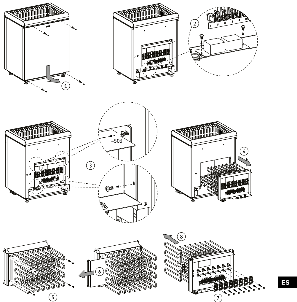
Figura 11. Sustitución de los elementos calefactores
