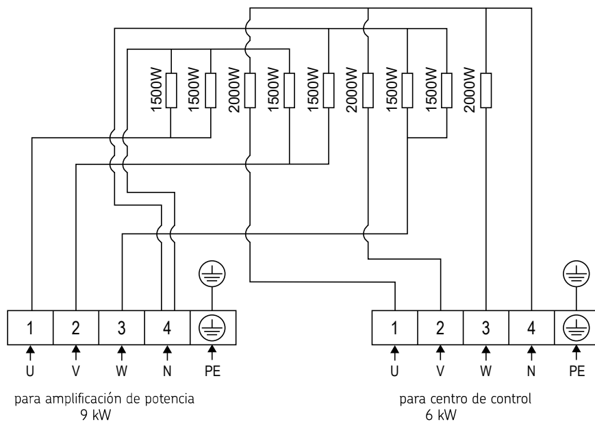
Figura 8. Esquema eléctrico CR150E
