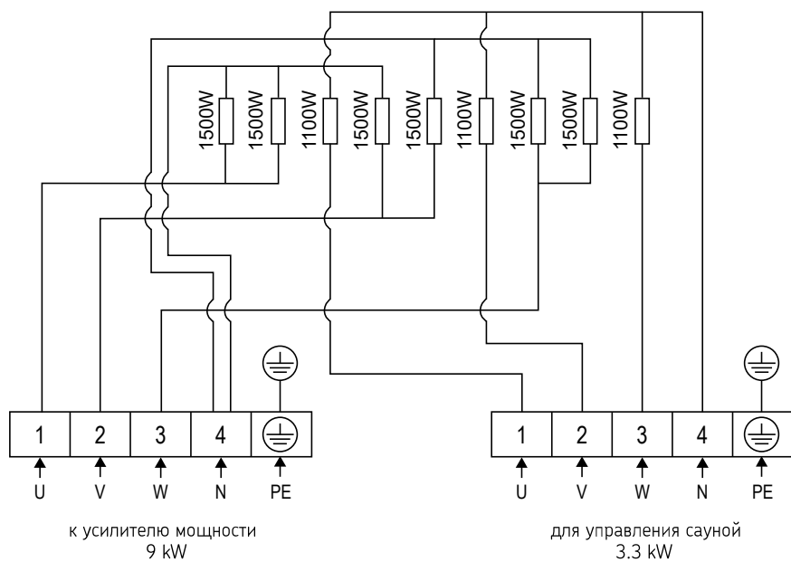
Рисунок 7. Электрическая схема CR120E
