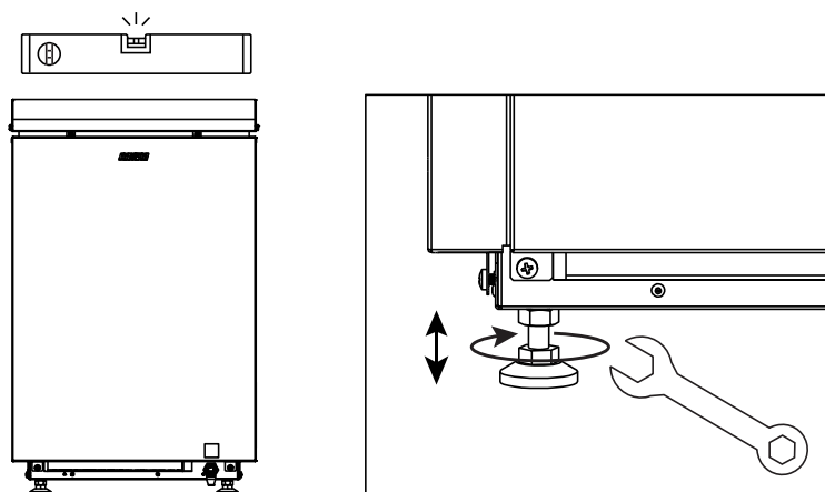
Figuur 2. Installatie saunakachel
