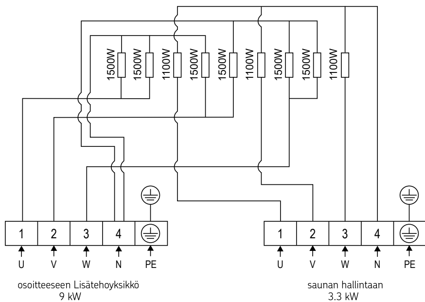
Kuva 7. Kytentäkaavio CR120E
