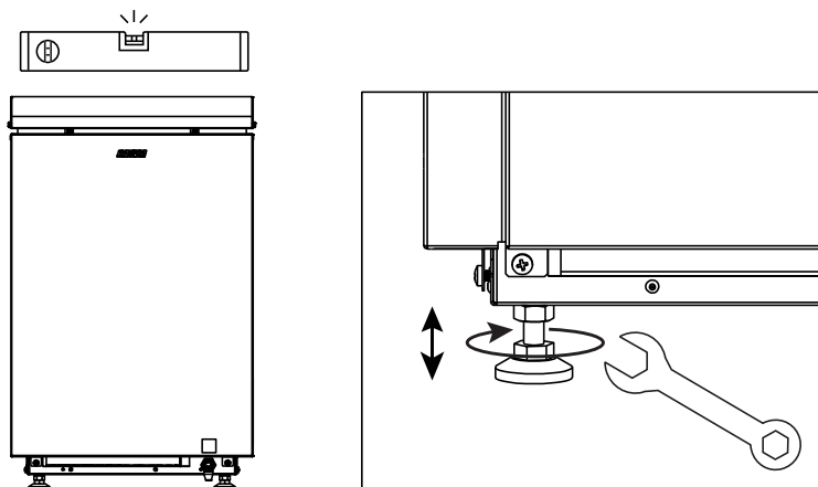
Kuva 2. Kiukaan asennus
