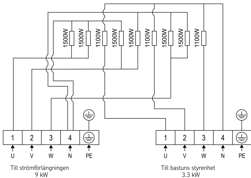
Bild 6. Kopplingsschema CR120E
