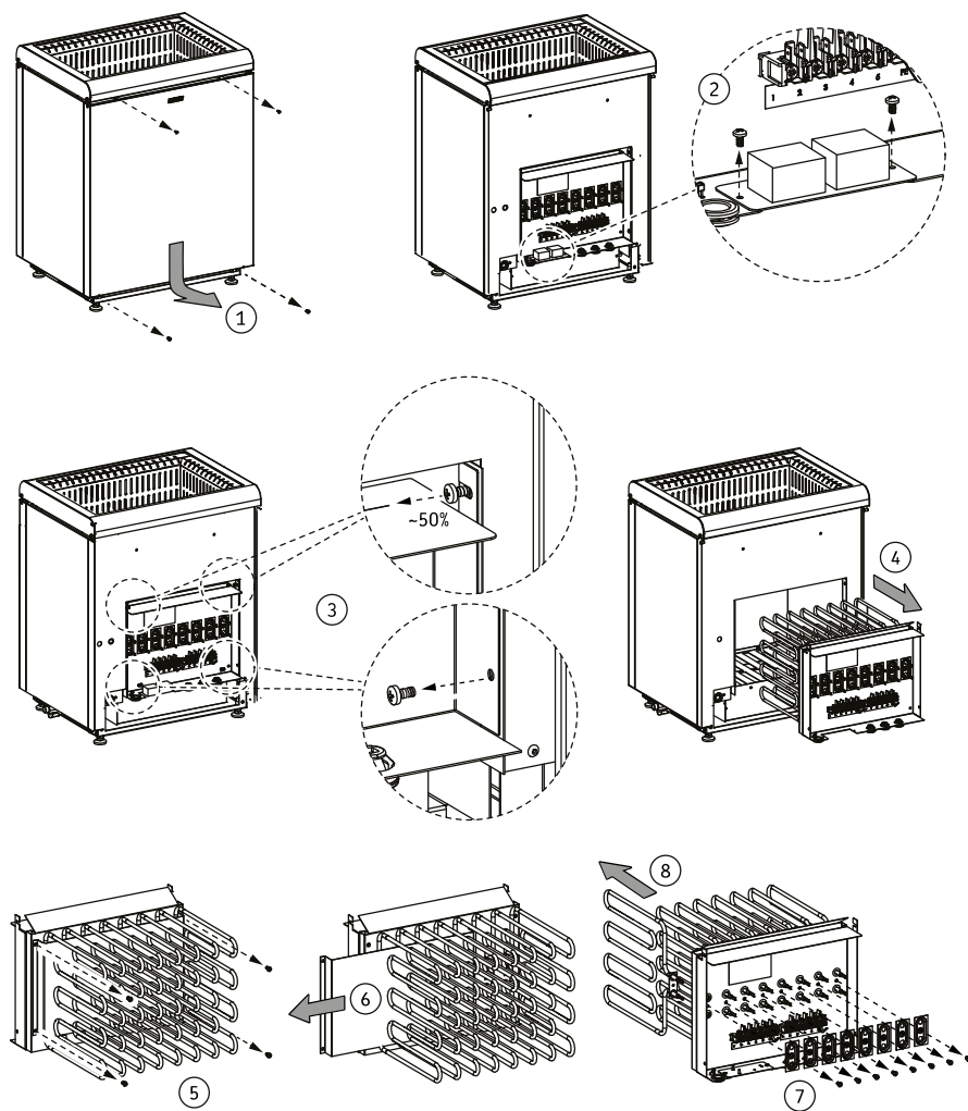
11. attēls. Sildelementu maiņa
