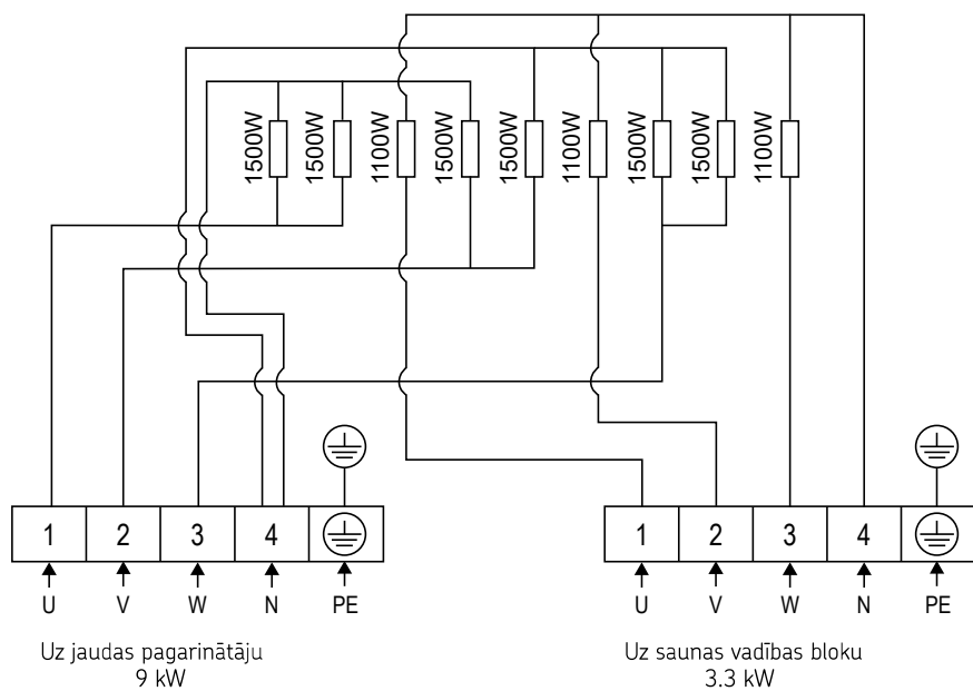
7. attēls. Elektroinstalācijas shēma CR120E
