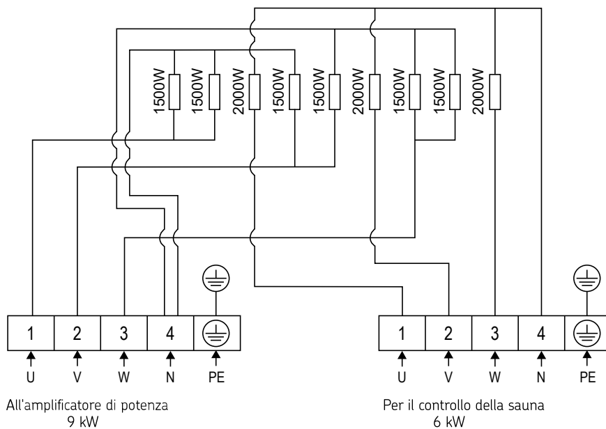
Figura 8. Schema elettrico CR150E
