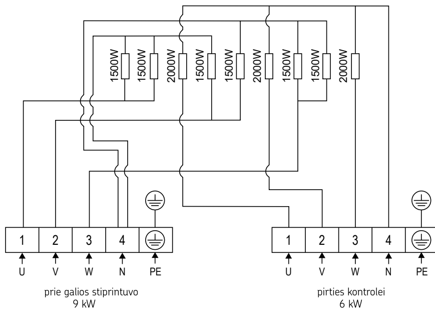
8 pav. Laidų prijungimo schema CR150E
