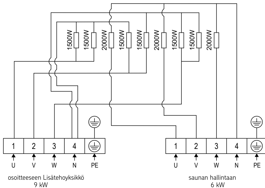
Kuva 8. Kytentäkaavio CR150E
