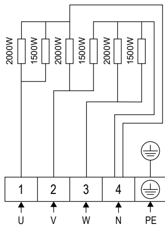
Figura 6. Schema elettrico CR105E
