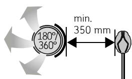
10 pav. Mažiausias atstumas nuo tiekiamo oro ventiliacijos angos iki temperatūros jutiklio
