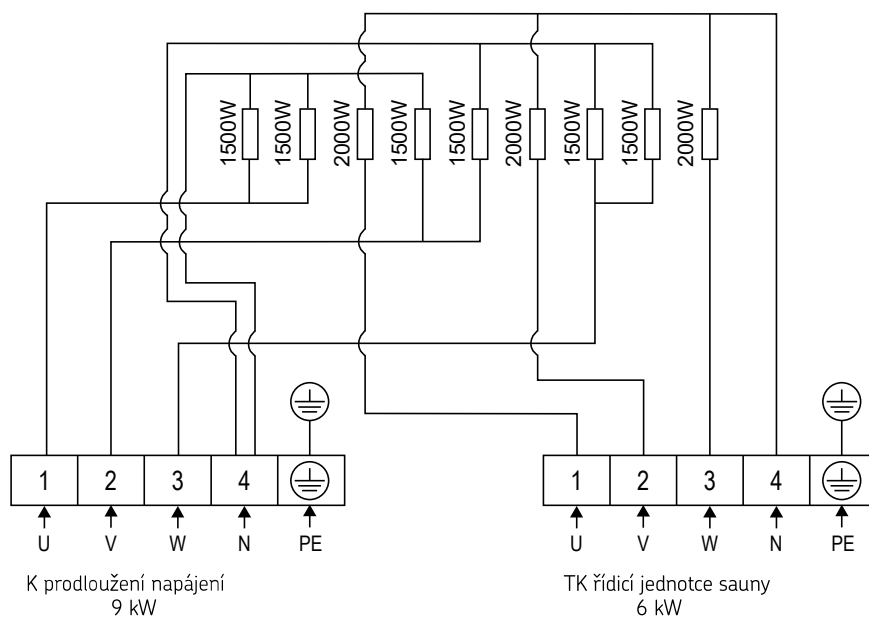
Obrázek 8. Schéma zapojení CR150E
