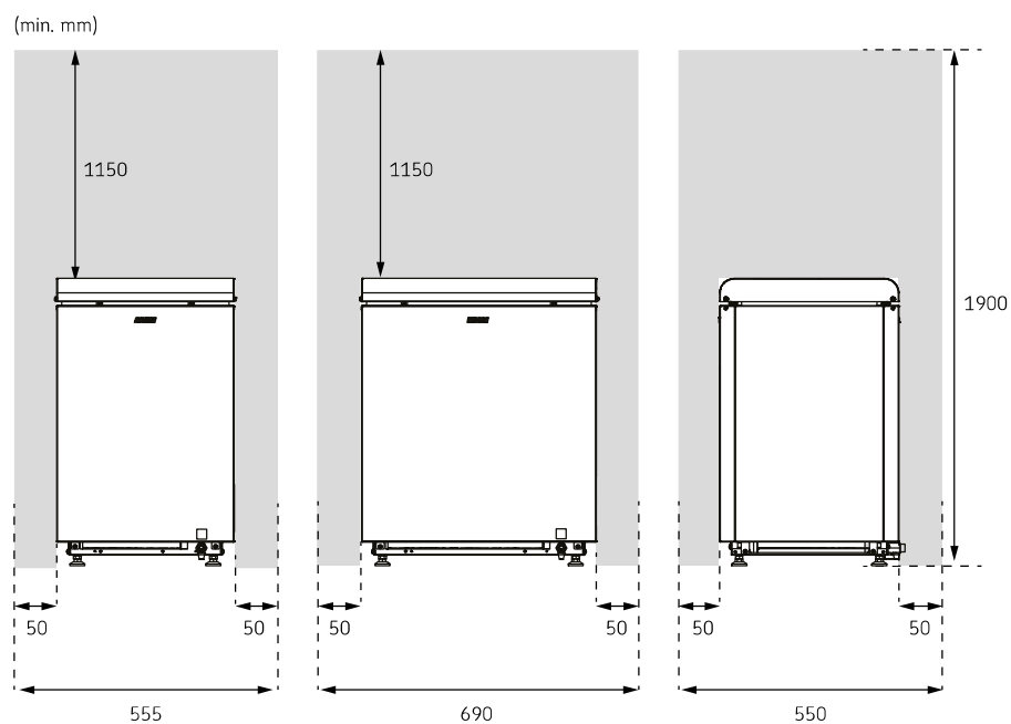
Figura 1. Distancias de seguridad
