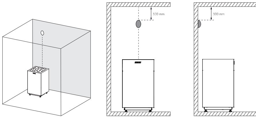
Kuva 3a. Lämpöanturin asentaminen seinälle
