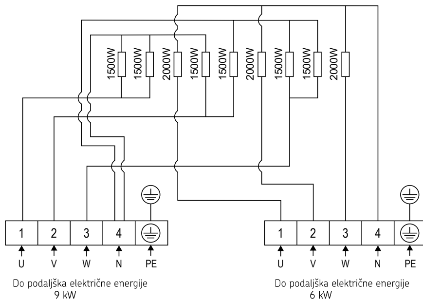
Slika 8. Shema ožičenja CR150E
