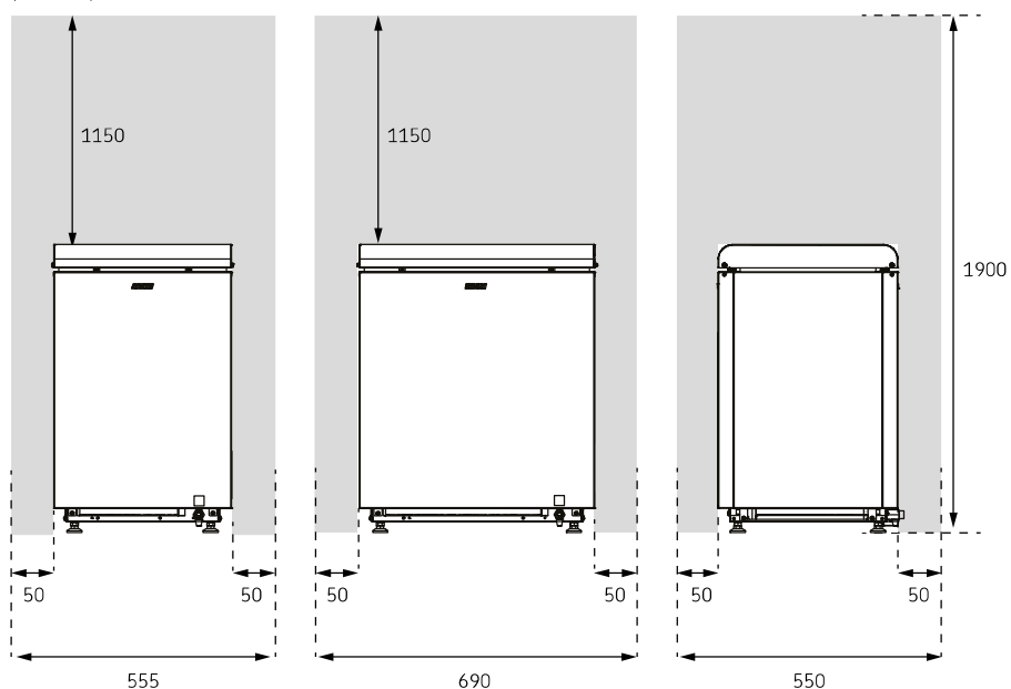
Figuur 1. Veiligheidsafstanden
