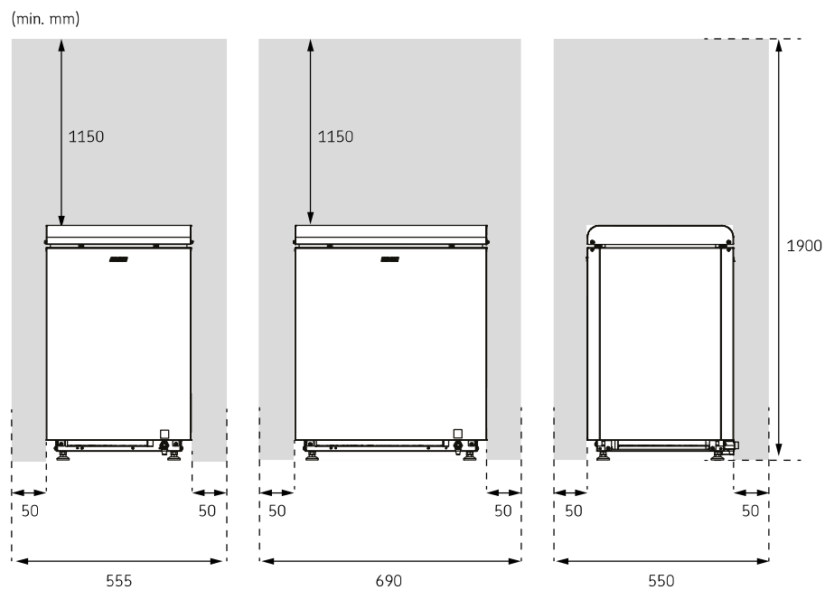
Bild 1. Säkerhetsavstånd
