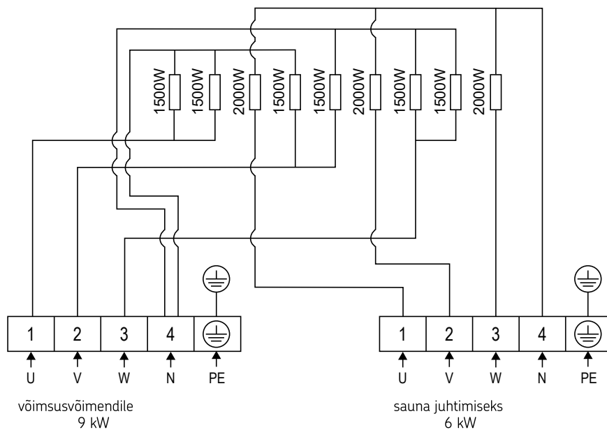
Joonis 8. Elektriskeem CR150E
