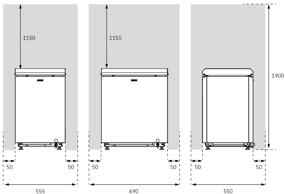
Obrázek 1 Bezpečnostní vzdálenosti
