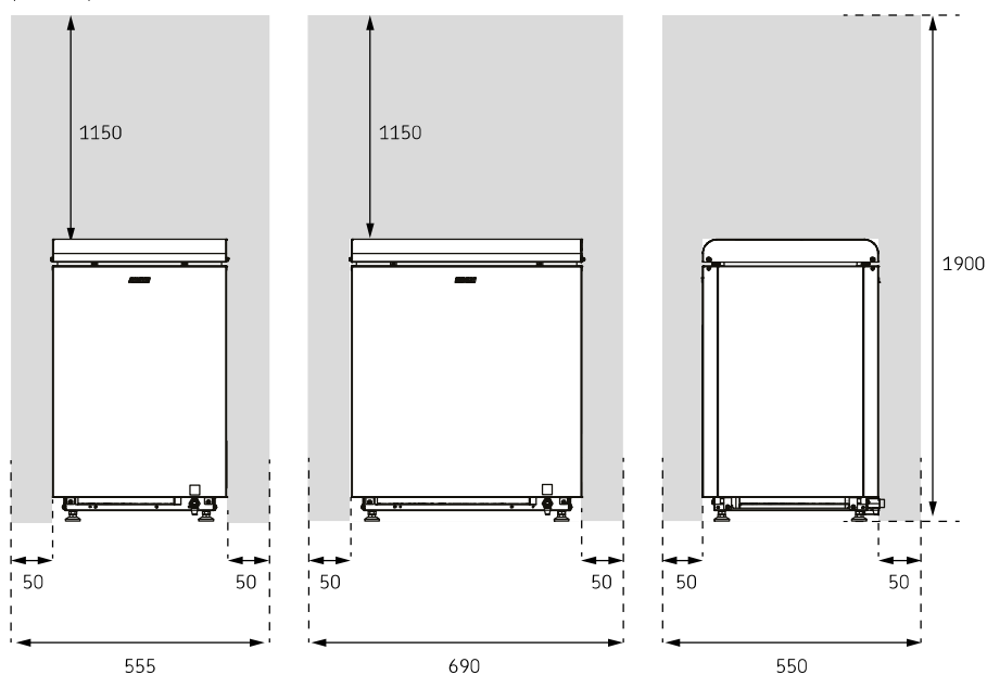
Kuva 1. Suojaetäisyydet
