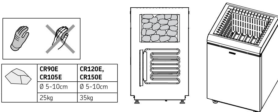
Abbildung 9. Befüllung der Steinkammer
