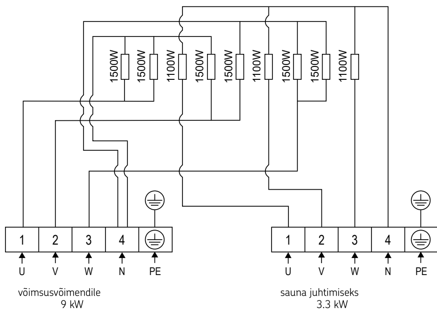
Joonis 7. Elektriskeem CR120E
