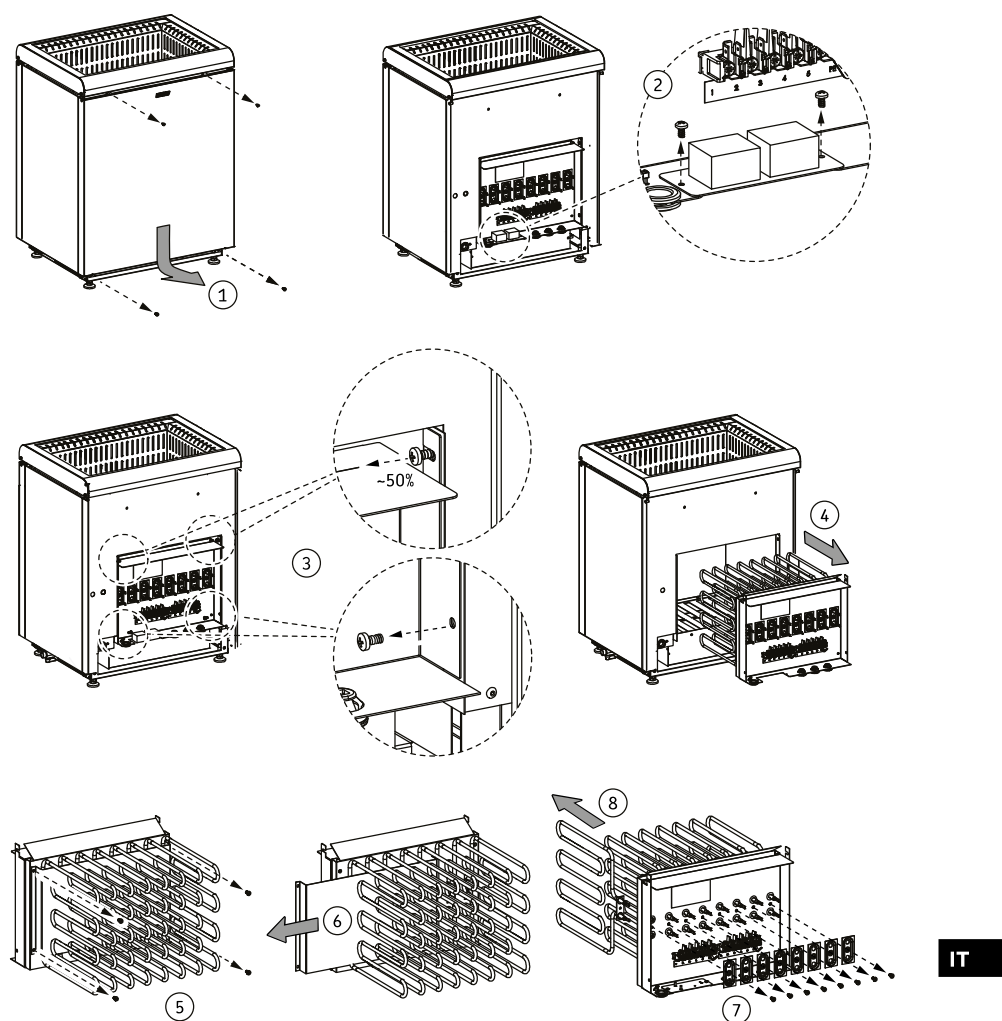
Figura 11. Sostituzione delle resistenze
