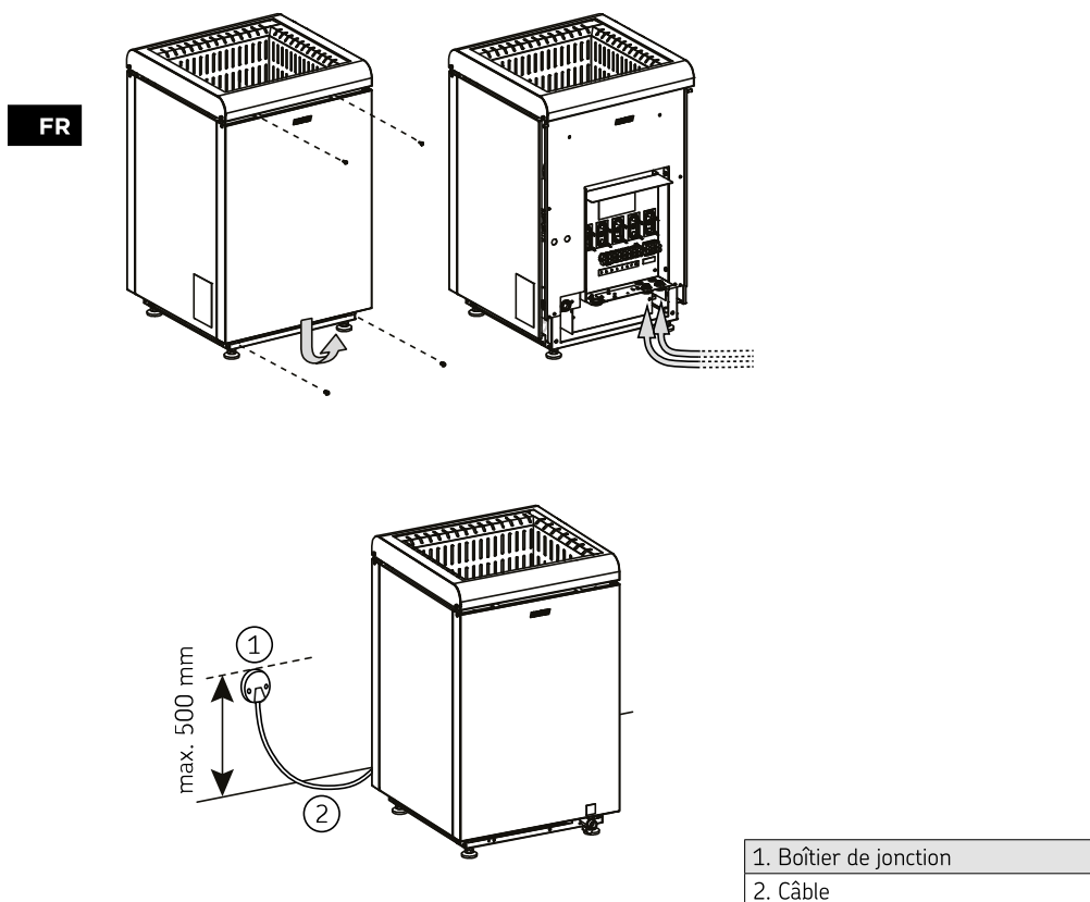
Figure 4. Raccordements électriques
