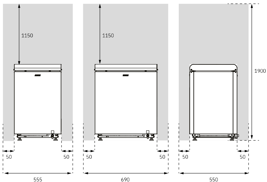
Slika 1. Varnostne razdalje
