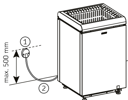
Obrázek 4 Elektrické připojení
