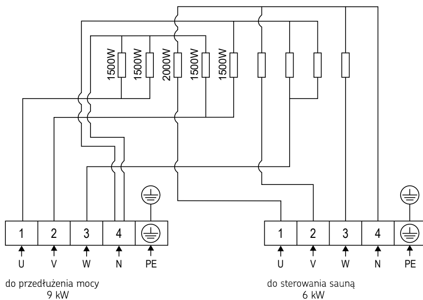
Rysunek 8. Schemat połączeń CR150E
