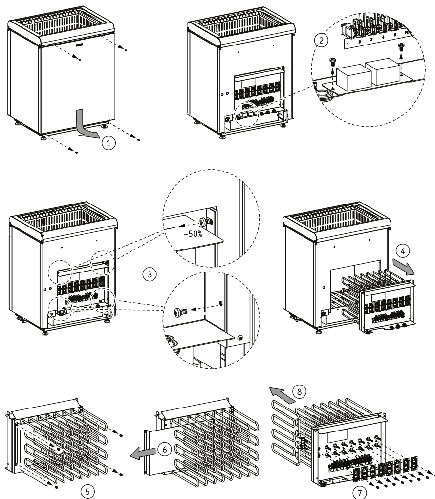
Obrázek 11 Výměna topných těles
