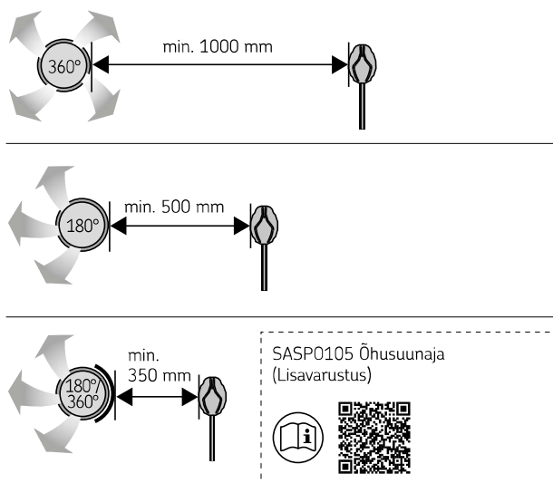
Joonis 10. Ventilatsiooniava minimaalne kaugus andurist.
