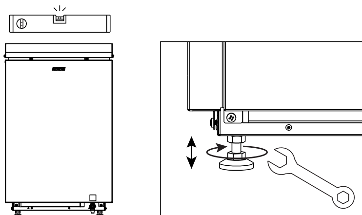
Joonis 2. Kerise paigaldamine
