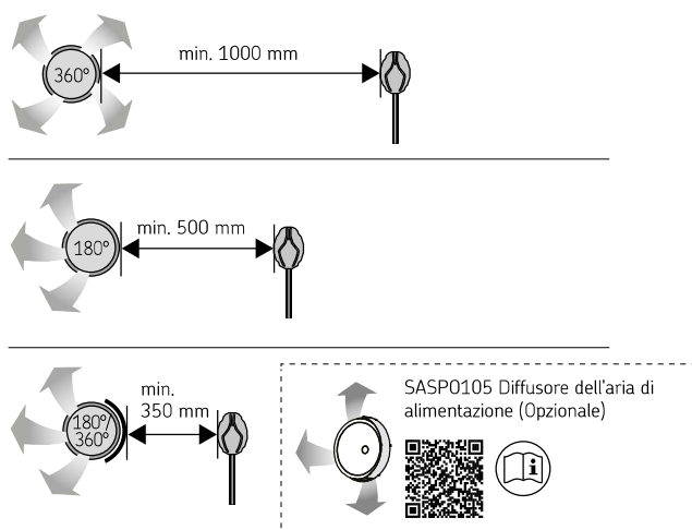
Figura 10. Distanza minima tra lo sfianto dell'aria di alimentazione e il sensore di temperatura.
