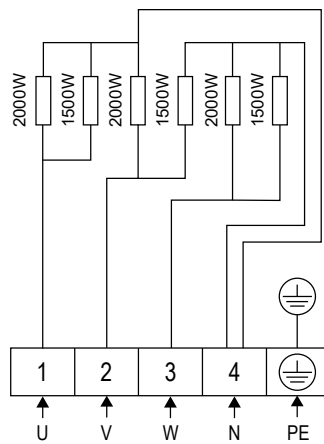
Abbildung 6. Verdrahtungsschema CR105E
