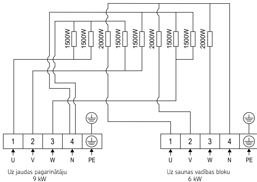
8. attēls. Elektroinstalācijas shēma CR150E
