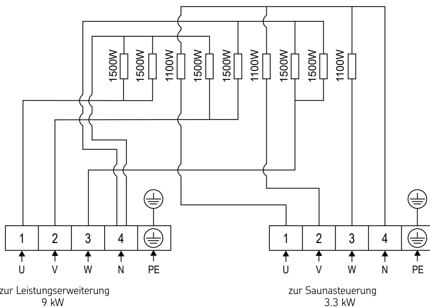
Abbildung 7. Verdrahtungsschema CR120E
