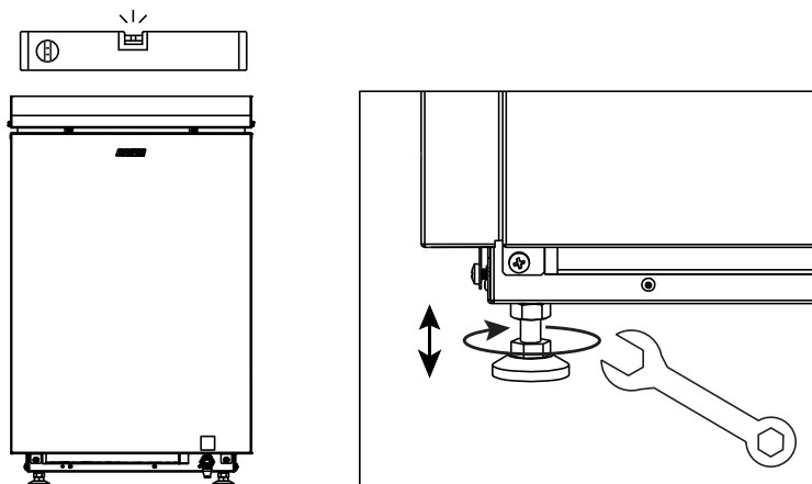
2. attēls. Pirts sildītāja uzstādīšana
