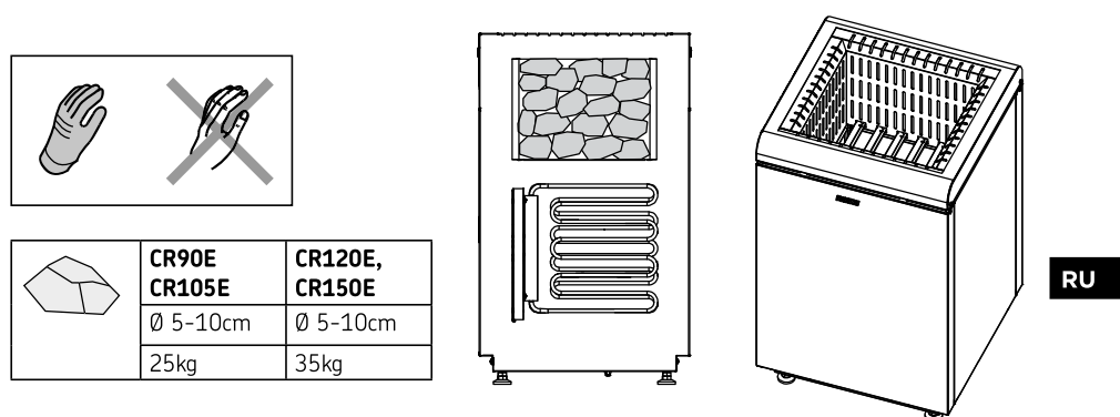
Рисунок 9. Наполнение каменки камнями
