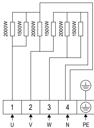
Joonis 6. Elektriskeem CR105E
