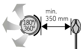
Obrázek 10 Minimální vzdálenost od větracího otvoru přívodu vzduchu k teplotnímu senzoru
