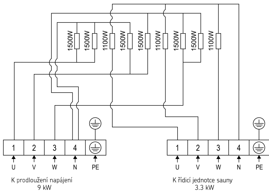
Obrázek 7. Schéma zapojení CR120E
