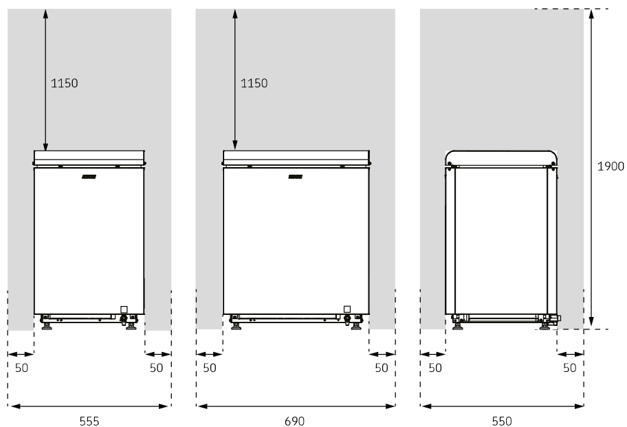
Joonis 1. Ohutuskaugused
