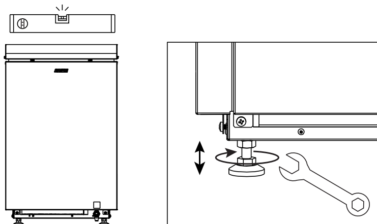
2 pav. Saunos krosnelės įrengimas
