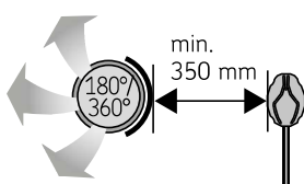
Kuva 10. Tuloilmaventtiilin vähimmäisetäisyys lämpötila-anturiin
