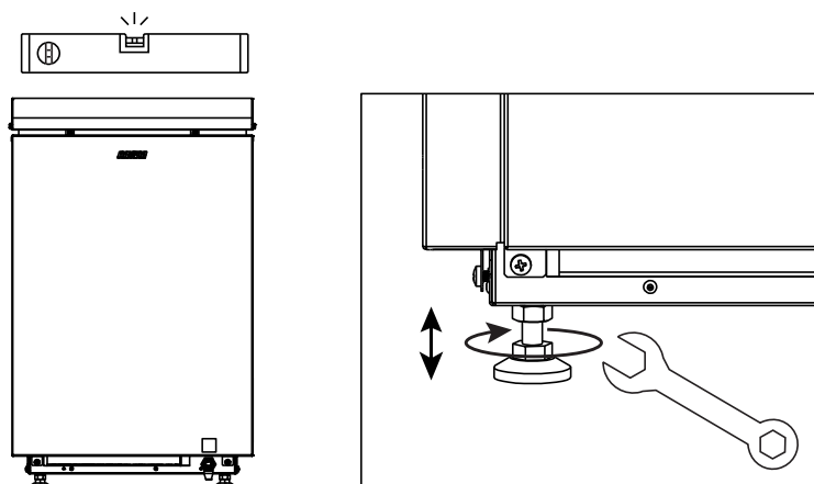
Figura 2. Installazione della stufa per sauna
