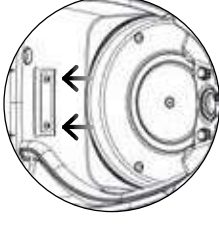
Montage an der Wand
