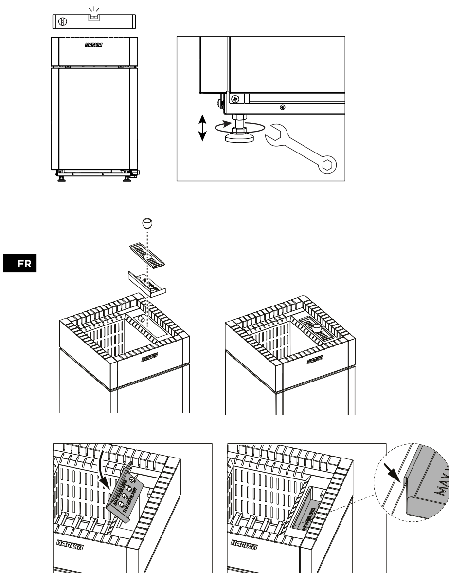
Figure 2. Installation du poêle pour sauna
