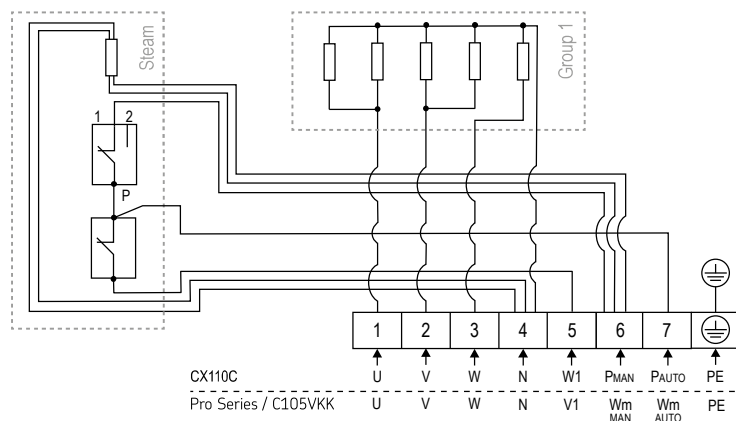
Slika 5. Shema ožičenja QU100S
