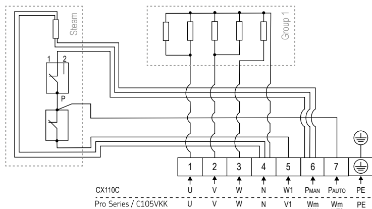
Joonis 5. Elektriskeem QU100S
