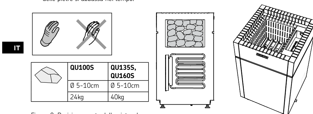
Figura 8. Posizionamento delle pietre da sauna
