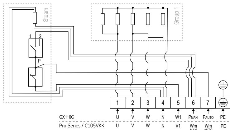
5. attēls. Elektroinstalācijas shēma QU100S
