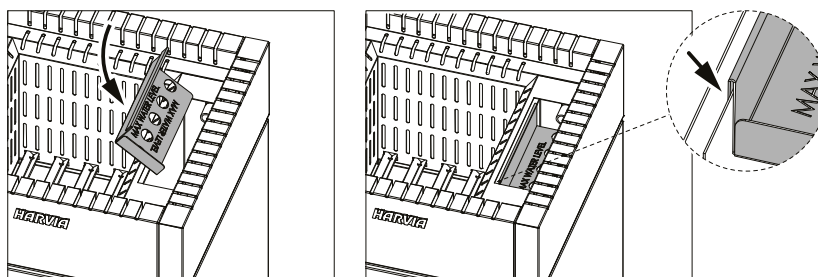
Kuva 2. Kiukaan asennus
