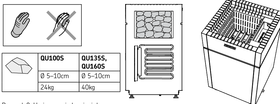
Rysunek 8. Umieszczanie kamieni do sauny
