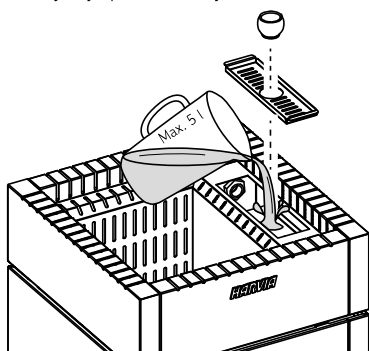
Slika 10. Polnjenje rezervoarja za vodo
