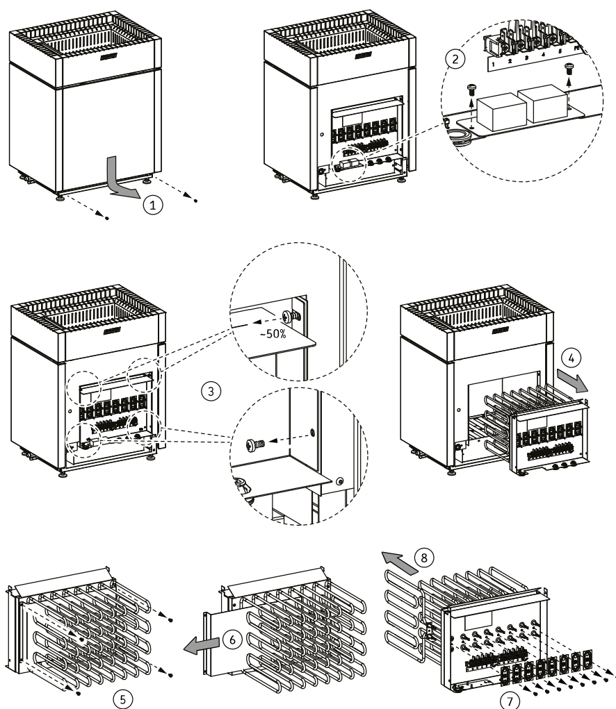
Рисунок 13. Замена нагревательных элементов
