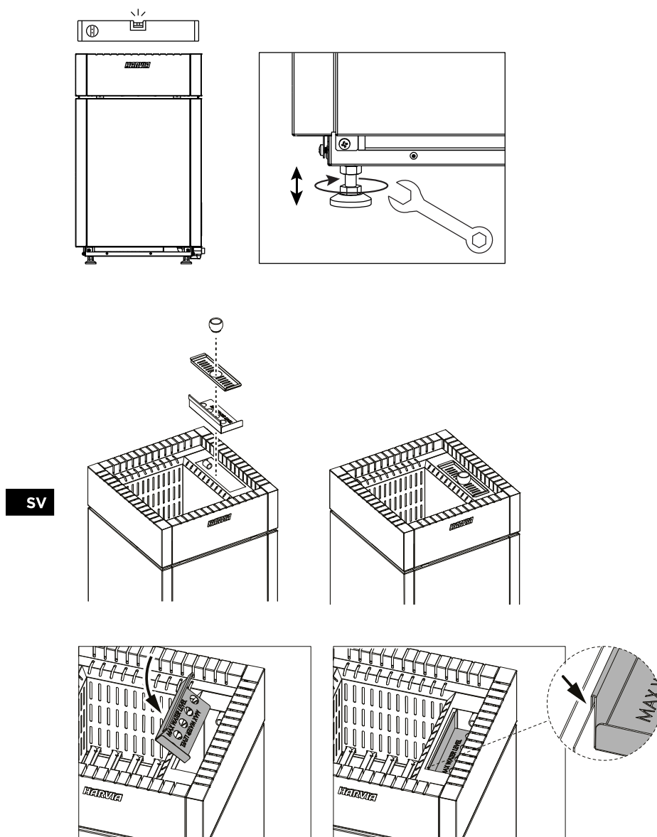
Bild 2. Installation av bastuaggregat
