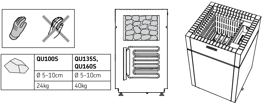
Figure 8. Placement des pierres de poêle
