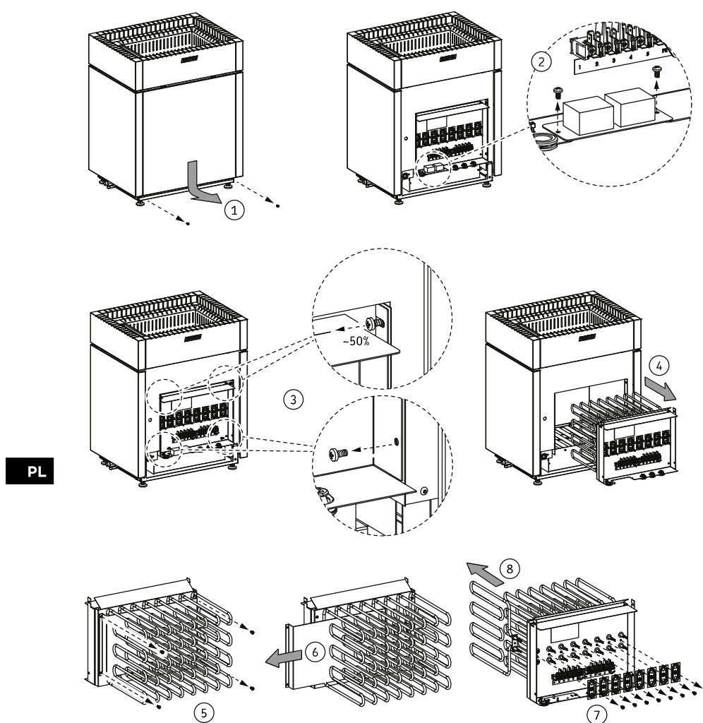
Rysunek 13. Wymiana elementów grzejnych
