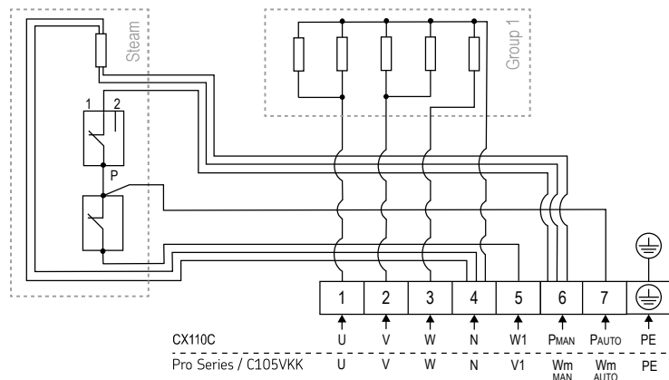
5 pav. Laidų prijungimo schema QU100S
