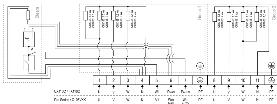
Figuur 6. Aansluitschema QU135S, QU160S
