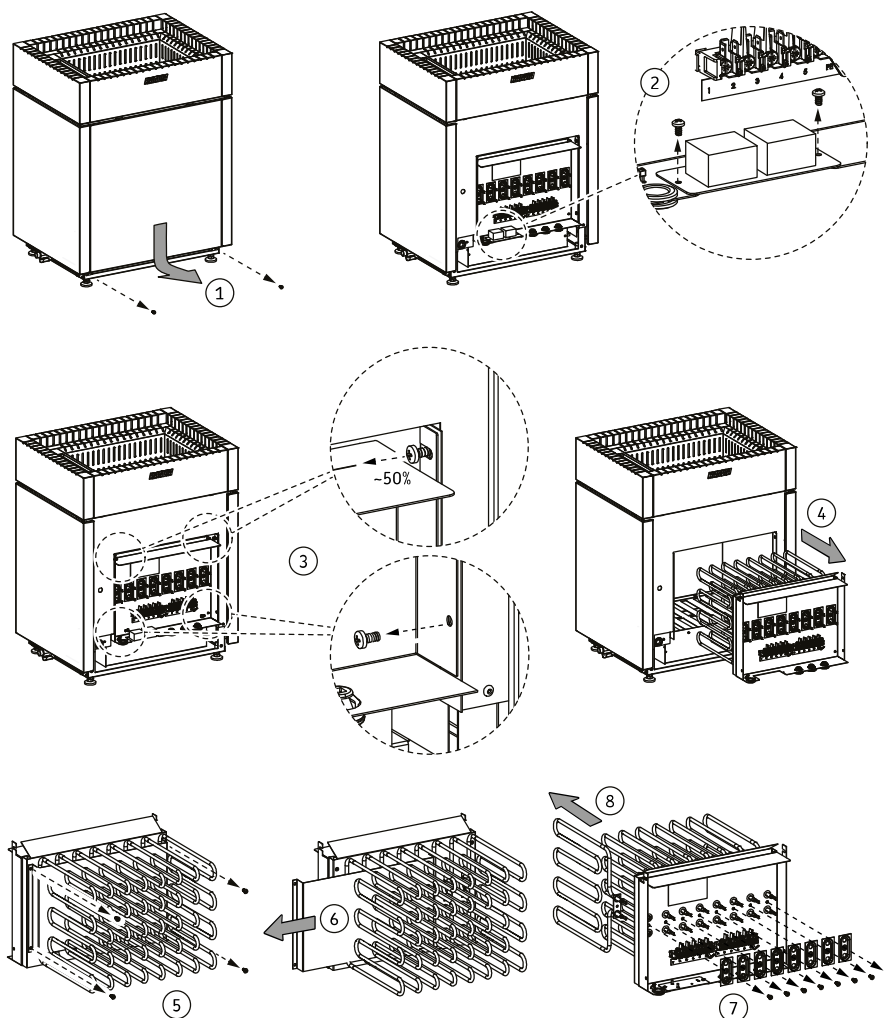
13 pav. Kaitintuvų keitimas
