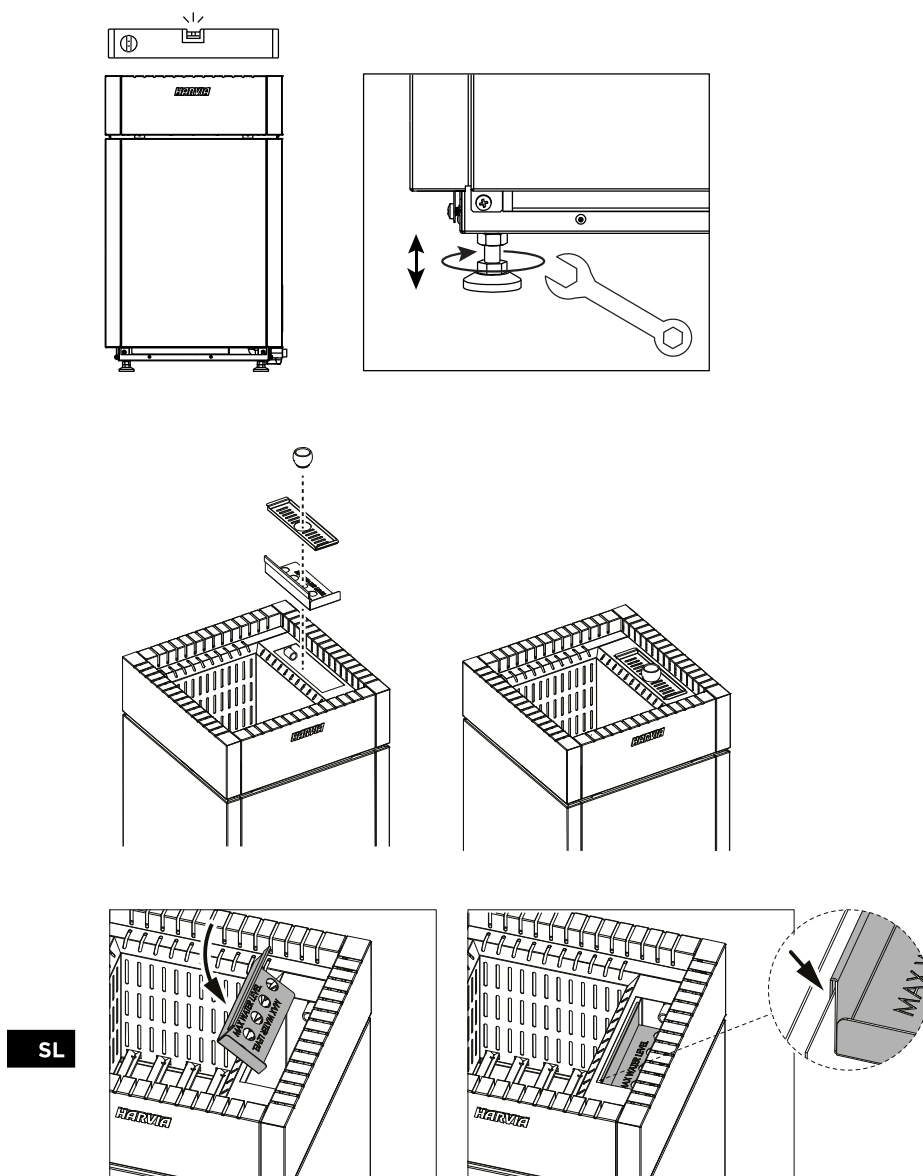
Slika 2. Namestitev grelca za savno
