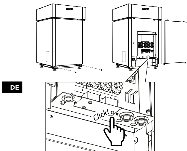
Abbildung 14. Zurücksetzen des Überhitzungsschutzes des Verdampfers
