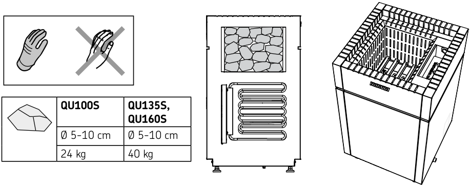
Abbildung 8. Befüllung der Steinkammer
