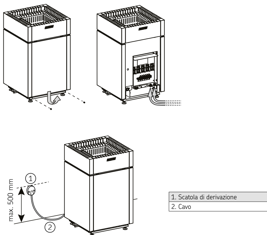
Figura 4. Collegamenti elettrici
