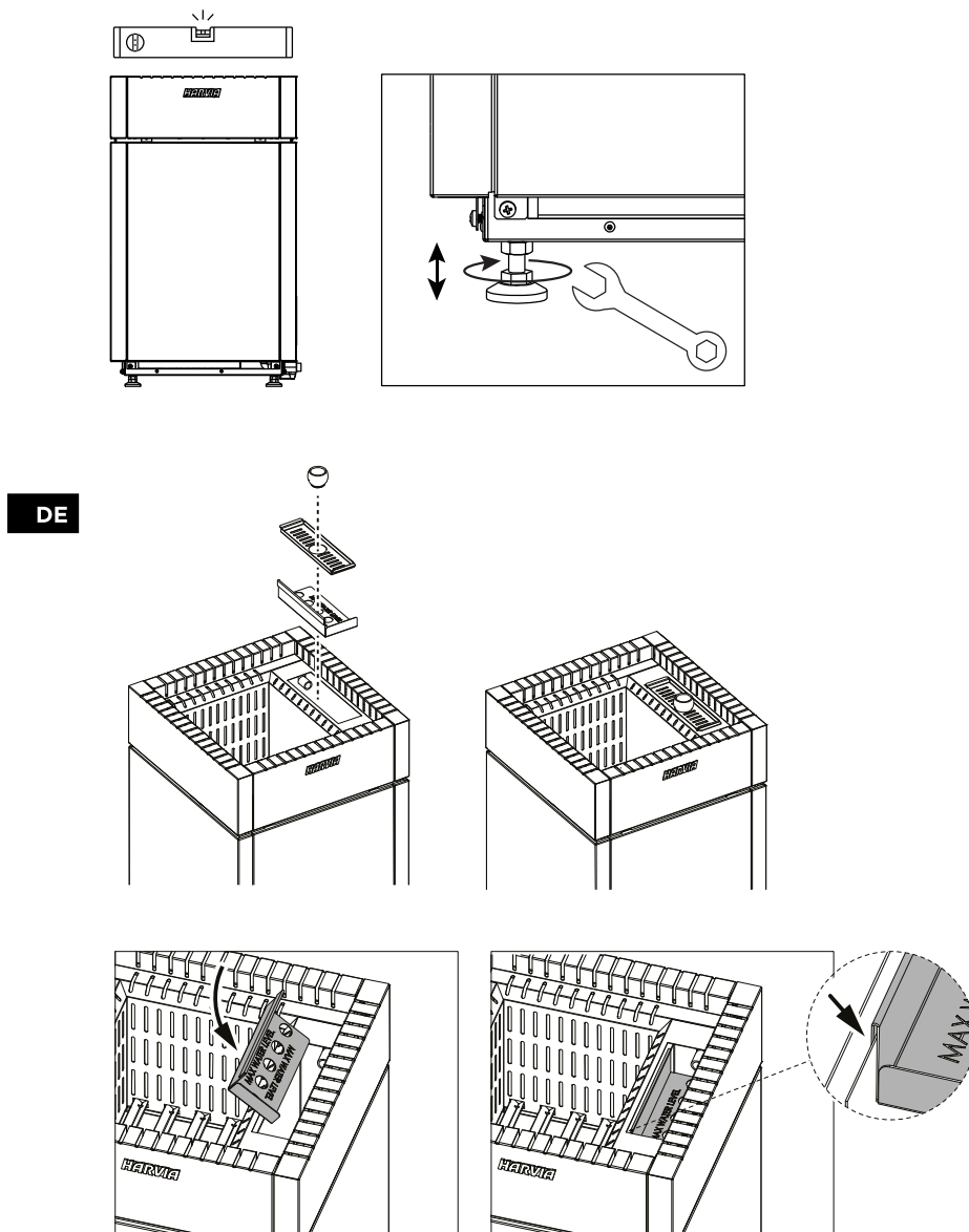
Abbildung 2. Installation eines Saunaofens
