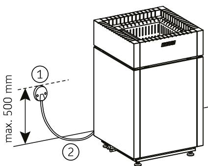
Рисунок 4. Электрические соединения
