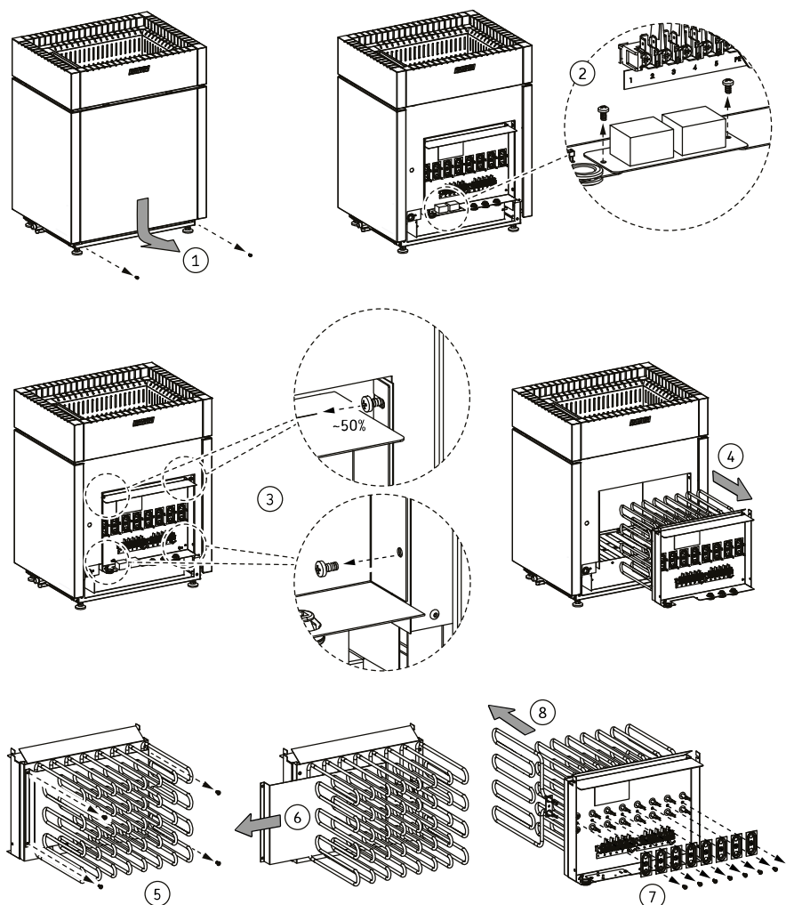
Figura 13. Sustitución de los elementos calefactores
