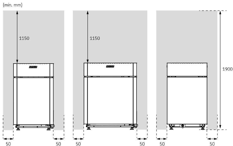
Figura 1. Distanza di sicurezza
