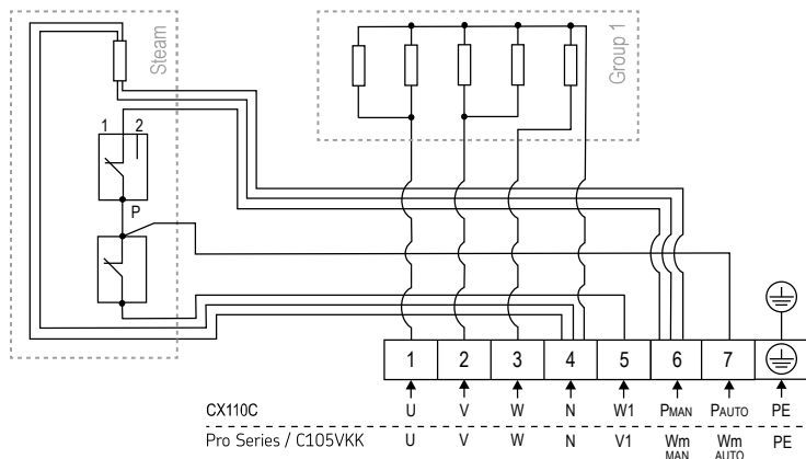
Kuva 5. Kytentäkaavio QU100S
