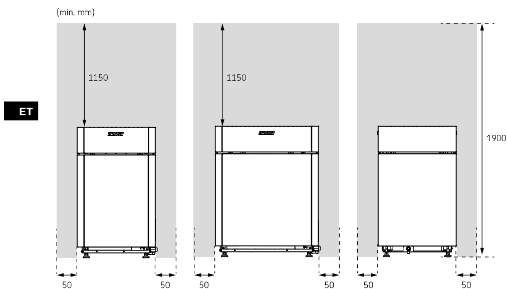
Joonis 1. Ohutuskaugused
