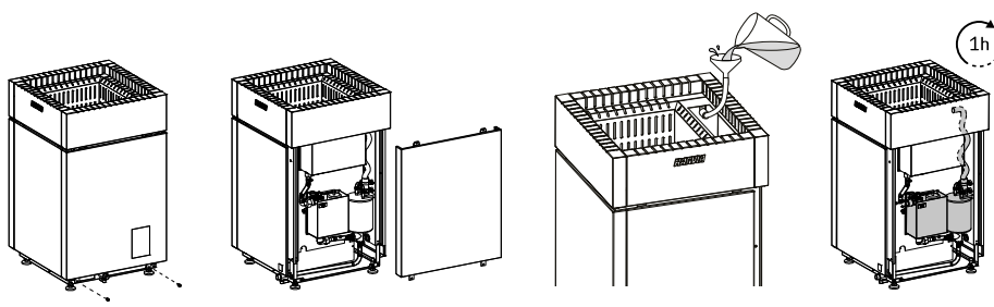
12. attēls. Atkaļķošana ar citronskābes šķīdumu
