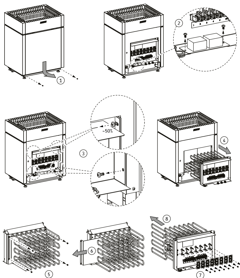
Figure 13. Remplacement des résistances
