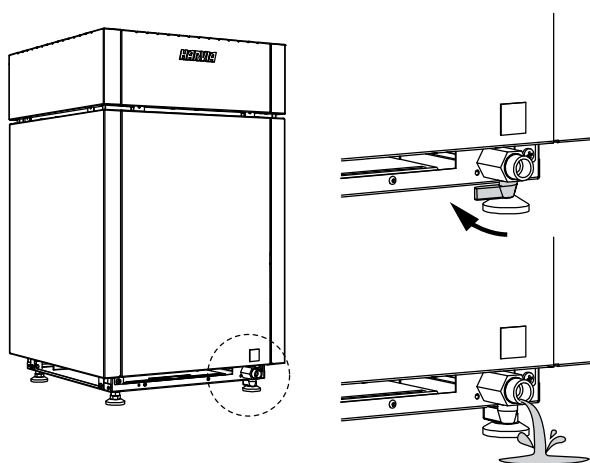
Bild 11. Tömma vattenbehållaren
