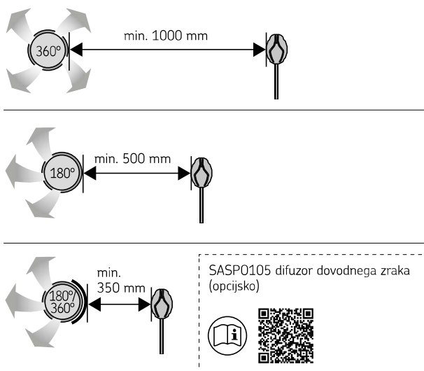
Slika 9. Najmanjša razdalja od zračnika za dovod zraka do senzorja za temperaturo.
