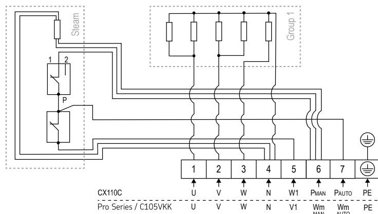
Obrázek 5 Schéma zapojení QU100S
