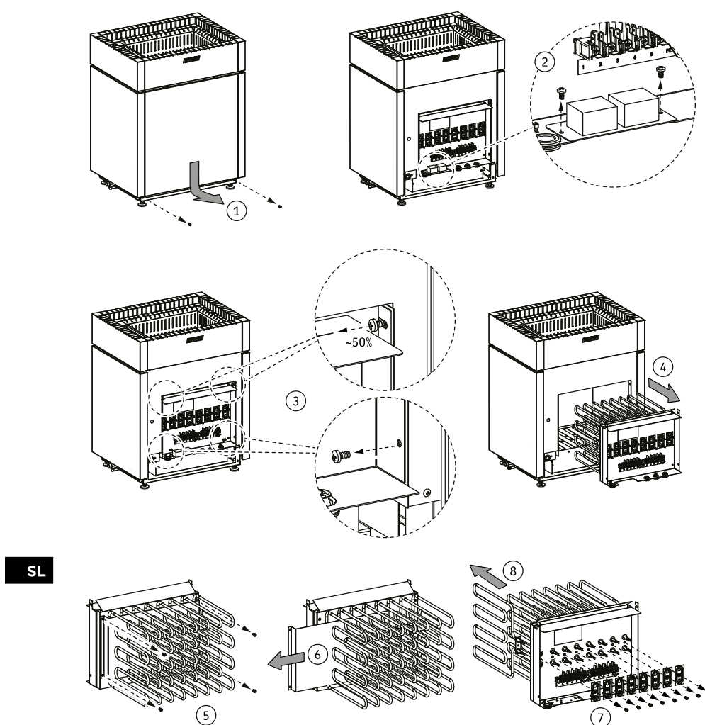
Slika 13. Menjava grelnih elementov
