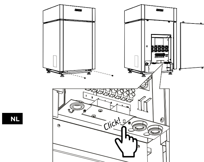
Figuur 14. Reset de beveiliging tegen oververhitting van de stoomgenerator
