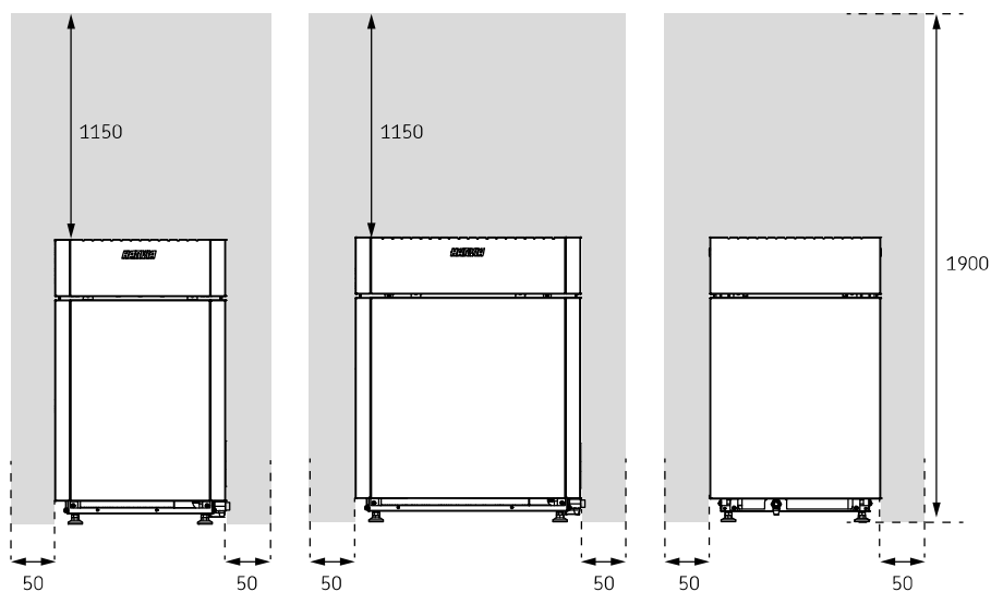
Figuur 1. Veiligheidsafstanden
