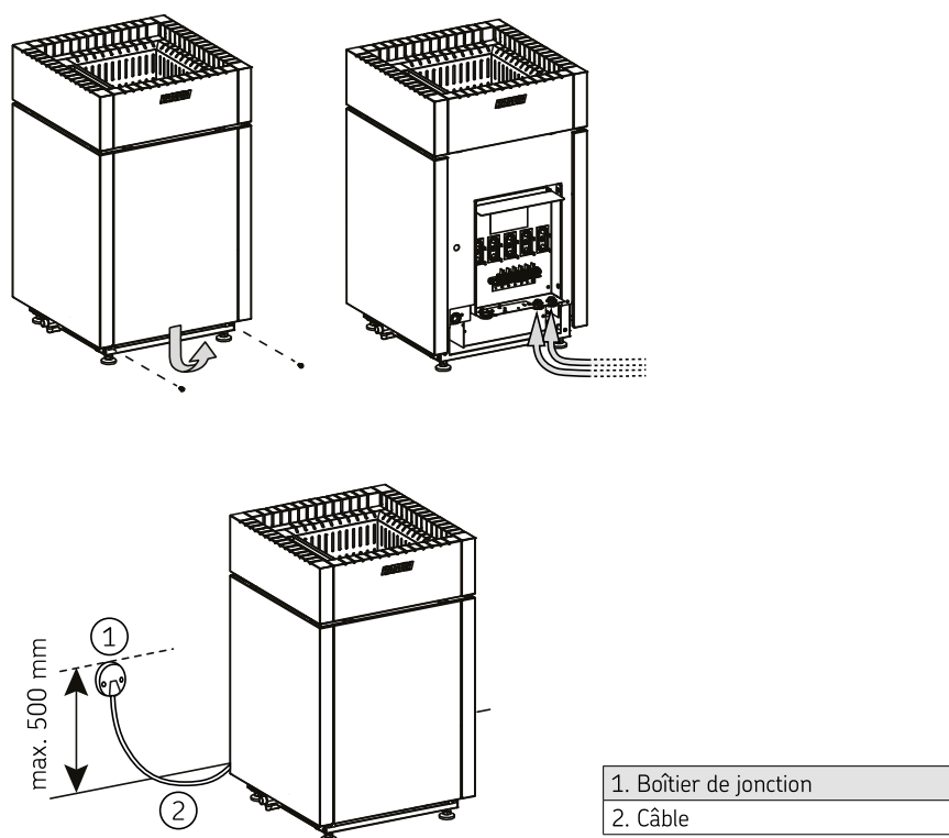
Figure 4. Raccordements électriques
