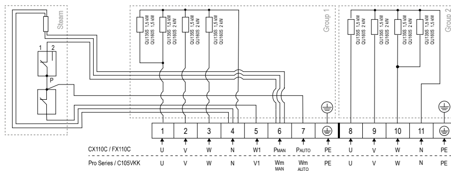
Joonis 6. Elektriskeem QU135S, QU160S
