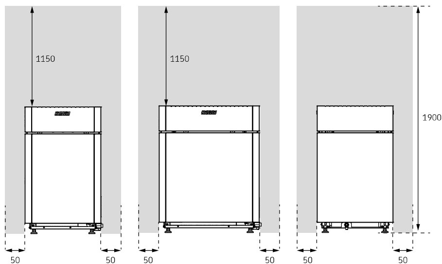
Obrázek 1 Bezpečnostní vzdálenosti
