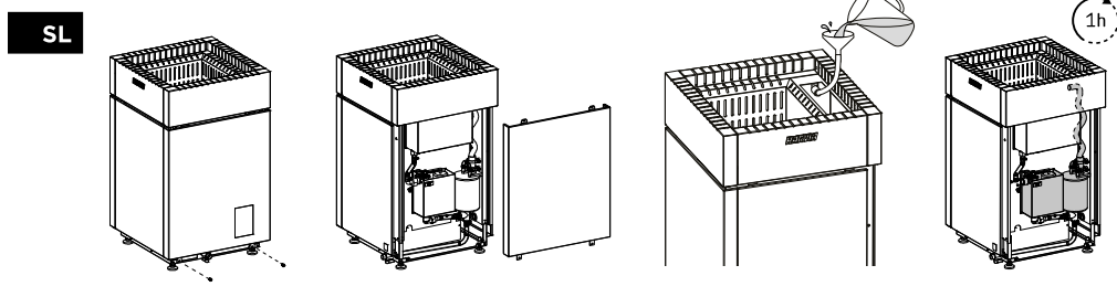
Slika 12. Odstranjevanje vodnega kamna z raztopino citronske kisline
