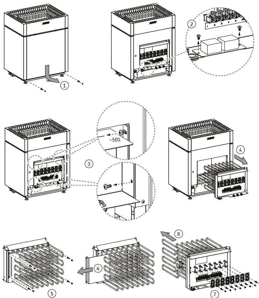
Figura 13. Sostituzione delle resistenze
