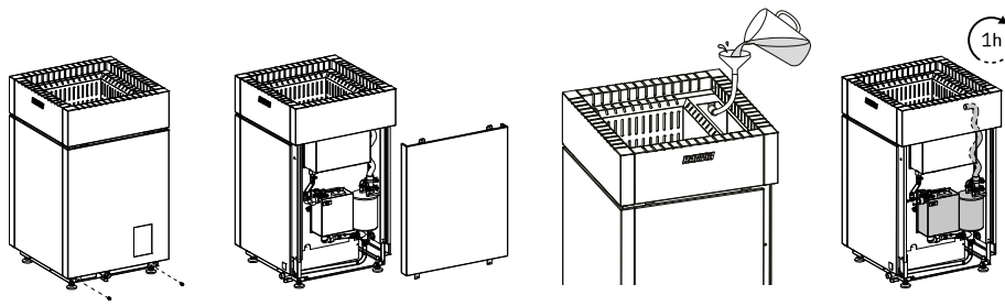
Kuva 12. Kalkinpoisto sitruunahappoliuoksella
