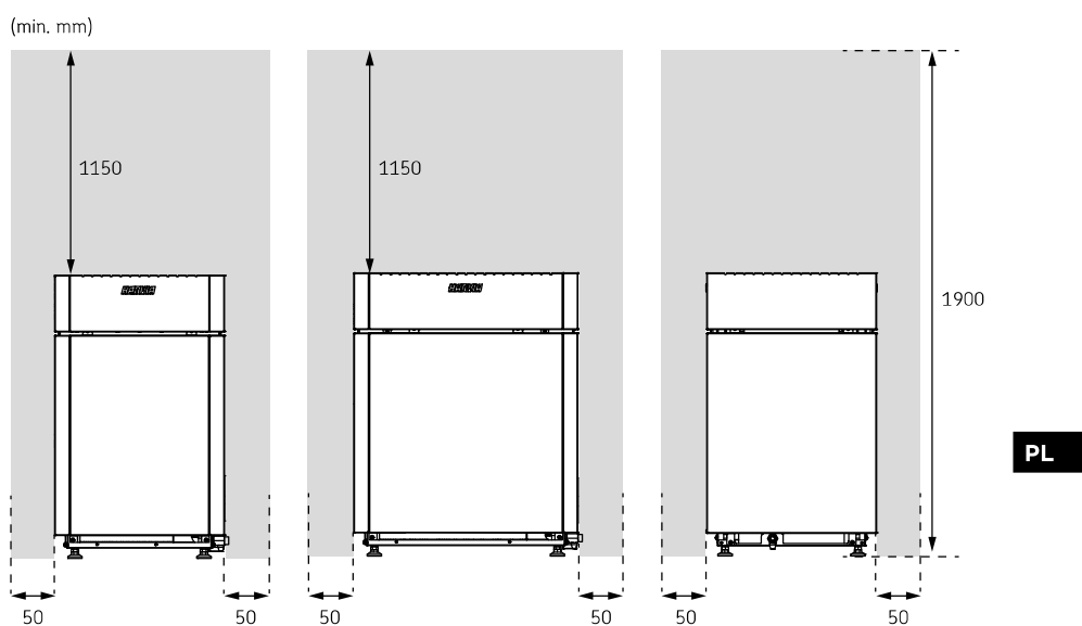
Rysunek 1. Odległości bezpieczeństwa
