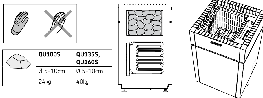
Figuur 8. Saunastenen plaatsen
