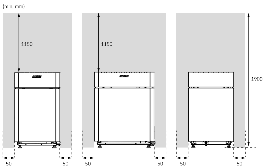
1 pav. Apsauginis atstumas
