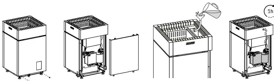
Bild 12. Avkalkning med en citronsyralösning
