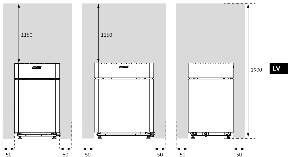
1. attēls. Droši attālumi
