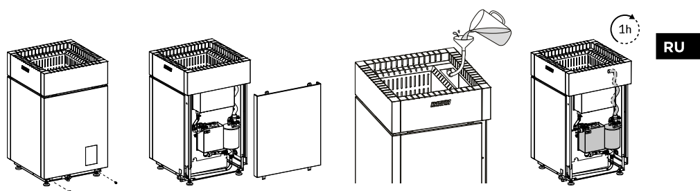
Рисунок 12. Удаление накипи раствором лимонной кислоты
