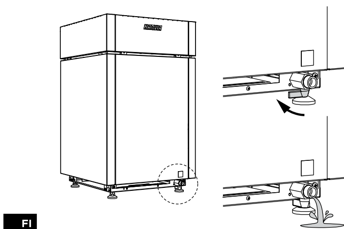
Kuva 11. Vesisäiliön tyhjentäminen
