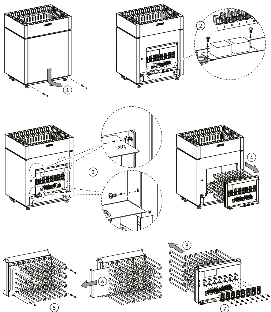
Abbildung 13. Auswechseln der Heizelemente
