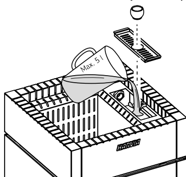
10 pav. Vandens bako pripildymas
