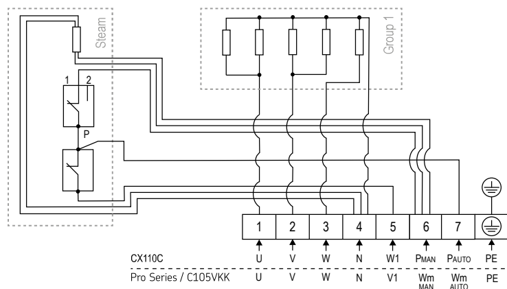
Bild 5. Kopplingsschema QU100S
