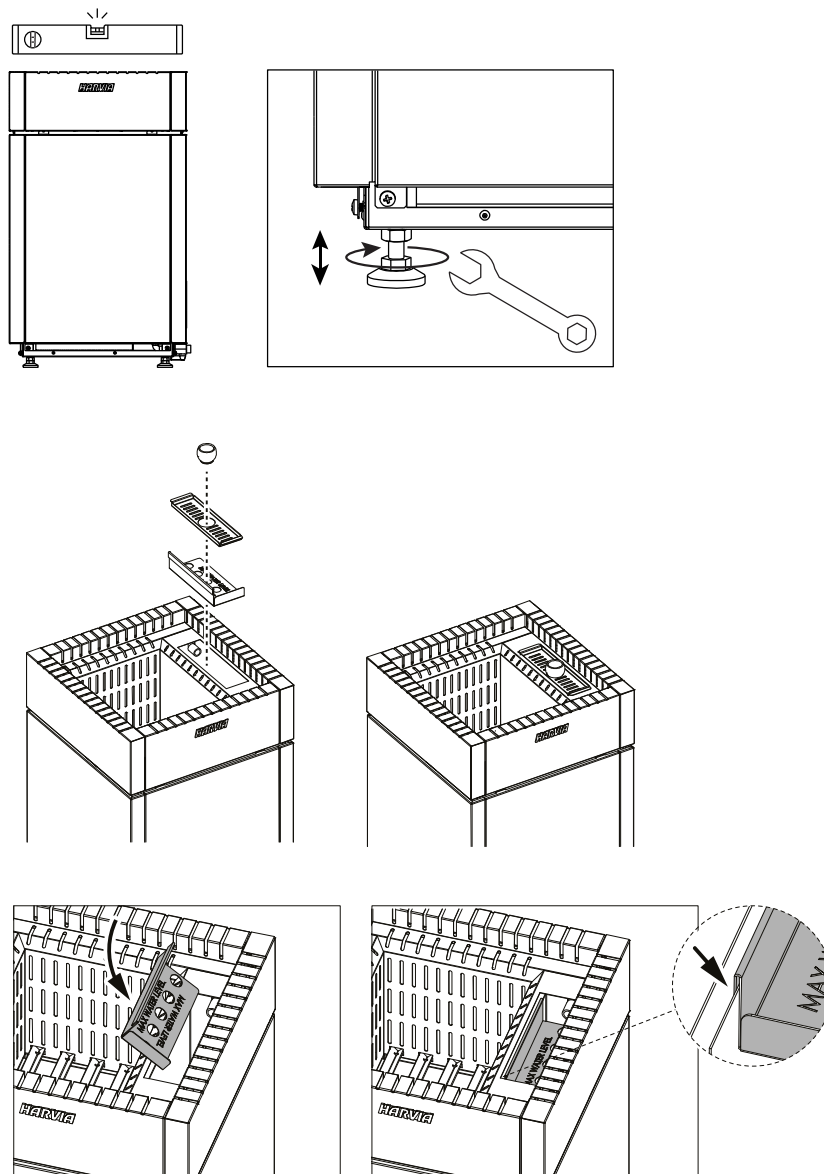
2 pav. Saunos krosnelės įrengimas
