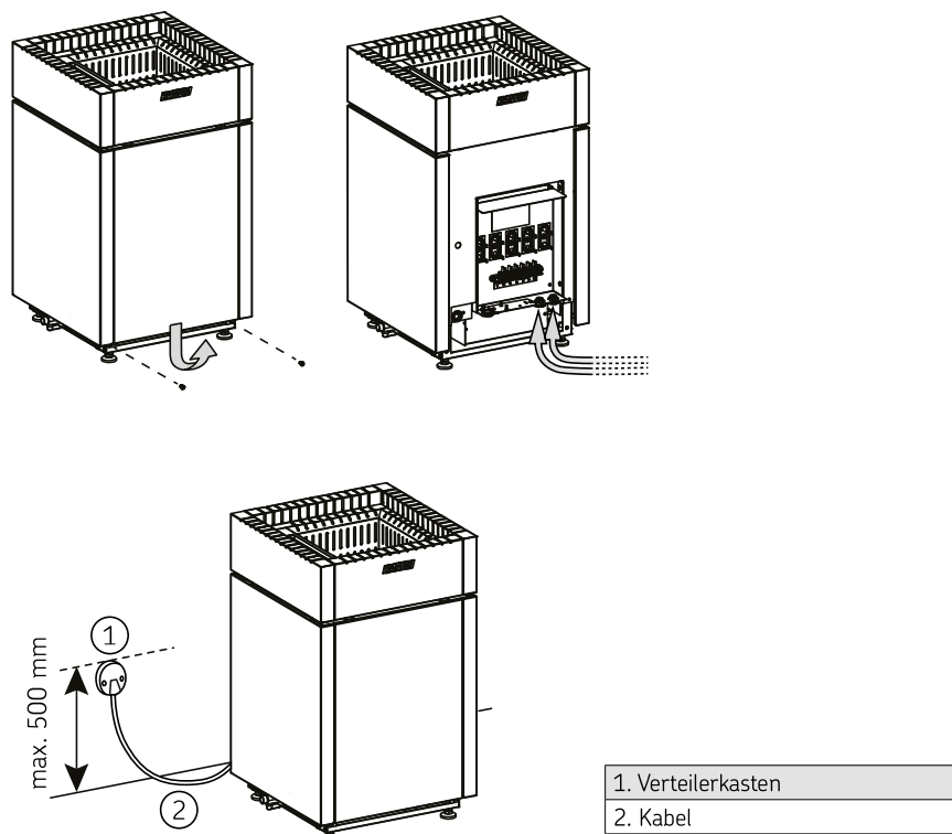
Abbildung 4. Elektroanschlüsse
