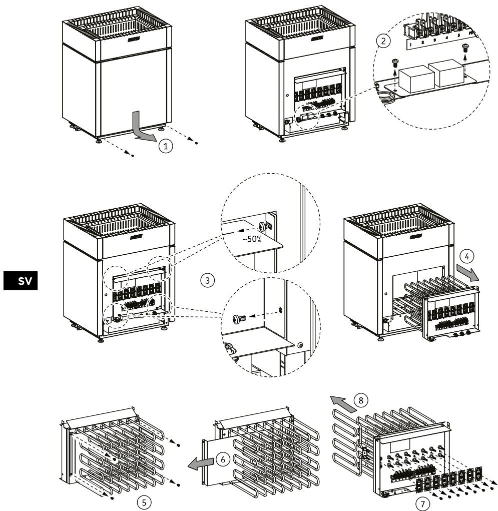
Bild 13. Byta värmeelement
