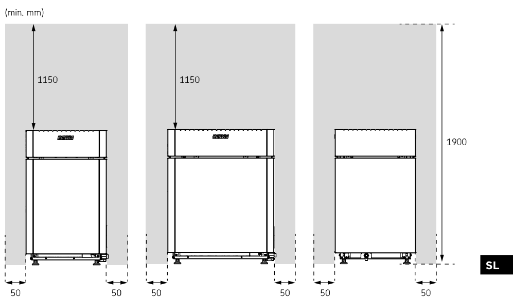
Slika 1. Varnostne razdalje
