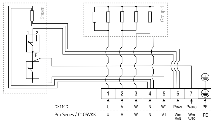
Abbildung 5. Stromlaufplan QU100S
