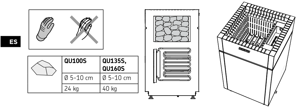
Figura 8. Colocación de las piedras de la sauna
