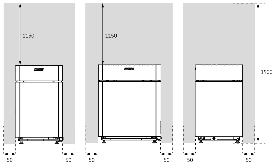
Kuva 1. Suojaetäisyydet
