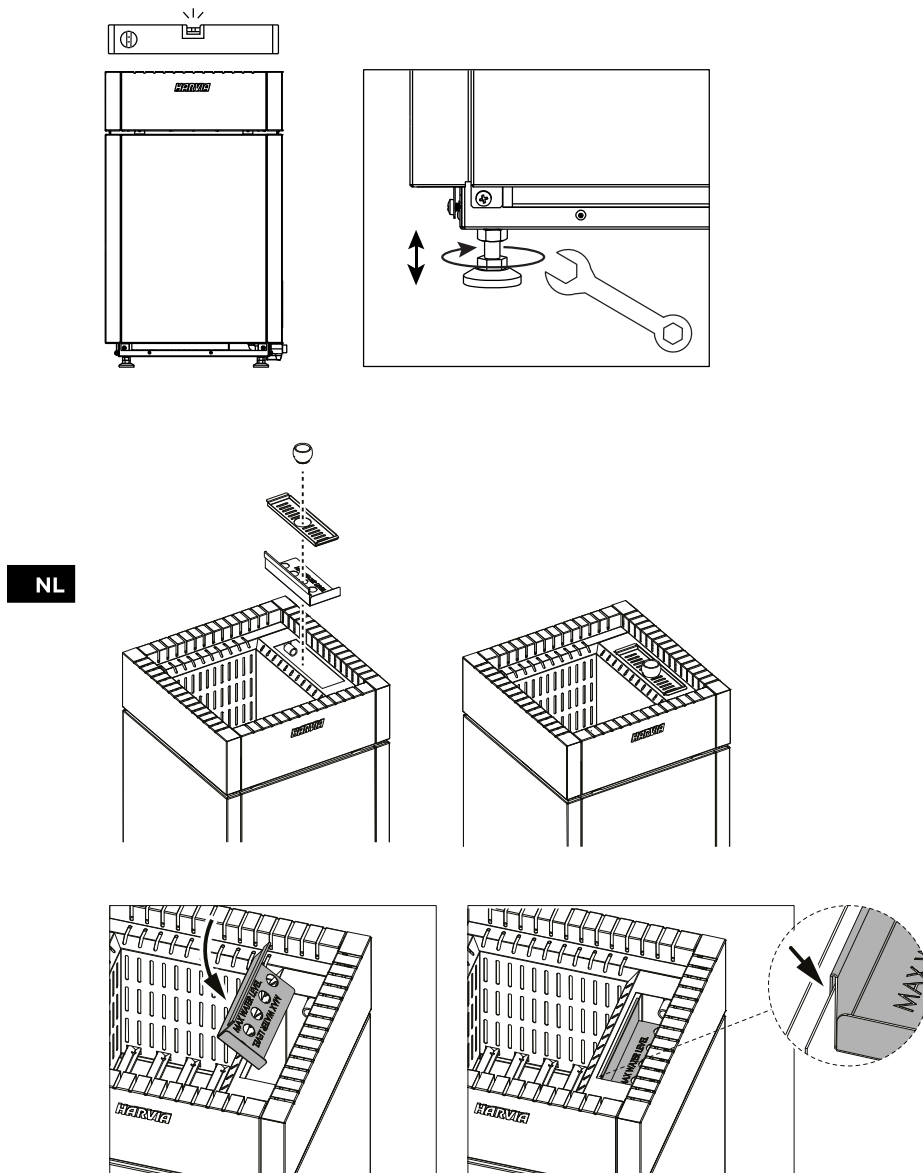
Figuur 2. Installatie saunakachel
