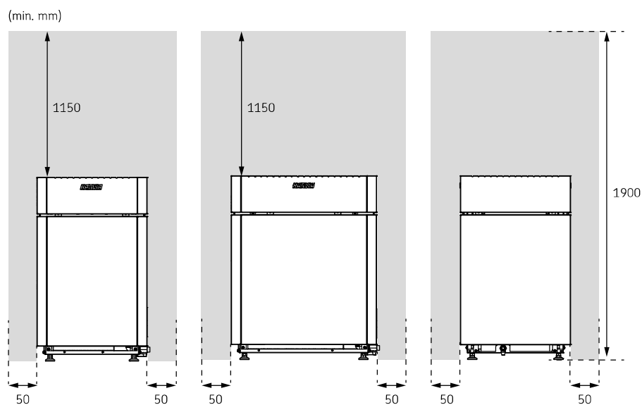
Abbildung 1. Sicherheitsabstände
