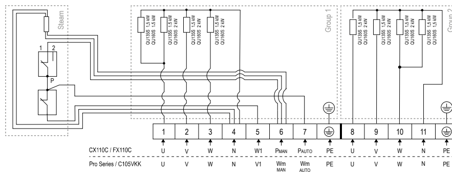
Abbildung 6. Stromlaufplan QU135S, QU160S
