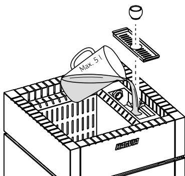
Joonis 10. Veepaagi täitmine
